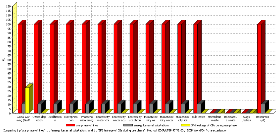
Fig. 3-14 : Comparaison des impacts environnementaux dans la phase d'utilisation de l'ensemble du système de transmission
