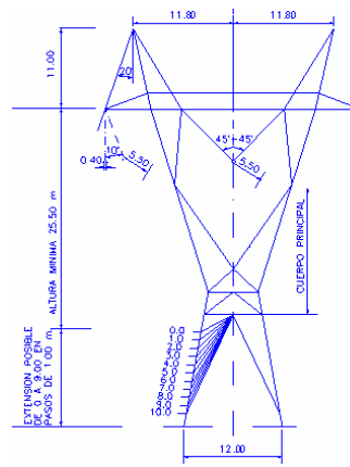
e) A/30 angle tension tower 27 ton
