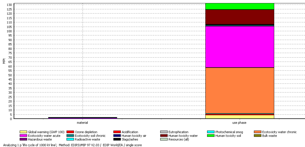
Fig. 4-4 : Résultat du score unique de la ligne de transmission chinoise à 1000 kV
