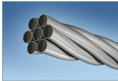
Fig. 3-5 : Alumoweld 7 #7 wire [58]
