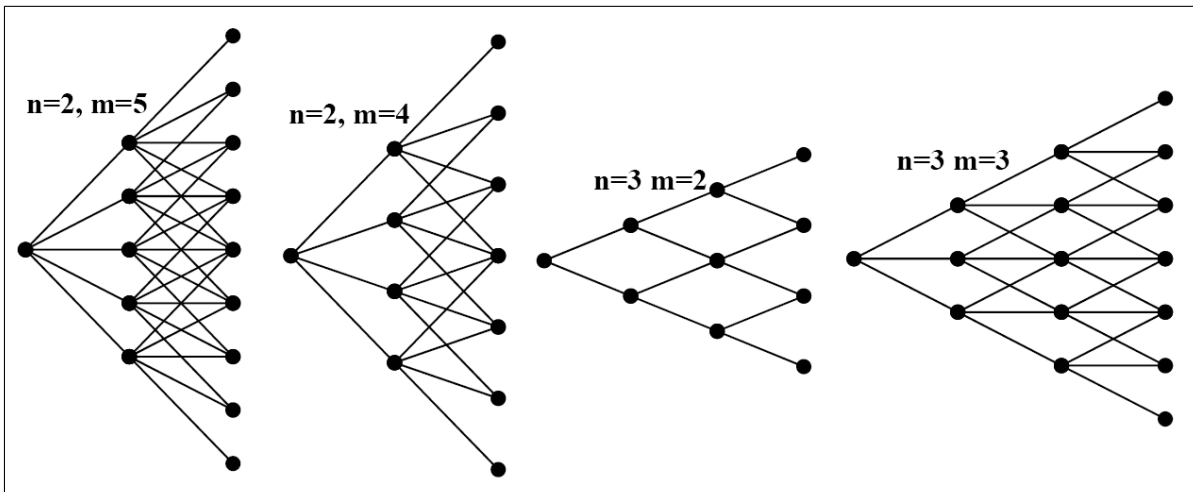
FIGURE 5.4 – Exemple d'arbres multinomiaux
