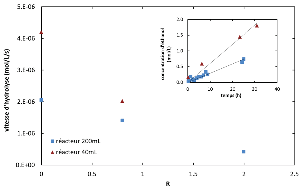
Figure 17 : Vitesse d'hydrolyse du TEOS en fonction du réacteur utilisé et de R, à 65°C et 250rpm. Insert : comparaison des cinétiques d'hydrolyse du TEOS à R=0 dans les deux réacteurs.
