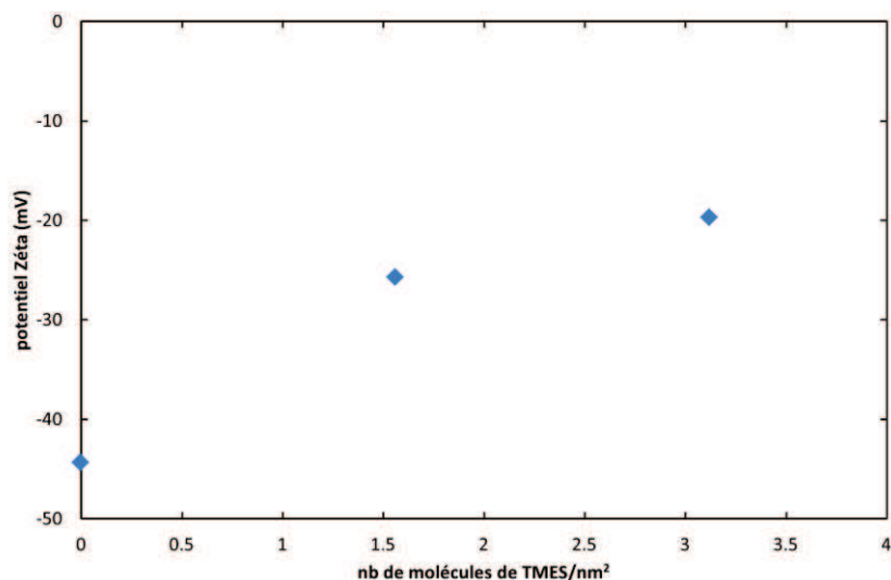
Figure 30 : Mesure du potentiel zêta des particules en fonction de la quantité de TMES utilisée pour le greffage.
