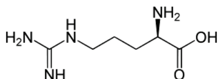
Figure 10 : Formule développée de l'arginine.
