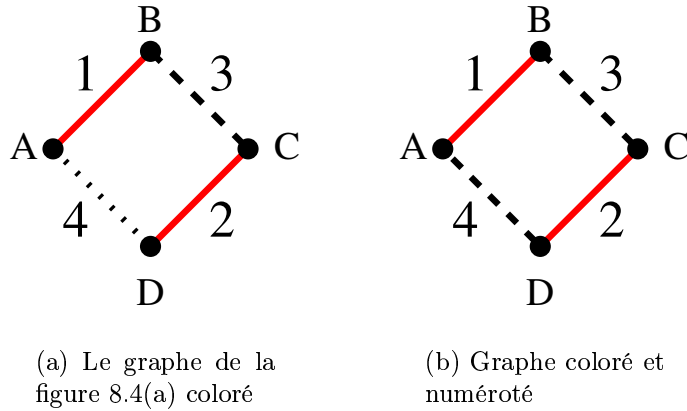
FIG. 8.5 – Colorations du graphe
