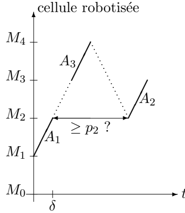
Figure 3.10: La séquence A_1A_3A_2
