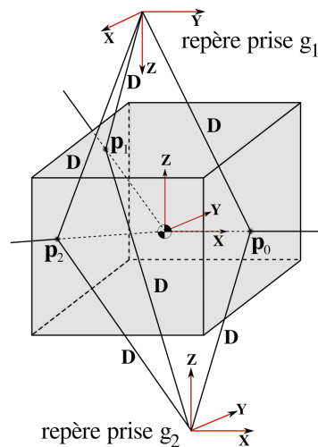
FIGURE 2.17 – Génération heuristique des prises à trois points de contact [Fischer 1997].
