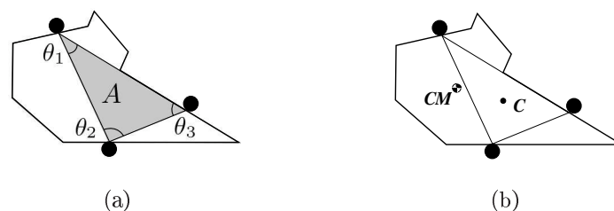
FIGURE 2.15 – Éléments utilisés dans les mesures basées sur les relations géométriques : (a) Angles internes et l'aire A du polygone de la prise. (b) Distance entre le barycentre du polygone et le centre de masse de l'objet.
