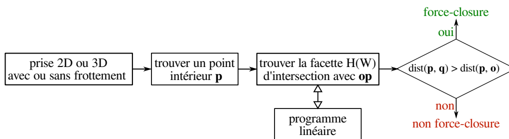
(a) Organigramme de l'algorithme de force-closure proposé par Liu [Liu 1999b].
