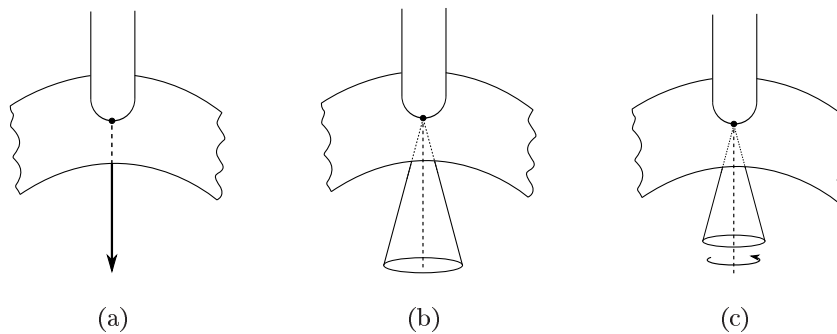
FIGURE 2.1 – Forces dans chaque type de contact : a) Ponctuel sans frottement. b) Ponctuel avec frottement ; c) Contact mou.
