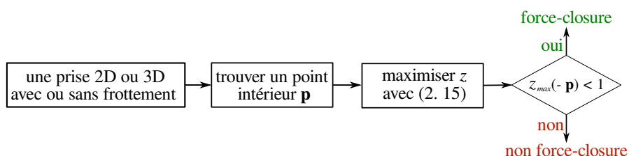
(b) Simplification proposée par Zheng et Qian [Zheng 2005].
