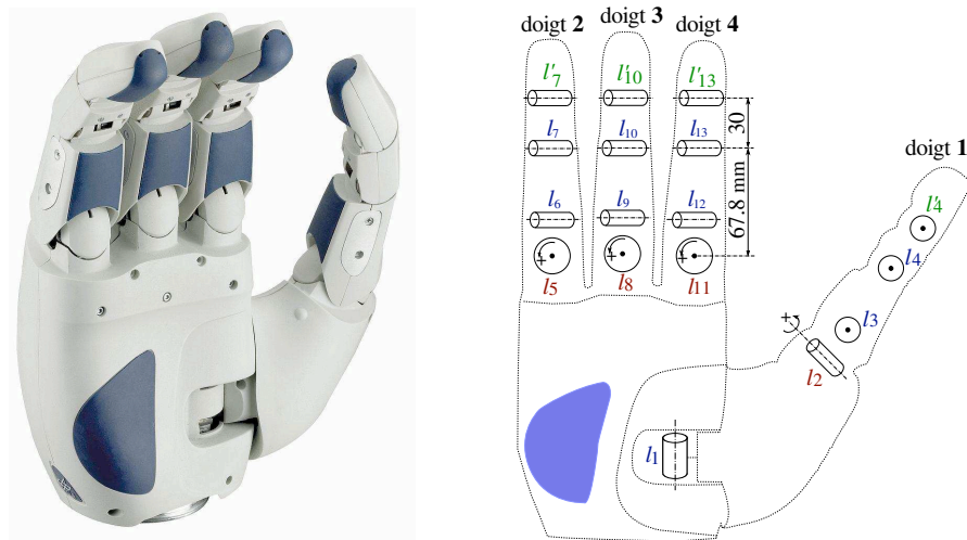
FIGURE 5.13 – Architecture cinématique de la main SAH.
