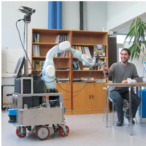
FIGURE 1.1 – Le manipulateur mobile Jido apportant une bouteille (LAAS).
