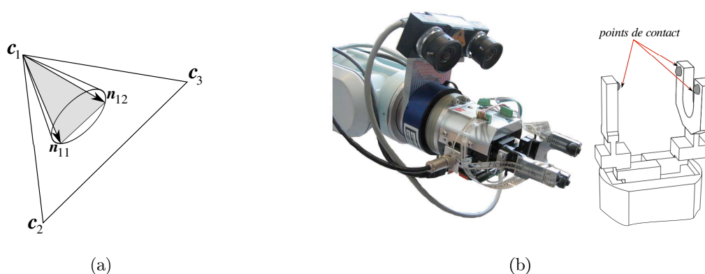
FIGURE 2.14 – (a) Intersection du cône de frottement avec le plan de contact. (b) Pince parallèle à trois points de contact.
