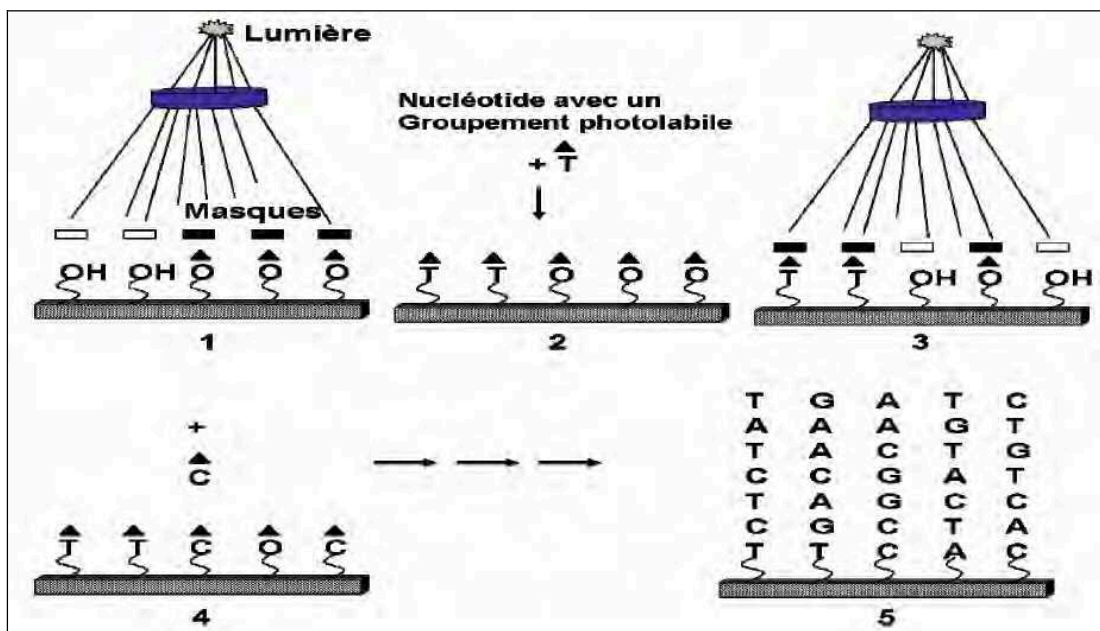
Figure 33 : Schéma de synthèse in situ des oligonucléotides par un procédé de photolithographie utilisé par Affymetrix.
