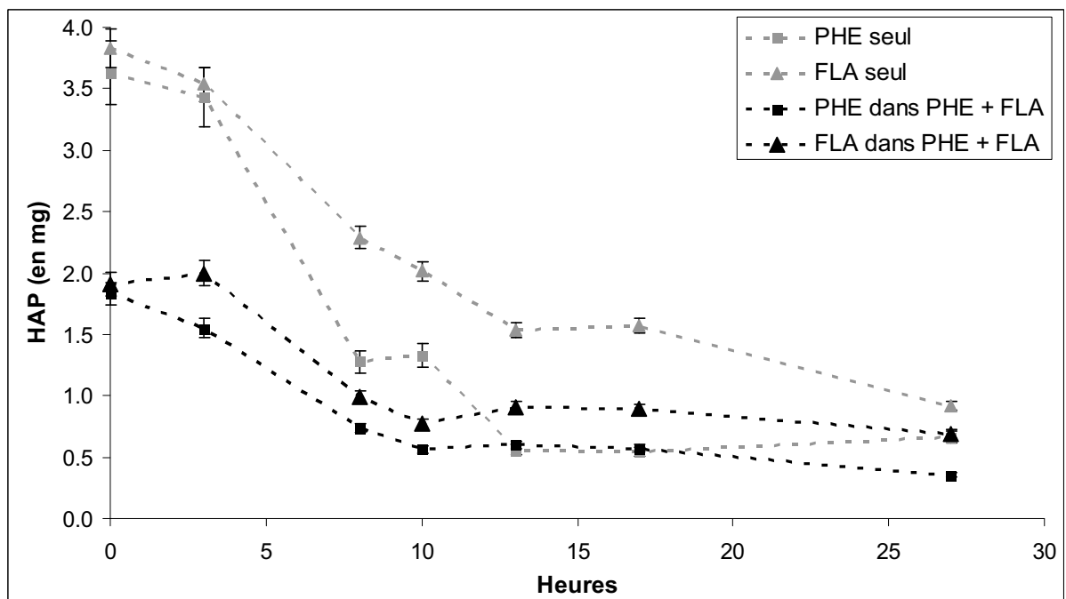
Figure 47 : Suivis de dégradation des HAP par CLHP, durant la croissance de la souche Sphingomonas paucimobilis sp. EPA505.
