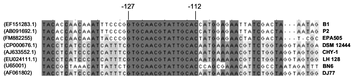
Figure 58 : Caractérisation de séquences régulatrices par alignement multiple des régions intergéniques des gènes xyfX et bphC de plusieurs espèces bactériennes.
