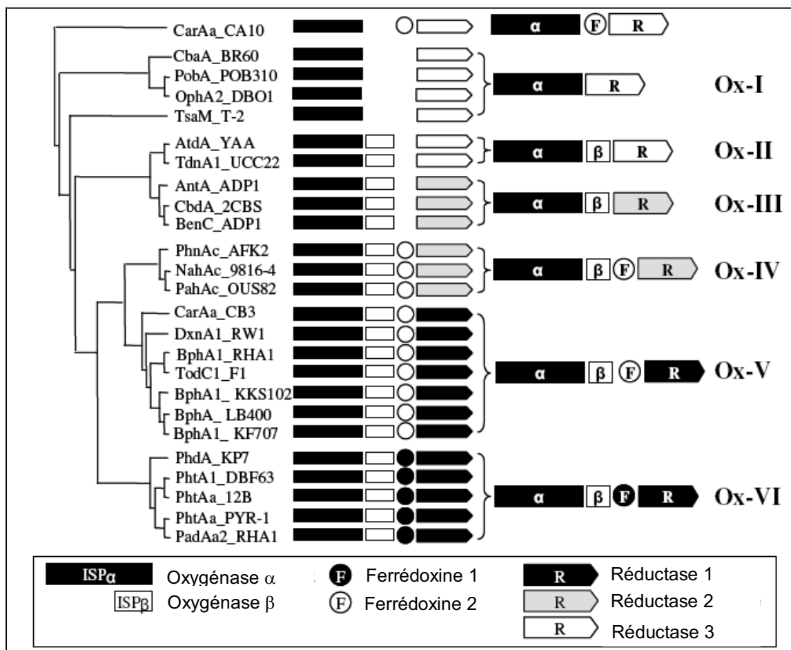
Figure 11 : Représentation graphique de l'organisation en plusieurs classes oxydatives (de I à VI) des dioxygénases. (Proposé par Kweon et al. , 2008).
