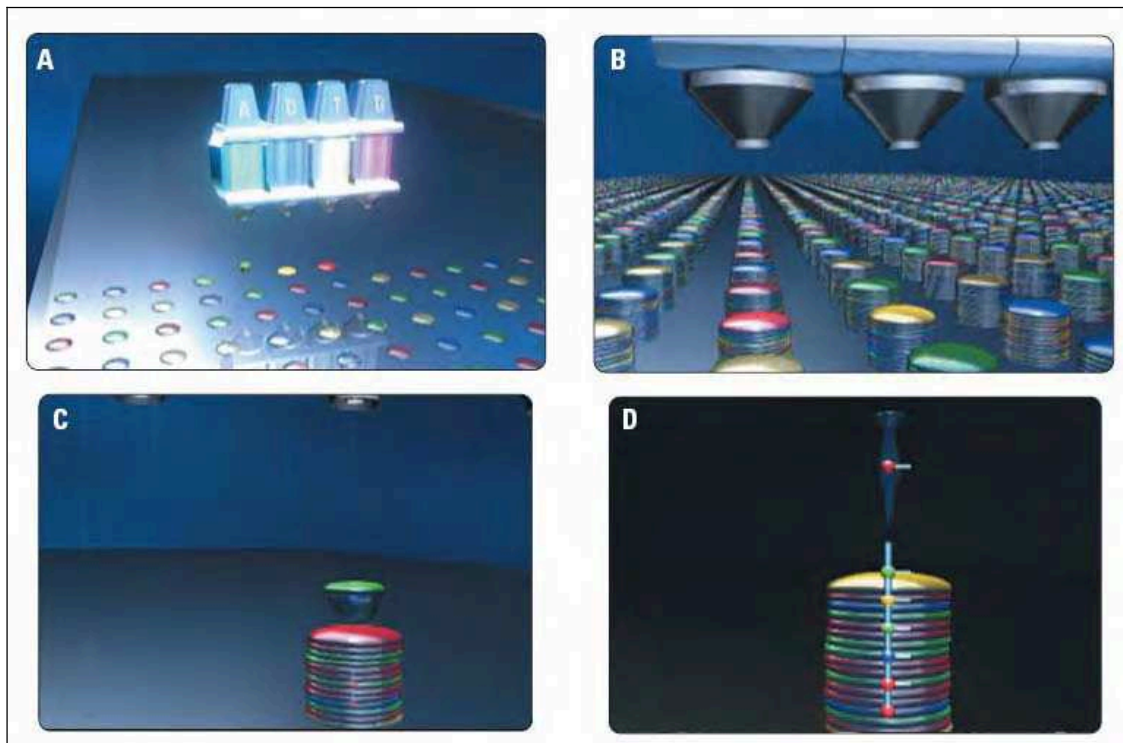
Figure 32 : Représentation schématique de la technologie de fabrication in situ des biopuces ADN Agilent.
