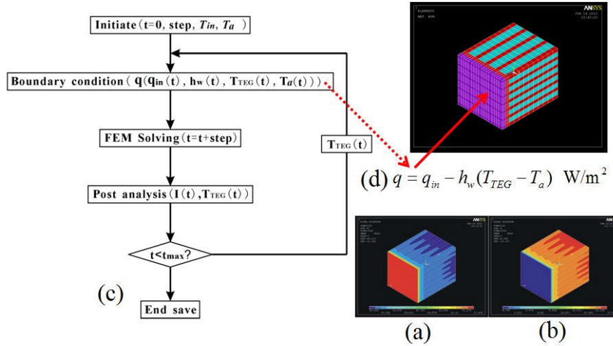
Figure (a9) : Modèle éléments finis et exemple de distribution de la température dans un élément de base (1TEG+MCP) (a) durant le jour (b) pendant la nuit, (c) et (d) organigramme de l'analyse transitoire
