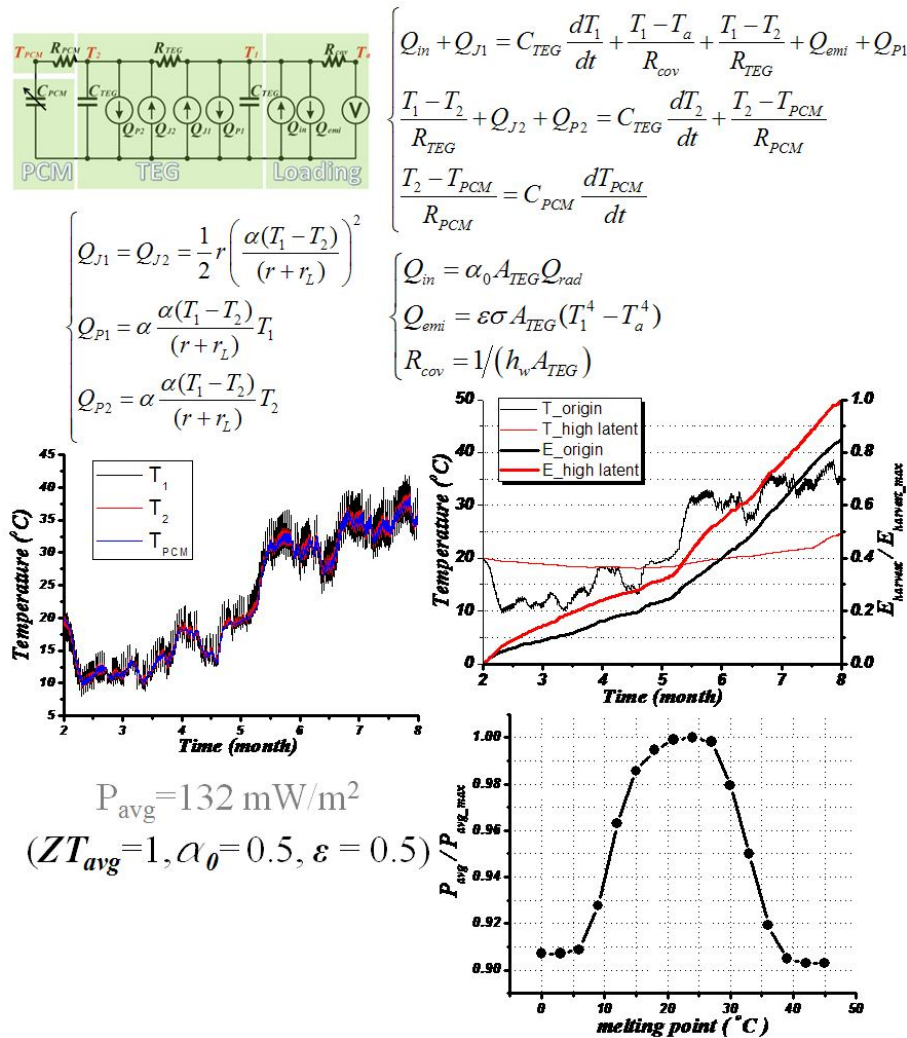
Figure (a10) : Modèle simplifié et résultats de simulation sur 6 mois
