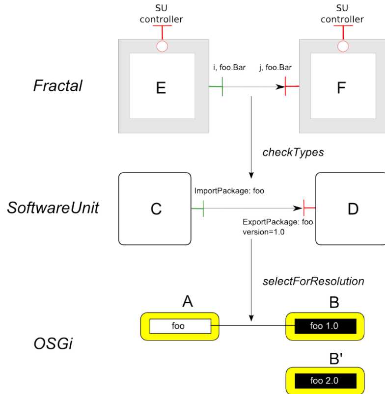
FIGURE 5.5 – Cohérence des liaisons entre composants définis avec des bundles OSGi
