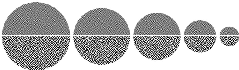
FIGURE D.11: Zoom sur une sphère texturée avec notre bruit de Gabor NPR avant (haut) et après seuillage binaire (bas). À chaque niveau de zoom, les propriétés statistiques du bruit sont bien préservées grâce à notre mécanisme de niveau de détail.
