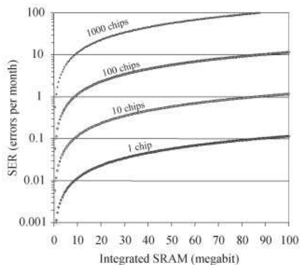
Figure 1.4 : Exemples de données de SER au cours d'un mois en fonction du nombre de puces et du nombre de mémoires SRAM par puce.
