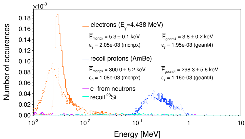
FIGURE 4.18 – Distribution d'énergie déposée (normalisée) calculée par MCNPX (en traits continus) et GEANT4 (en traits pointillés) pour notre source AmBe. Le rapport n_{\gamma}/n_{\text{neutrons}} a été pris en compte. Les spectres sont normalisés [VHH + 11].
