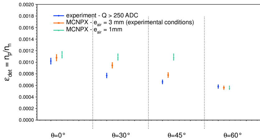
FIGURE 4.39 – Comparaison des efficacités de détection expérimentale et simulées du capteur pour différents angles d’incidence et différentes épaisseurs d’air.
