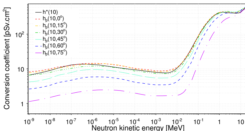
FIGURE 1.20 – Facteurs de conversion flux-dose en fonction de l'énergie des neutrons et pour différents angles [ICR96].
