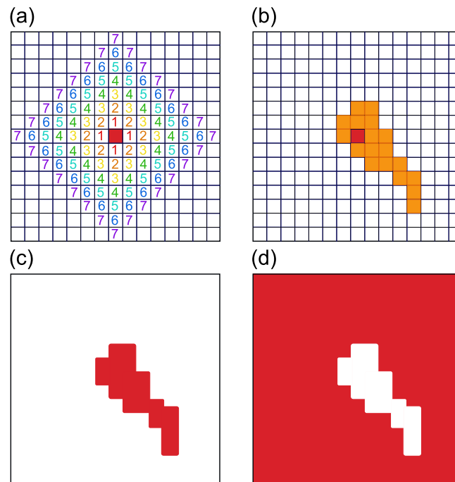
FIGURE 2.42 – Schéma de l'algorithme de « clusterisation ».
