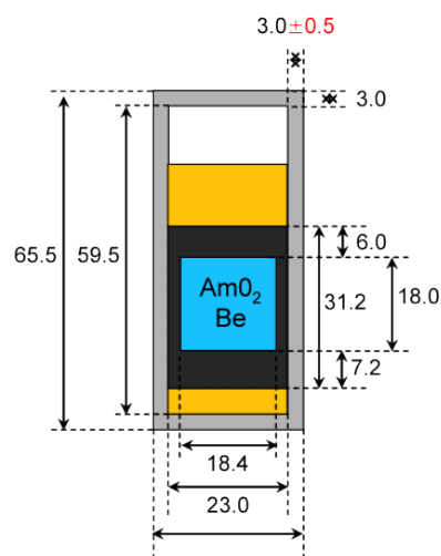
FIGURE 2.28 – Dimensions de la source ^{241}\text{AmBe} [Tro10]. Les cotes sont données en mm.
