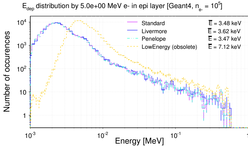
FIGURE 3.6 – Distribution de l'énergie déposée par des électrons de 5 MeV dans la couche épitaxiale du capteur obtenue avec GEANT4 .
