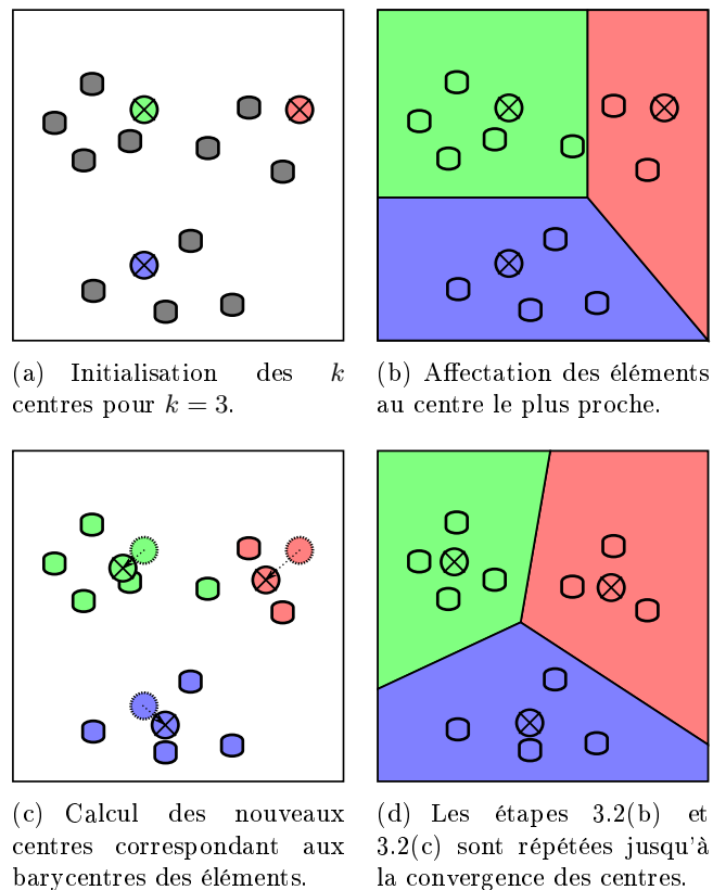
FIG. 3.2 – Algorithme du k -means.
