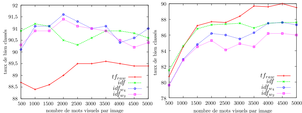
FIG. 3.6 – Résultats comparant les différentes pondérations utilisant la fréquence documentaire pour des vocabulaires de 5000 mots basés sur le descripteur mstd (à gauche) et sift (à droite).
