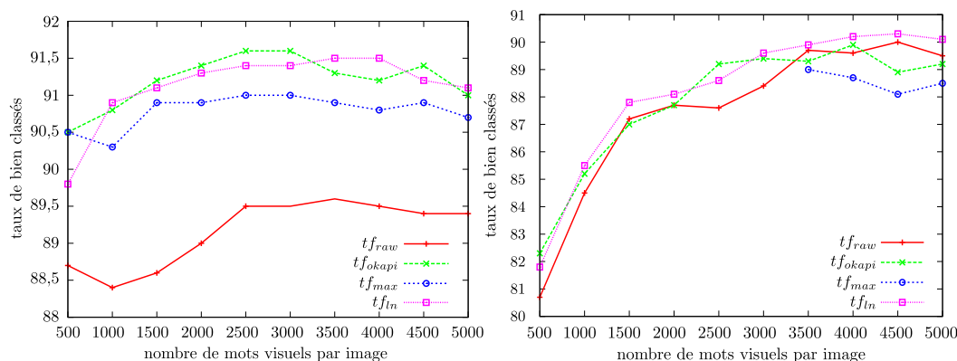
FIG. 3.5 – Résultats comparant les différentes pondérations utilisant la fréquence des termes pour des vocabulaires de 5000 mots basés sur le descripteur mstd (à gauche) et sift (à droite).
