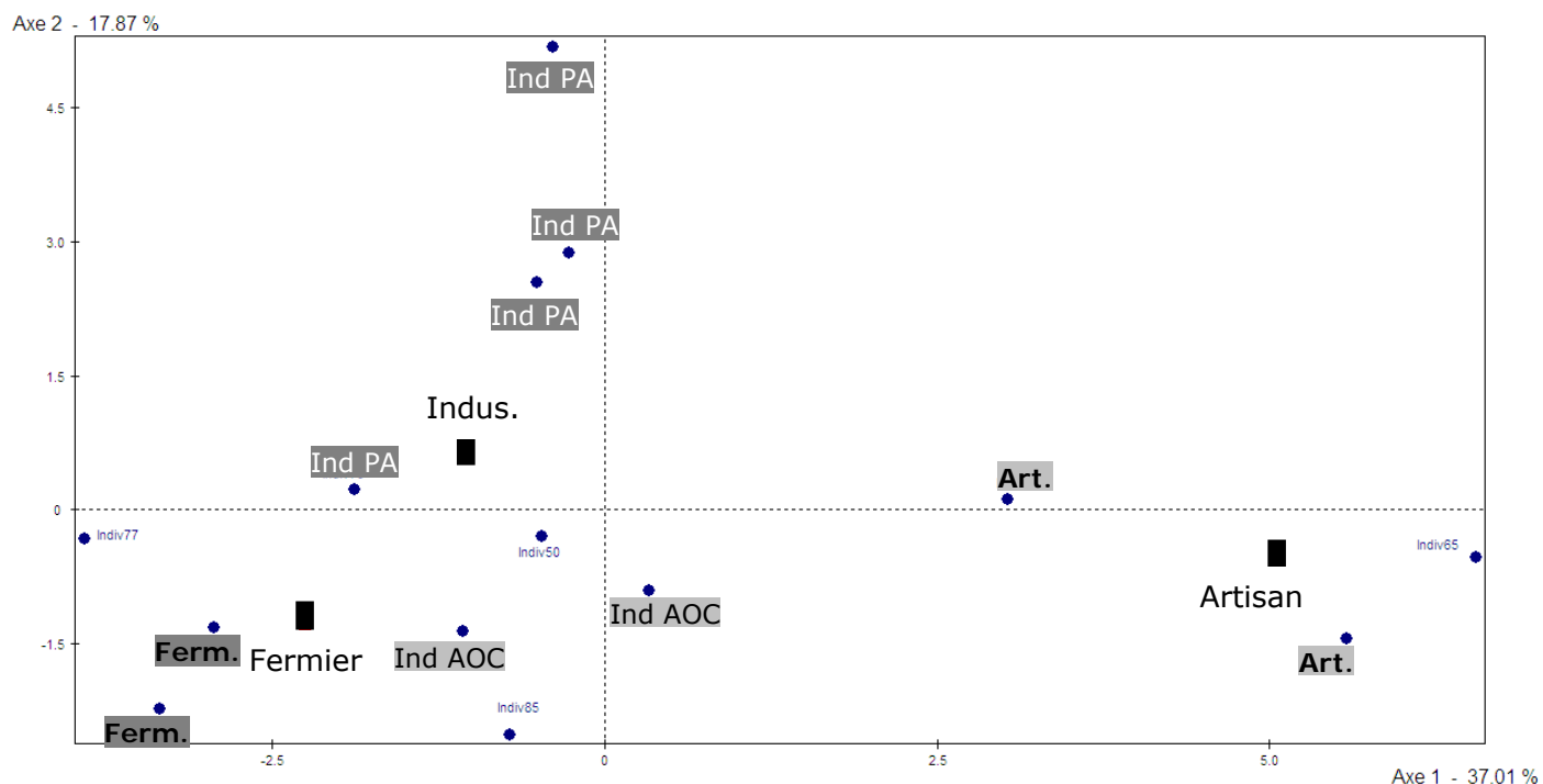
Figure 23 : ACP réalisée sur les aires relatives de 24 composés volatils pour les échantillons (individus) prélevés lors de la dernière phase de la fermentation alcoolique l'année 2
