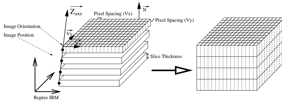
FIG. 3.3 – La reconstruction des IRM doit se faire avec précaution. Les coupes ne sont pas obligatoirement jointives, et rien ne garantit que l’axe de progression de l’origine du repère 2D – \vec{Z}_{axe} – soit perpendiculaire au plan de coupe. Dans tous les cas, les voxels issus de l’acquisition coupe à coupe (à gauche) ne seront pas automatiquement les mêmes que ceux de l’image finale qui sera traitée par le système (à droite).
