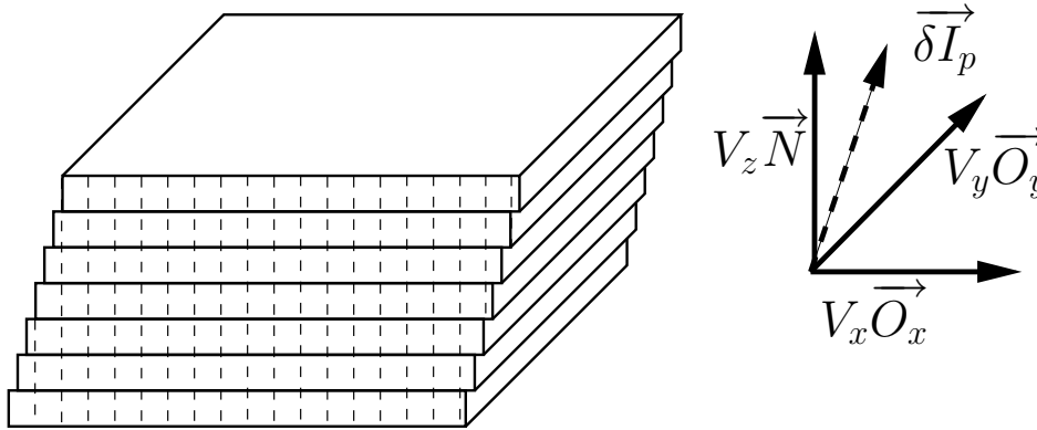
FIG. 9.1 – La reconstruction correcte des images IRM issues des données DICOM nécessite un rééchantillonnage : dans le cas général, \vec{\delta I}_p , le vecteur de progression de l'origine du repère 2D de chaque coupe I_p , n'est pas colinéaire à la normale au plan de coupe \vec{N} .
