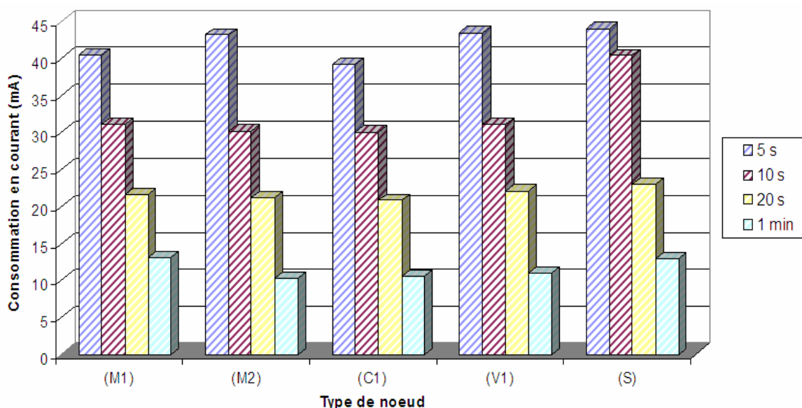
Figure 67 : Impact de la périodicité sur les performances des nœuds dans le réseau.
