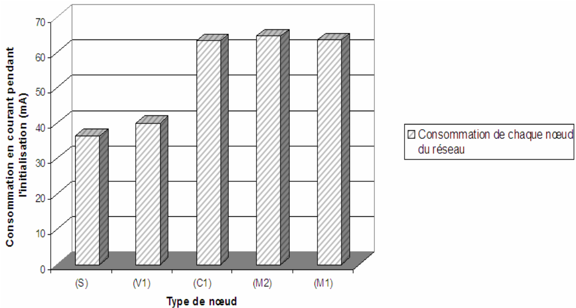
Figure 64 : Consommation de chaque nœud du réseau pendant la phase d'initialisation.
