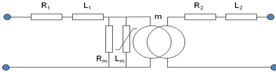
FIG. 2.3a Modélisation d'un transformateur monophasé en basse fréquence avec saturation
