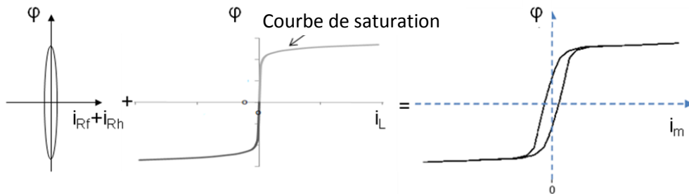
FIG. 2.9d. Calcul d'un cycle d'hystérésis réel
