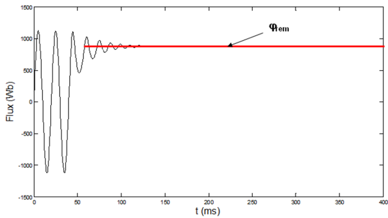
FIG. 3.4a Flux sur une phase d'un transformateur mis hors tension à C_p = 10nF
