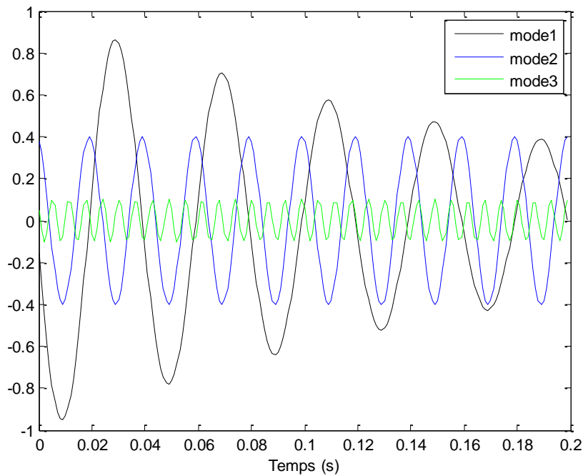
FIG. 3.7b Composantes modales estimées par MP, f_l=25
