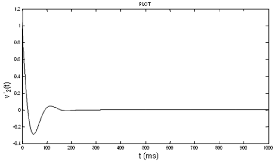
FIG.5.2a. Réponse indicielle du TCT
