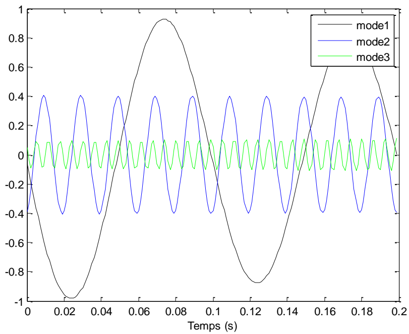
FIG. 3.8b Composantes modales estimées par MP, f_I=10
