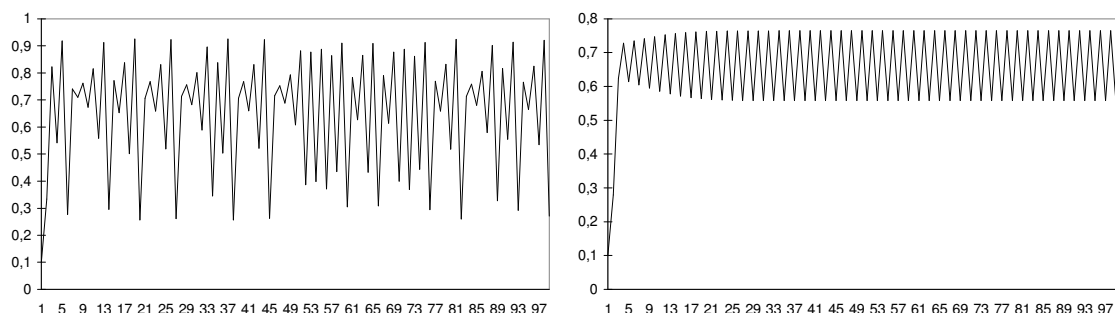
Graphique 2 : Exemples de simulation pour A=3,7 et A=3,1 ( K_0=0,1 )
