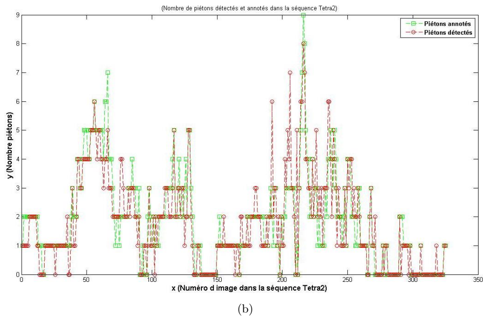
Figure 5.7. Comparaison entre les résultats obtenus et les données expérimentales de référence. Les courbes comparent, pour les deux séquences, le nombre de piétons réels et le nombre de piétons correctement détectés.
