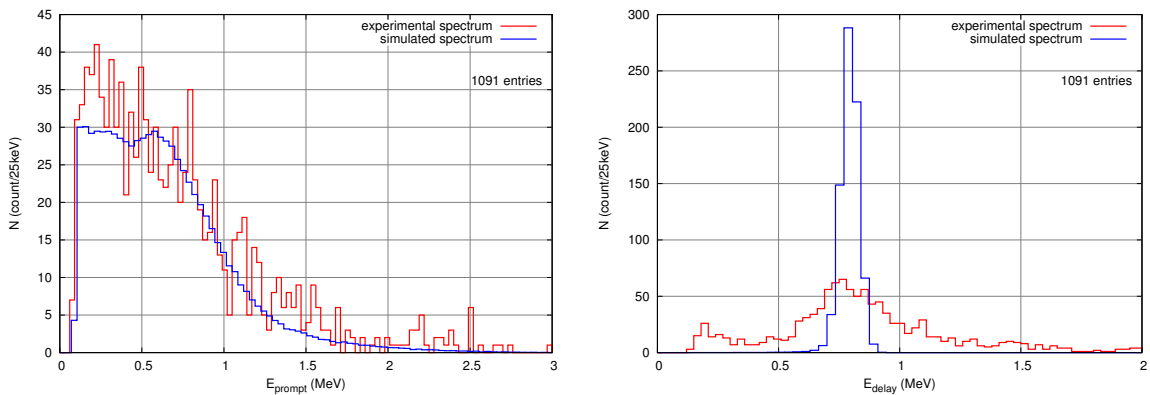
FIG. 9.29: Spectres en énergie des évènements \beta et \alpha retardé du 214 Bi des modules dédiés à la mesure de contamination de surface ; en rouge : données réelles ; en bleu : données simulées
