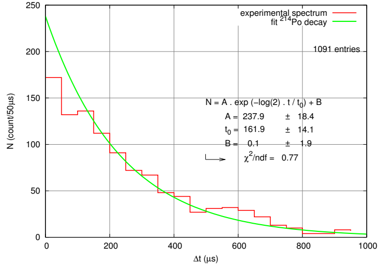
FIG. 9.28: Décroissance du 214 Po - évènements back-to-back des modules dédiés à la mesure de contamination de surface ; en rouge : données réelles ; en vert : ajustement exponentiel
