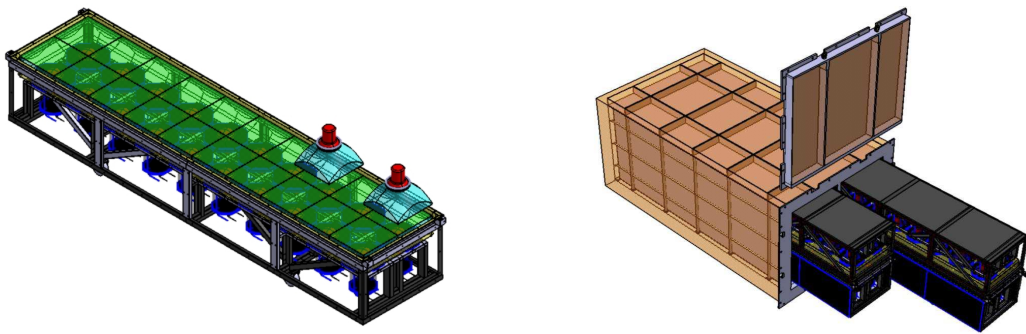
FIG. 9.34: Vue générale du détecteur BiPo3 ; à gauche : schéma d'un module en cours d'assemblage ; à droite : détecteur complet et blindage
