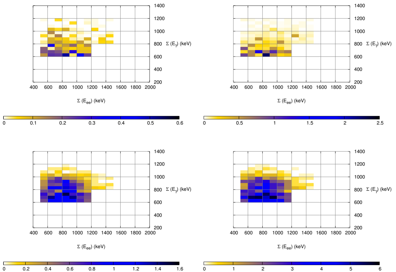
FIG. 6.10: Distribution des évènements simulés de bruit de fond (en haut) et de signal recherché (en bas) en fonction des énergies des électrons et des \gamma ; à gauche : phase 1 ; à droite : phase 2
