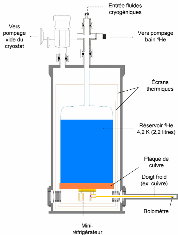
Figure 6.1 : Représentation du cryostat complété d'un doigt froid de mesure
