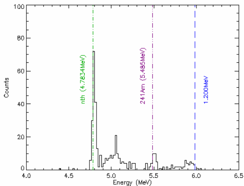
Figure 4.26 : Spectre en énergie à 1200 keV avec cône d'ombre (durée effective = 560 s).
