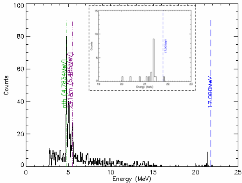
Figure 4.31 : Spectre en énergie à 17 MeV (polarisation basse) sans cône d'ombre (en encadré, zoom sur la raie à 17 MeV) (durée effective = 1160 s).
