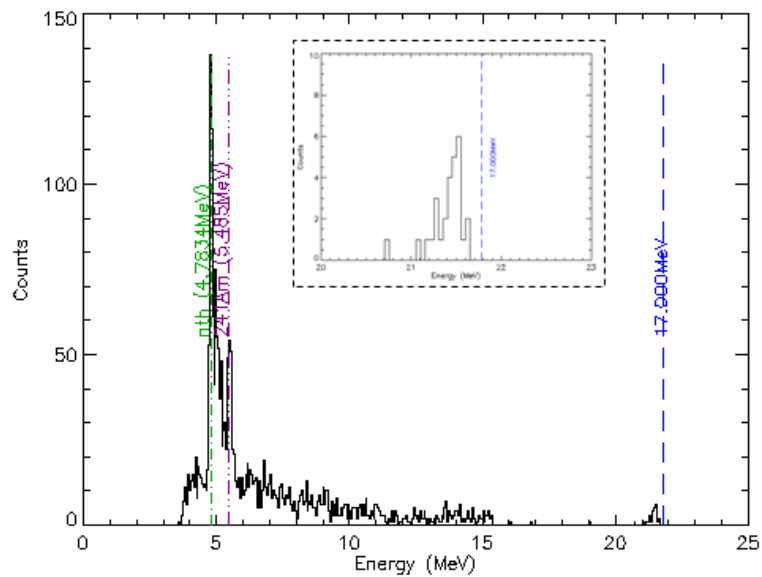
Figure 4.35 : Spectre en énergie à 17 MeV (polarisation haute) sans cône d'ombre (en encadré, zoom sur la raie à 17 MeV) (durée effective = 2725 s).
