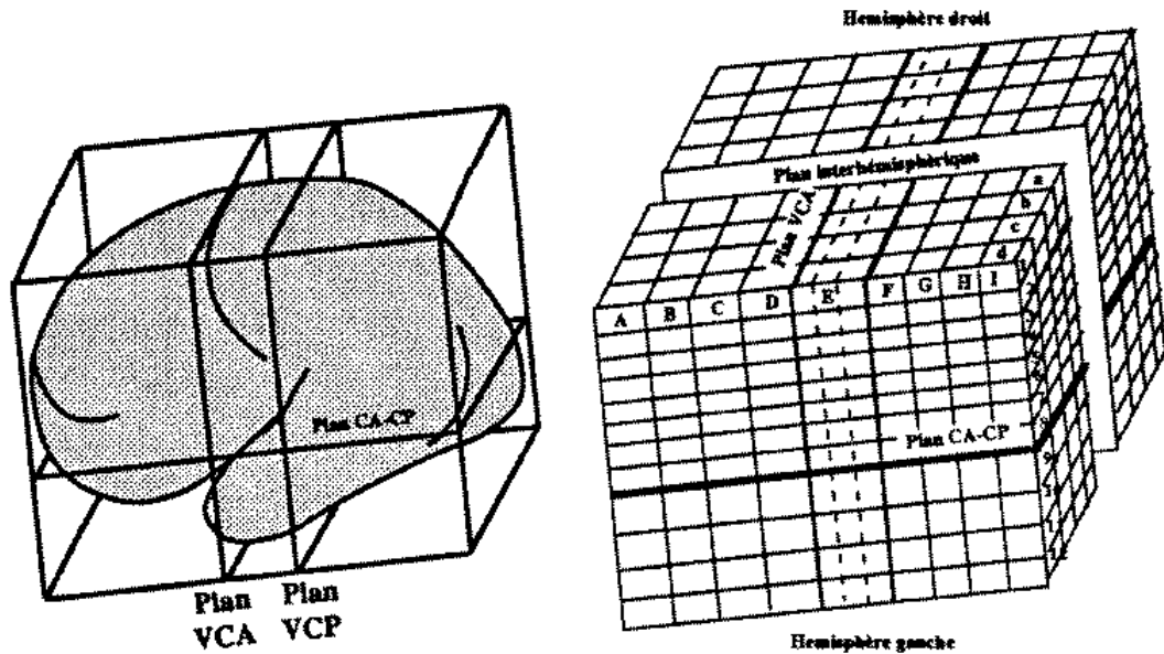
FIG. 3.6 – Le système de grille proportionnelle tridimensionnelle de Talairach [Talairach and Tournoux, 1988]. Chaque structure cérébrale a des coordonnées dans l'espace 3D, ce qui permet de la comparer directement aux structures correspondantes identifiées à la même position chez d'autres sujets.
