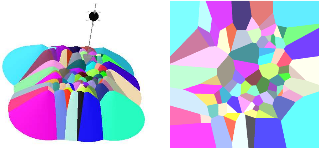
FIG. 5.32 – Calcul rapide de diagrammes de Voronoï 2D en utilisant la carte graphique de l'ordinateur: des cônes sont placés au dessous de chaque graine et une vue de dessus de cette scène tridimensionnelle obtenue par la technique du z-buffer permet d'obtenir directement le diagramme de Voronoï associé à ces graines.
