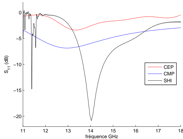
FIGURE 4 – Perte d'adaptation simulé avec une dipôle placée près d'un plan de masse de trois types
