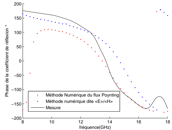
FIGURE 20 – Comparaison des résultats numériques avec la mesure (Polarisation verticale, échantillon avec une fente à côté du carré métal)
