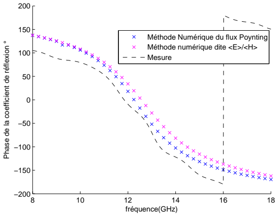
FIGURE 17 – Comparaison des résultats numériques avec la mesure (Polarisation verticale, échantillon rectangulaire : D_x = 4 mm, D_y = 6 mm, W = 7 mm, L = 9 mm, h = 1.6 mm, \epsilon_r = 4.2 .)
