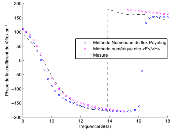
FIGURE 18 – Comparaison des résultats numériques avec la mesure (Polarisation horizontale, échantillon rectangulaire : D_x = 4 mm, D_y = 6 mm, W = 7 mm, L = 9 mm, h = 1.6 mm, \epsilon_r = 4.2 .)
