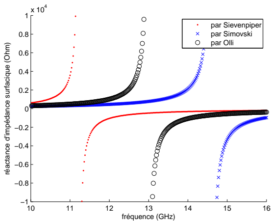
FIGURE 10 – Comparaison d'impédance surfacique des différents méthodes analytiques avec la structure en champignon ( D = 10\text{mm} , g = 5\text{mm} , h = 2\text{mm} , \varepsilon_r = 4.4 )
