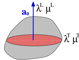
FIG. 2.15 – Définition de coefficients de Lamé dans la direction privilégiée et dans le plan transverse
