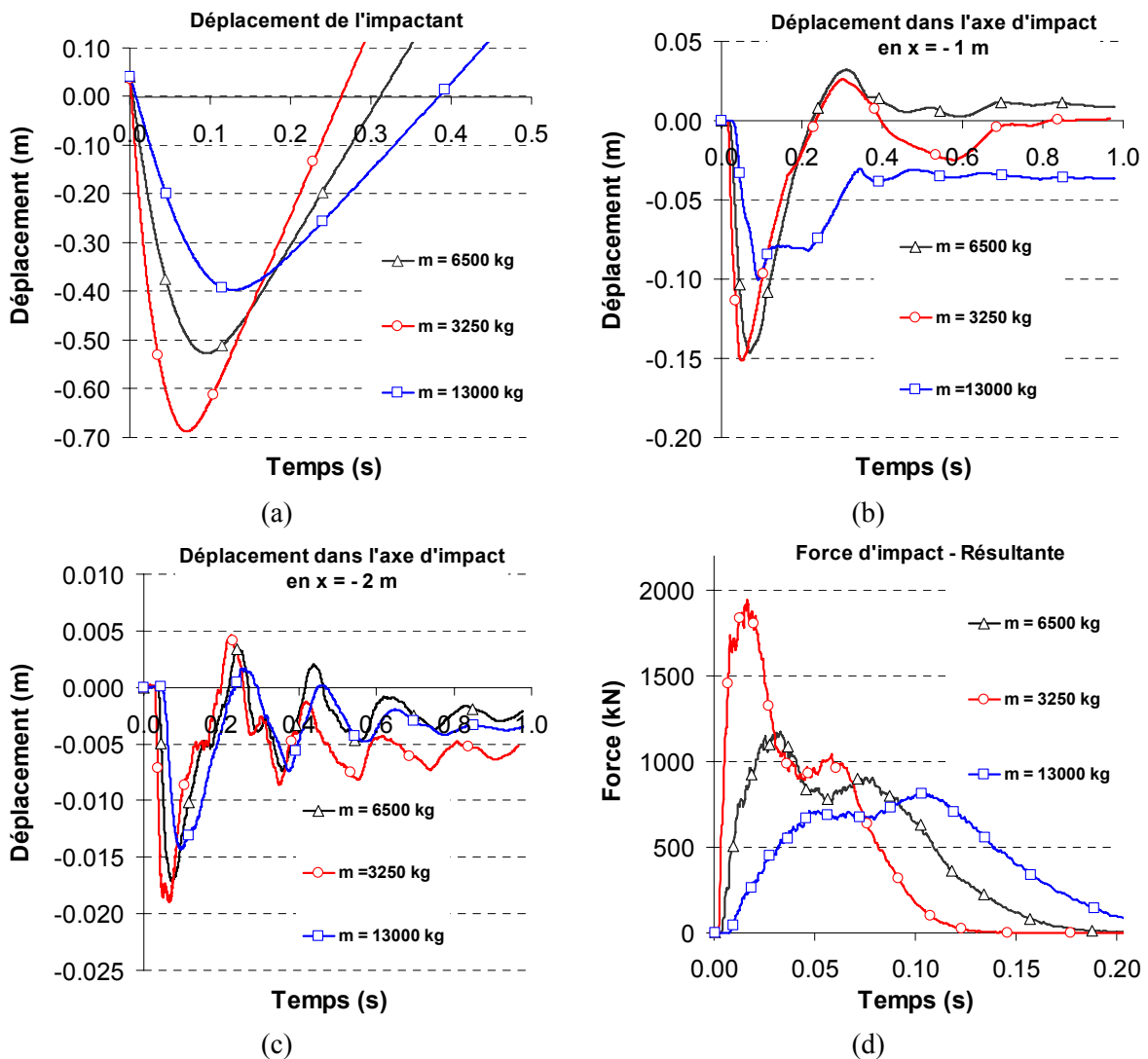
Figure 4-52 : Effet de la taille de l'impactant, à quantité de mouvement initiale constante ( p_I = 84\,000 \text{ kg.m.s}^{-1} ), sur le calcul du déplacement horizontal de l'impactant (a), à l'interface parement-noyau (b), à l'interface noyau-remblai (c), et de la force d'impact (d).
