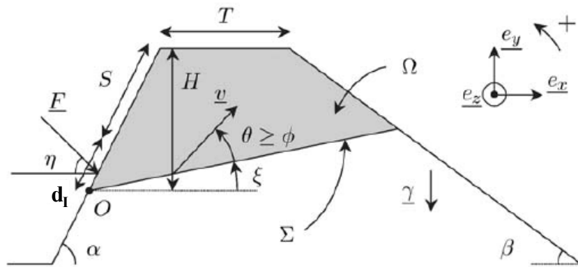
Figure 1-3 : Modèle géométrique et surface de rupture supposés par Subrin [Subrin 2006].
