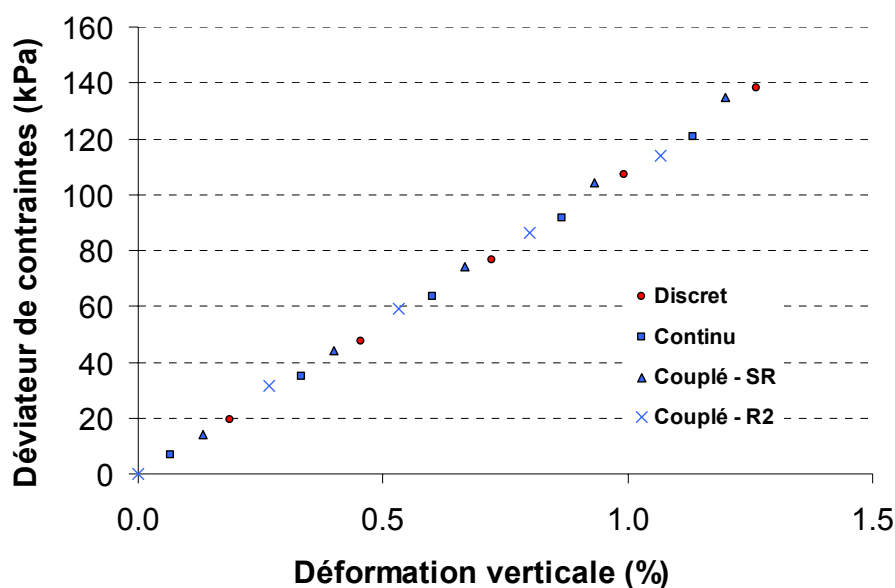
Figure 3-15 : Caractérisation du module d'Young : Evolution des contraintes verticales avec la déformée pour les modèles couplés et comparaison avec les approches discrète et continue.
