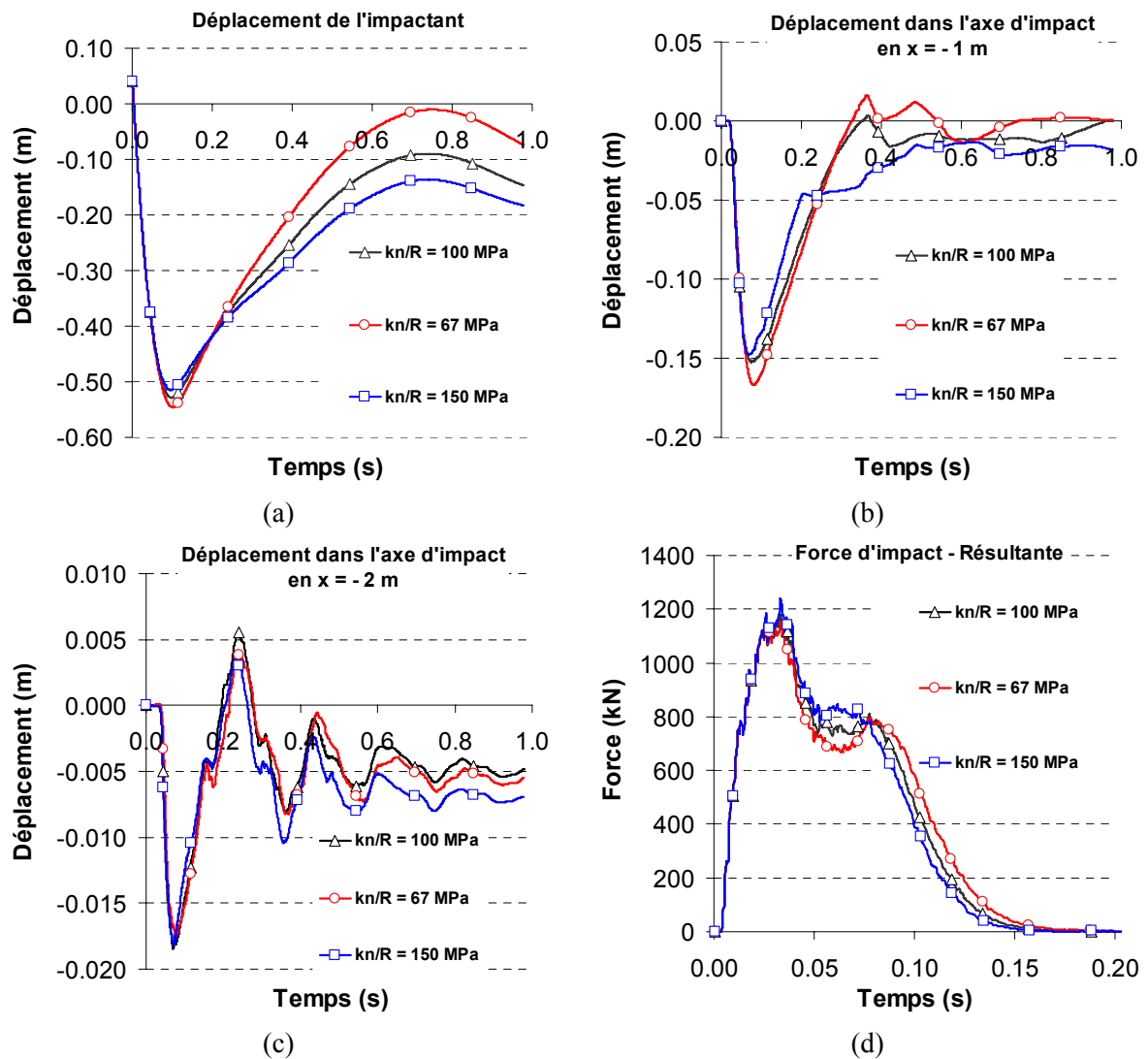
Figure A 23 : Influence de la raideur normale k_n (à rapport des rigidités contant) du matériau de remplissage des gabions « sable + pneus », sur le calcul du déplacement horizontal de l'impactant (a), à l'interface parement-noyau (b), à l'interface noyau-remblai (c), et de la force d'impact (d), pour un impact à 500 kJ d'énergie.
