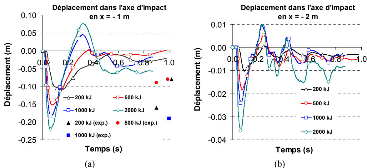
Figure 4-43 : Déplacements horizontaux en x = -1 m obtenus numériquement pour différents niveaux d'énergie d'impact, et comparaison avec les données expérimentales (a). Déplacements horizontaux en x = -2 m obtenus pour différents niveaux d'énergie d'impact.
