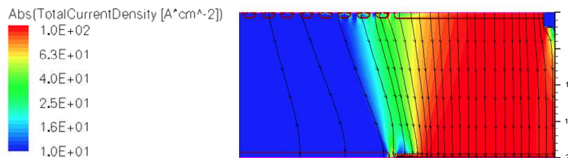
Figure 4-15. Répartition des lignes de courant pour un fort niveau de courant
