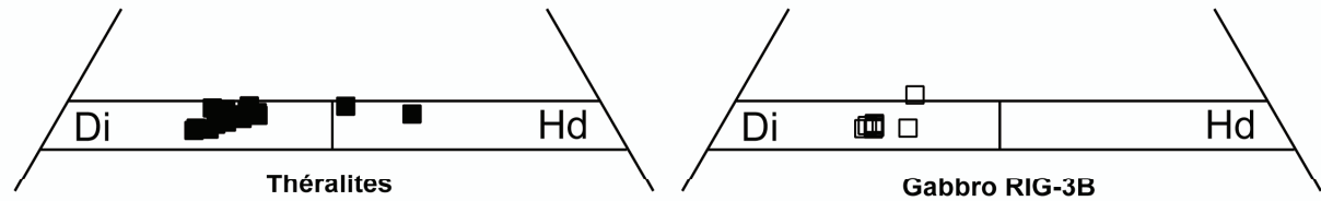
FIG. IV.1: Classification des clinopyroxènes ferro-magnésiens des roches à texture grossière des massifs de Tahiti Nui et Raiatea. A - Clinopyroxènes de Tahiti Nui: en encadré figure le schéma général de classification des pyroxènes ferro-magnésiens (Morimoto 1988). Les analyses sont reportés, pour chaque type de roche, dans un extrait du diagramme délimité par un trait pointillé dans l'encadré. Les coeurs des cristaux sont représentés par les symboles pleins, et les bords par des symboles vides. B - Clinopyroxènes de Raiatea: Les analyses sont reportés dans le même extrait du diagramme de classification que dans le cas de Tahiti Nui. Les clinopyroxènes des théralites sont représentées par les carrés pleins et ceux du gabbro RIG-3B par les carrés vides.
