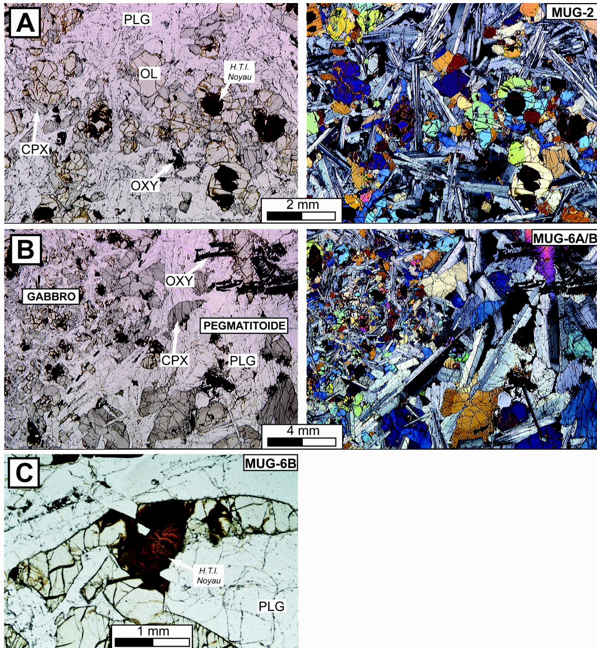
FIG. III.8: Photographies des lames-minces représentatives des deux faciès de l'intrusion gabbroïque du Faataufi (Maupiti): A - Gabbro MUG-2 à texture équilibrée. L'H.T.I. se présente en noyaux au coeur de certains cristaux d'olivine. B - Pegmatitoïde trachy-basaltique MUG-6B en contact (trait pointillé) avec le gabbro encaissant MUG-6A. Cette pegmatitoïde semble d'affinité oïcoerystique. C - Détail de la pegmatitoïde MUG-6B montrant un cristal xénomorphe d'olivine qui comporte en son coeur un noyau d'H.T.I. semblable à ceux remarqués dans le gabbro hôte.
