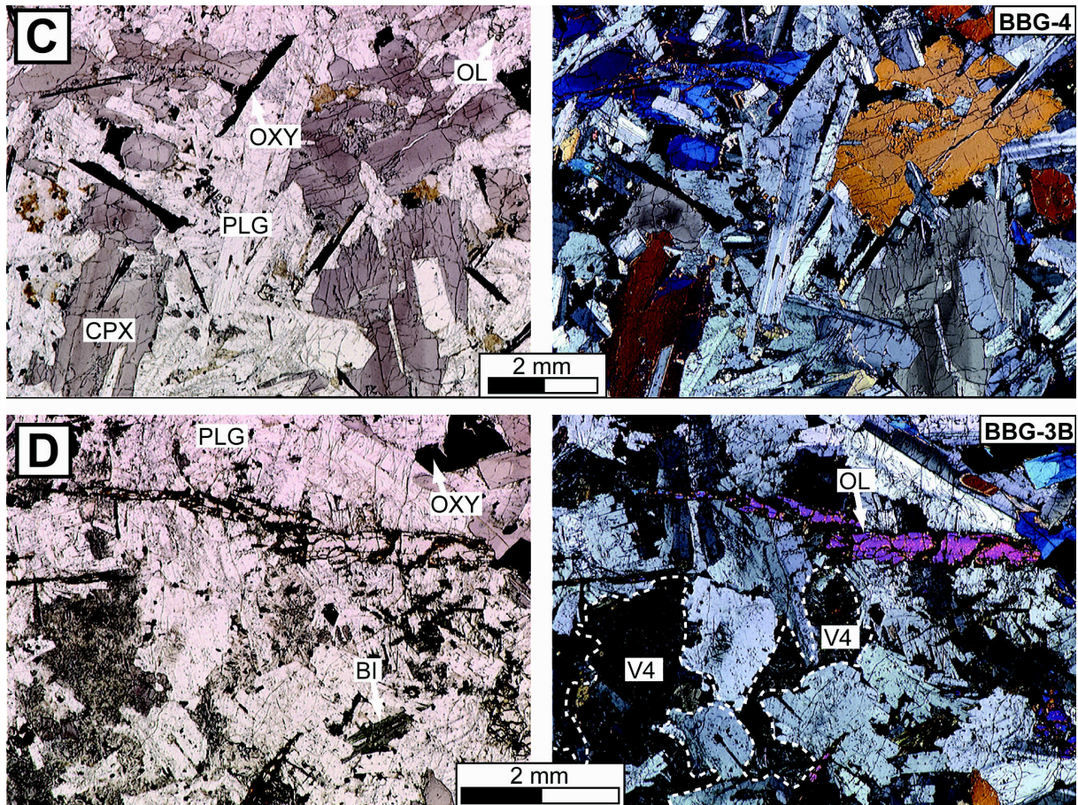
FIG. III.7 - suite: Photographies des lames-minces représentatives des roches de l'intrusion pegmatitoïdique de la Cloche de Hiro (Bora Bora): C - Pegmatitoïde trachy-basaltique BBG-4, texture pegmatitoïdique d'affinité oikocrystique. D - Pegmatitoïde téphritique BBG-3B, texture pegmatitoïdique d'affinité équigranulaire. L'image met l'accent sur un cristal d'olivine aciculaire plurimillimétrique ainsi que sur une vésicule de ségrégation de forme complexe remplie d'un matériel microlitique en partie altéré (V4).
