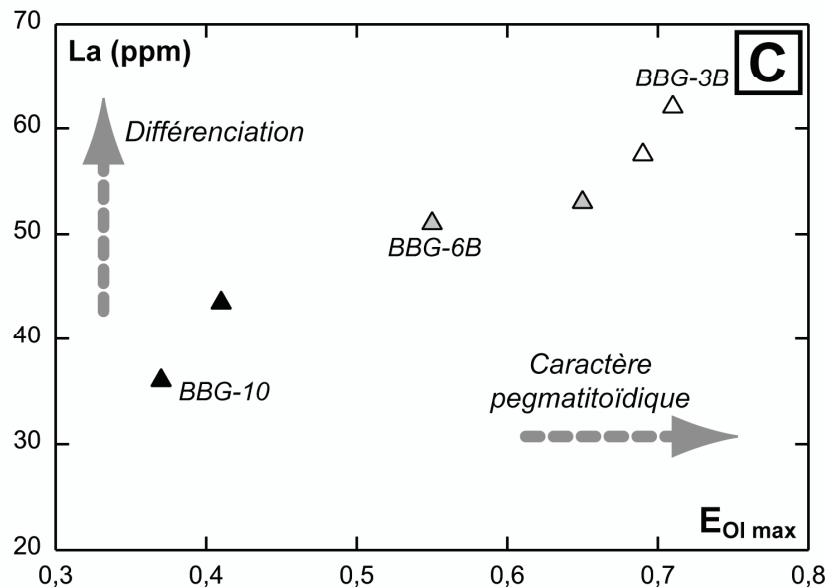
FIG. VIII.9C: Diagramme montrant, pour les échantillons de la Cloche de Hiro pris en compte lors des analyses cristallographiques, l'évolution de la teneur en La (ppm) en fonction du paramètre d'élongation des olivines. La valeur de ce paramètre, défini dans la partie B (article soumis au Journal of Petrology), est fonction du caractère pegmatitoïdique de la roche considérée.
