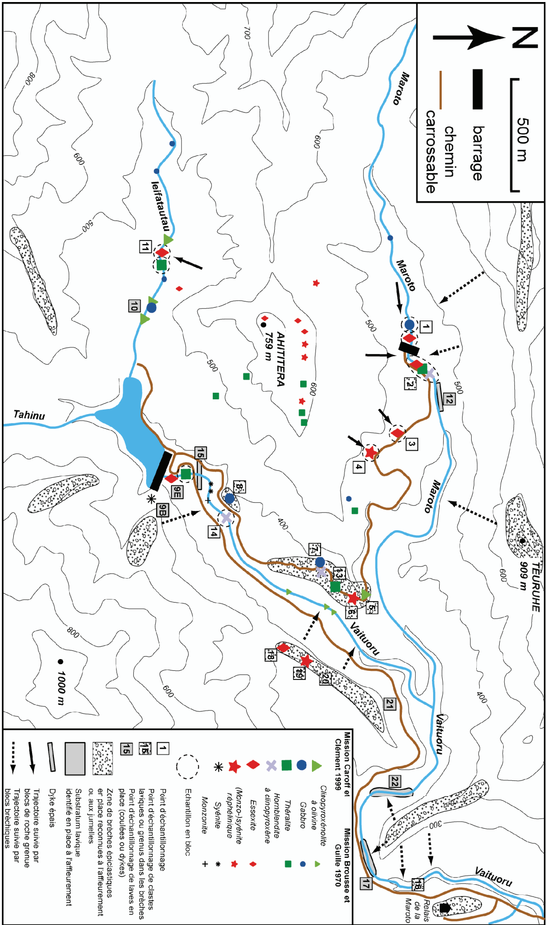
FIG. II.4: Carte d'échantillonnage de la zone d'affleurement du massif de roches grenues de Ahititera et de son environnement. Y figurent les échantillons de roche grenue collectés lors des deux missions de 1999 et 1970 (Nitecki Novotny 1975). N.B.: les échantillons grenus indiqués à l'intérieur de zones bréchiques ont été collectés en tant que clastes dans ces brèches.
