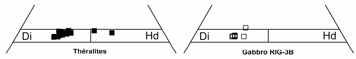
FIG. IV.1: Classification des clinopyroxènes ferro-magnésiens des roches à texture grossière des massifs de Tahiti Nui et Raiatea. A - Clinopyroxènes de Tahiti Nui: en encadré figure le schéma général de classification des pyroxènes ferro-magnésiens (Morimoto 1988). Les analyses sont reportés, pour chaque type de roche, dans un extrait du diagramme délimité par un trait pointillé dans l'encadré. Les coeurs des cristaux sont représentés par les symboles pleins, et les bords par des symboles vides. B - Clinopyroxènes de Raiatea: Les analyses sont reportés dans le même extrait du diagramme de classification que dans le cas de Tahiti Nui. Les clinopyroxènes des théralites sont représentées par les carrés pleins et ceux du gabbro RIG-3B par les carrés vides.
