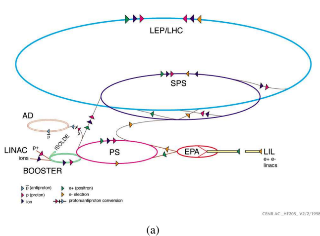
FIGURE III.1: Représentation du complexe d'accélération dont le LHC est le dernier maillon (a) et emplacement des détecteurs et de certains points stratégiques autour de cet anneau (b).
