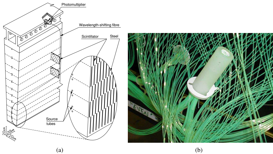
FIGURE III.22: Détail de l'assemblage de couches d'acier et de tuiles scintillantes formant un module du calorimètre hadronique à tuiles (a) et groupement de fibres optiques en amont des photo-multiplicateurs (b).
