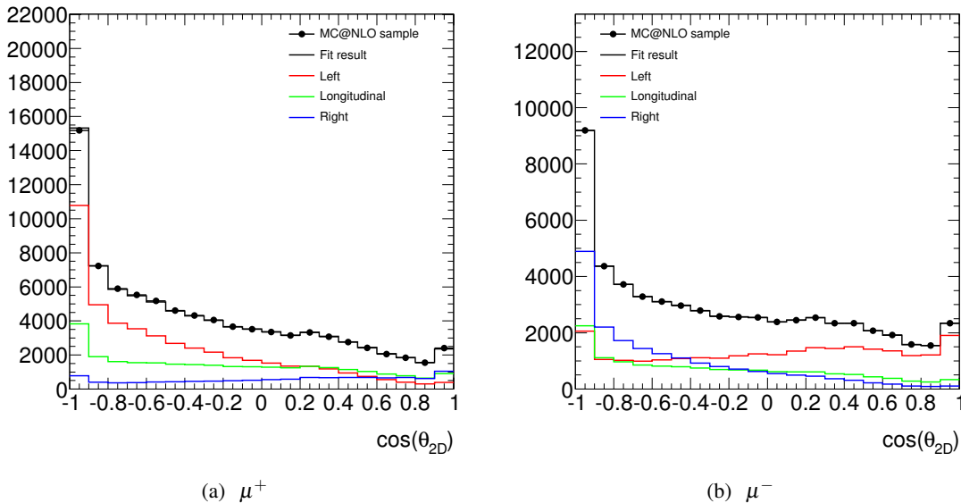
FIGURE VII.11: Résultats des ajustements par les templates d'hélicité sur \cos\theta_{2D} , pour les muons, dans des événements Monte-Carlo où le W a une impulsion transverse comprise entre 35 et 50 GeV, après simulation du détecteur. Les distributions rouges représentent les contributions du template gauche, les bleues celle du template droit et les vertes celles du template longitudinal. Les lignes noires représentent les sommes des différentes contributions.
