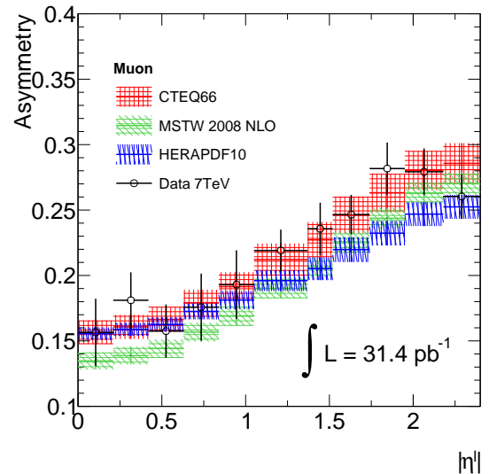
FIGURE VIII.13: Évolution des valeurs d'asymétrie de charge en fonction de la pseudo-rapacité des muons, dans les données (noirs) et dans le Monte-Carlo en utilisant différents jeux de PDFs.
