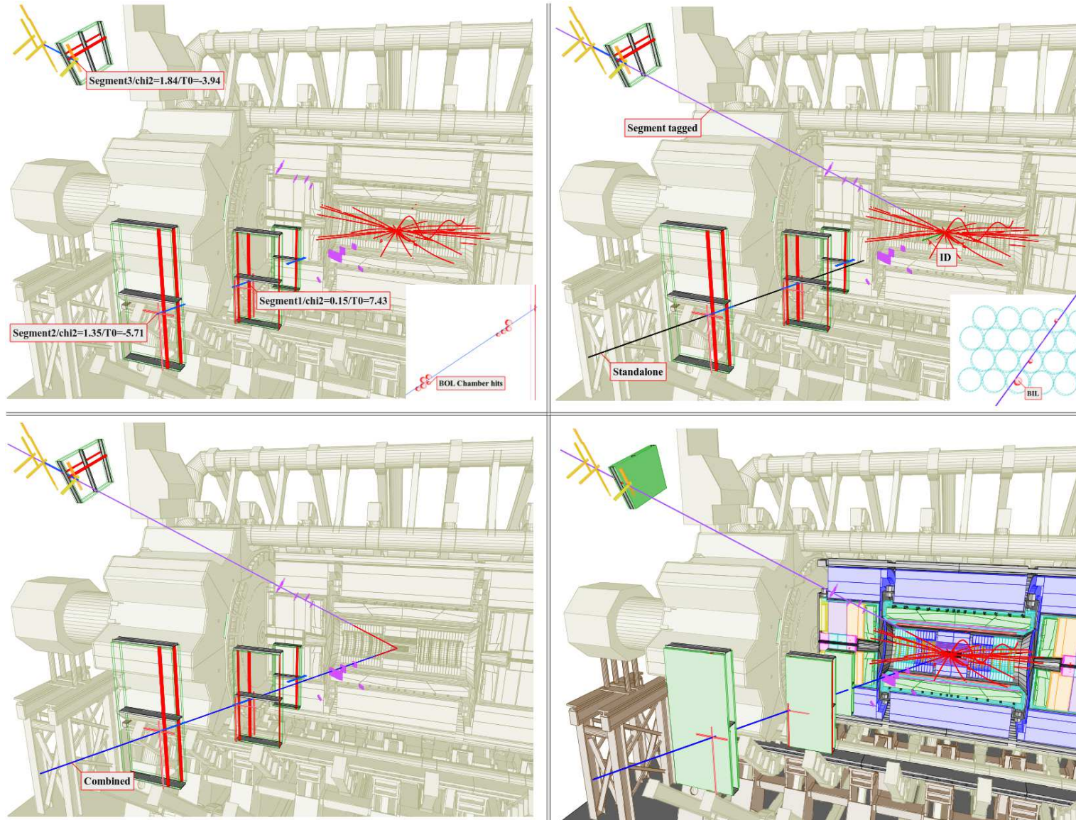
FIGURE V.13: Schéma des quatre étapes de reconstruction d'un muon combiné dans un événement Z \rightarrow \mu\mu issu des données. Les deux premières étapes (partie supérieure gauche) consistent à isoler les régions d'activités grâce aux informations des RPCs/TGCs et reconstruire une droite par chambre (dans cette image un des muons est tag car il ne passe que par une seule chambre, seul l'autre sera détaillé par la suite). la partie supérieure droite montre la reconstruction de la trace standalone du muon en passant par les trois chambres activées. Finalement la partie inférieure gauche montre l'association faite entre les deux traces du spectromètre et deux des traces du détecteur interne.
