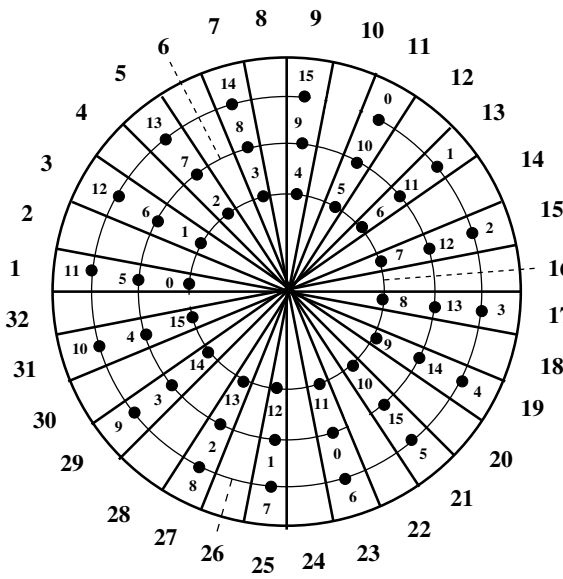
FIGURE IV.12: Emplacement des 48 sondes de la roue HEC1 sur leurs anneaux respectifs.
