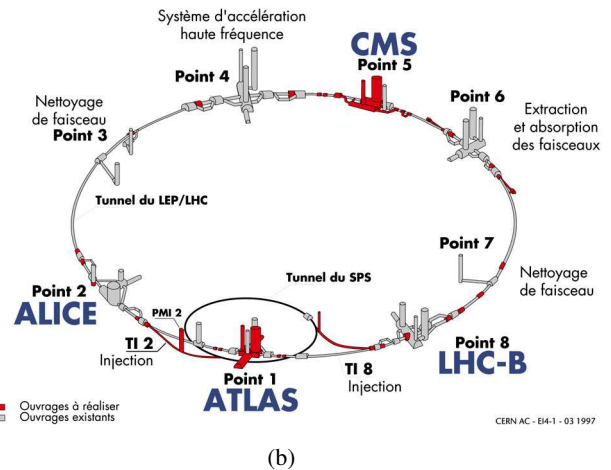
FIGURE III.1: Représentation du complexe d'accélération dont le LHC est le dernier maillon (a) et emplacement des détecteurs et de certains points stratégiques autour de cet anneau (b).
