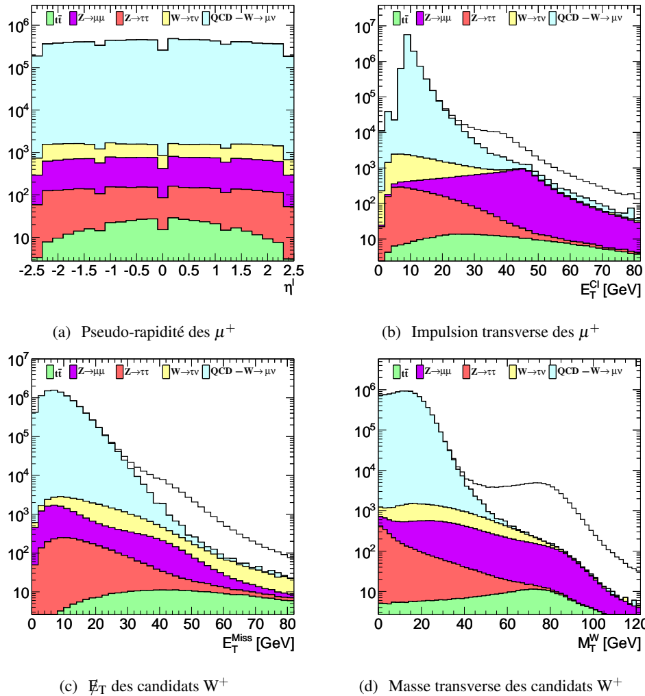
FIGURE VI.2: Distribution de pseudo-rapidité du lepton (a), d'impulsion transverse du lepton (b), d'énergie transverse manquante (c) et de masse transverse du W (d) pour les candidats W^+ du Monte-Carlo. Toutes les coupures de sélection sont appliquées à l'exception du déclenchement et des trois coupures cinématiques ( p_T^\ell , \cancel{E}_T et M_T^W ).
