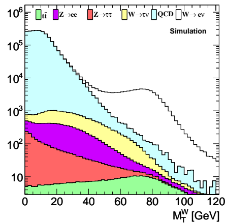
(d) Masse transverse des candidats W^+
