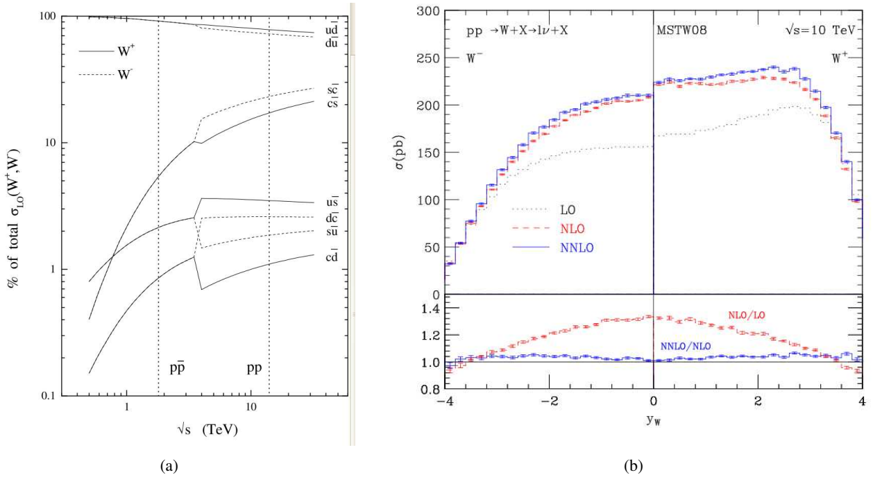
FIGURE I.6: (a) Pourcentage de la section efficace totale de production LO de bosons W^+ et W^- , selon les paires de quark-antiquark considérées, en fonction de \sqrt{s} [34]. (b) Section efficace de production des bosons W^- (gauche) et W^+ (droite) en fonction de y_W pour différents ordres de calcul de perturbation QCD (LO, NLO et NNLO) [35]
