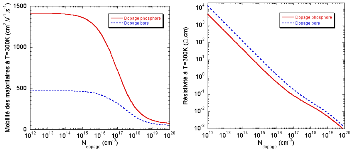
(a) Mobilité des porteurs majoritaires.
