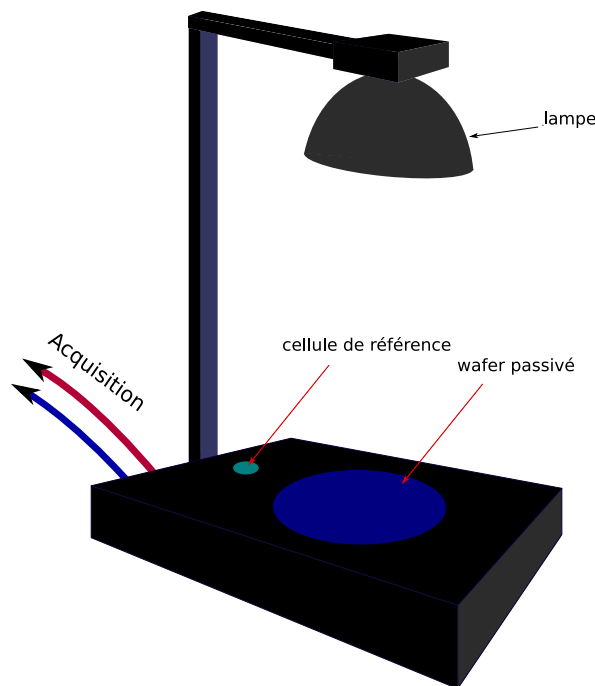
FIGURE 3.7 – Représentation du WCT-120.
