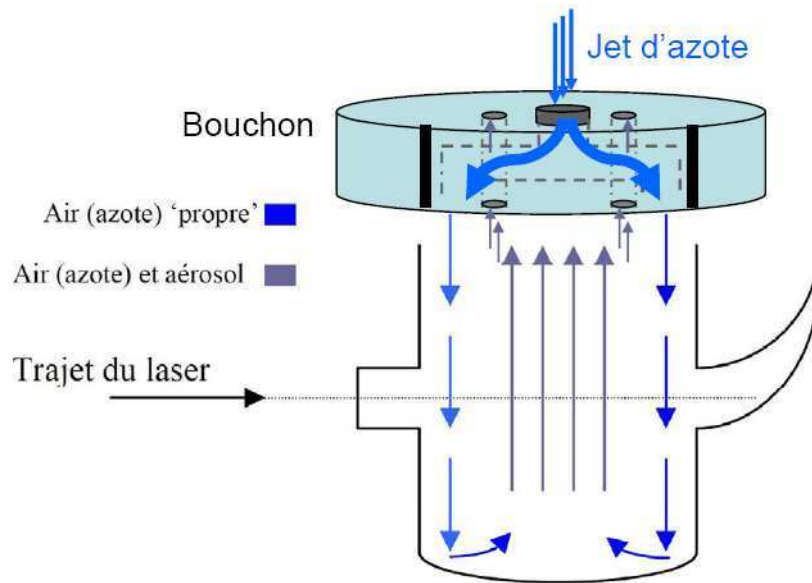
Figure 27 : Principe de fonctionnement de lévitation des particules par jet d'azote dans la fiole
