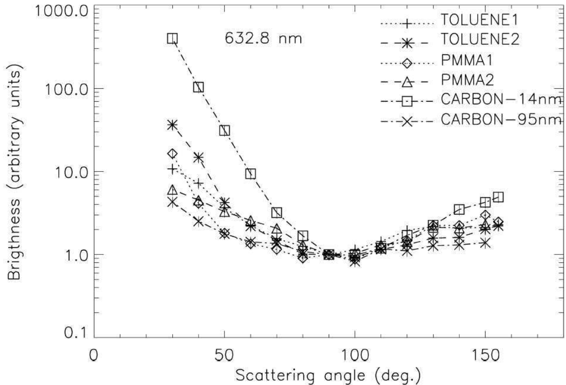
Figure 104 : Les courbes d'intensité normalisées à 90° d'angle de diffusion produite par l'ensemble complet d'agglomérats de suie en lévitation et de noir de carbone à \lambda = 632,8 nm.
