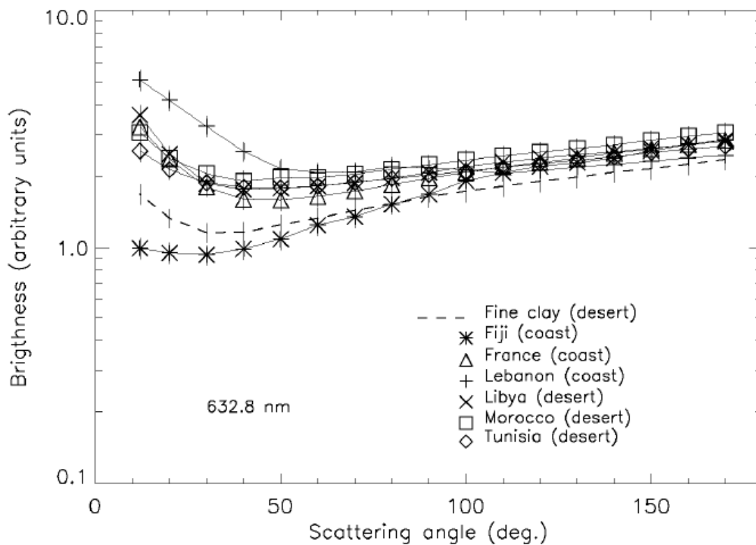
Figure 42 : Courbes de radiance produites par les échantillons de sable déposés, à \lambda= 632,8 nm.
