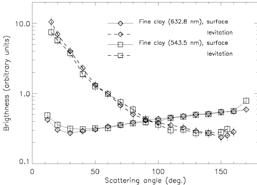
Figure 52 : Comparaison entre les courbes de radiance produites par l'échantillon argile fine déposé et en lévitation, mesuré à \lambda = 632,8 et à \lambda = 543,5 nm.
