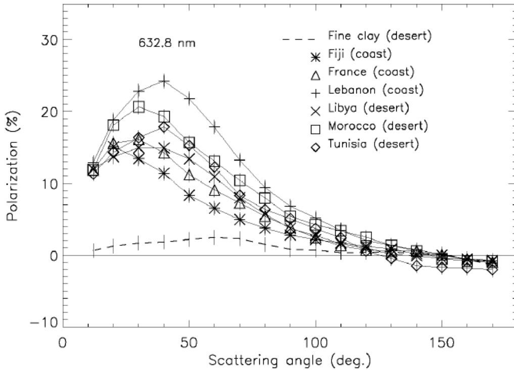
Figure 40 : Courbes de polarisation produites par les échantillons déposés, à \lambda= 632,8 nm.
