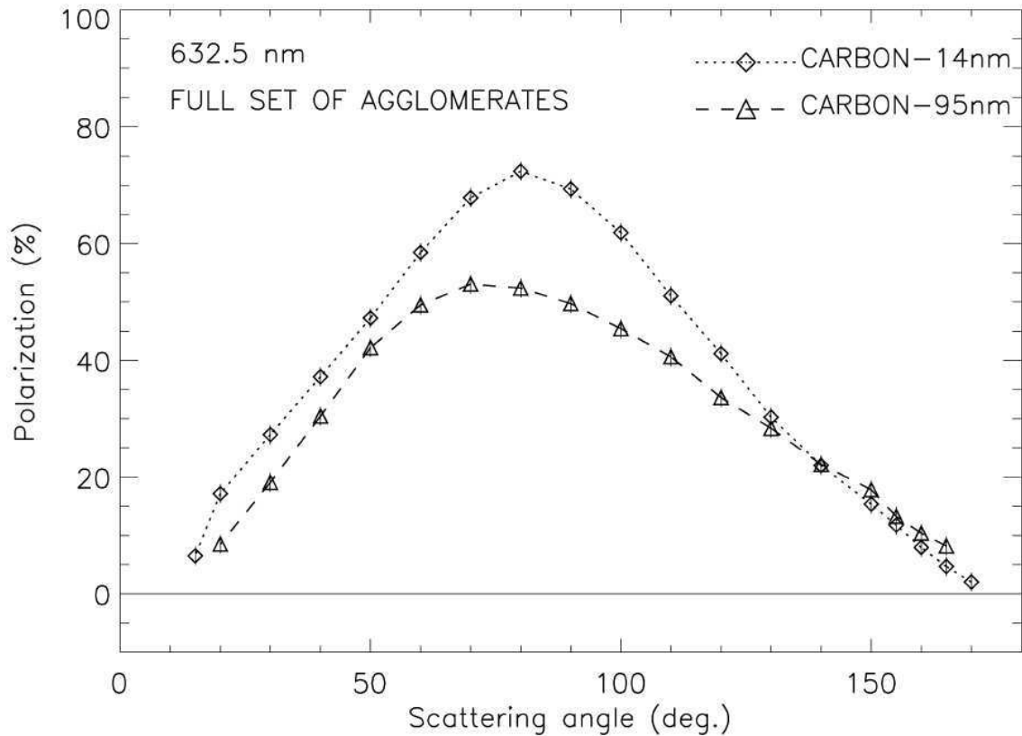
Figure 93 : Courbes de polarisation à \lambda = 632,8 nm produites par l'ensemble complet d'agglomérats des deux échantillons de noir de carbone: C14 et C95 en lévitation.
