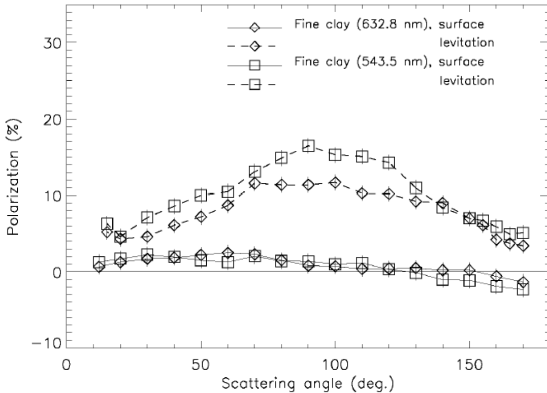
Figure 51 : Comparaison entre les courbes de polarisation produites par l'échantillon argile fine déposée et en lévitation, mesurées à \lambda = 632,8 et à \lambda = 543,5 nm.
