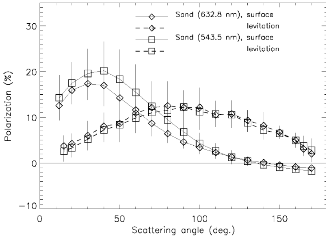
Figure 48 : Courbes de polarisation synthétiques des échantillons de sable à l'exception du sable noir, à \lambda = 632,8 nm et \lambda = 543,5 nm. Les marges d'erreur correspondent à la dispersion des courbes individuelles.
