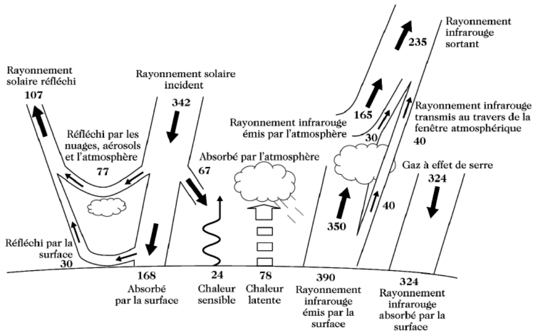
Figure 2 : Bilan d'énergie journalier dans l'atmosphère terrestre en W/m^2 pour une température de surface de 15^\circ C . Extrait de Kiehl et Trenberth (1997)
