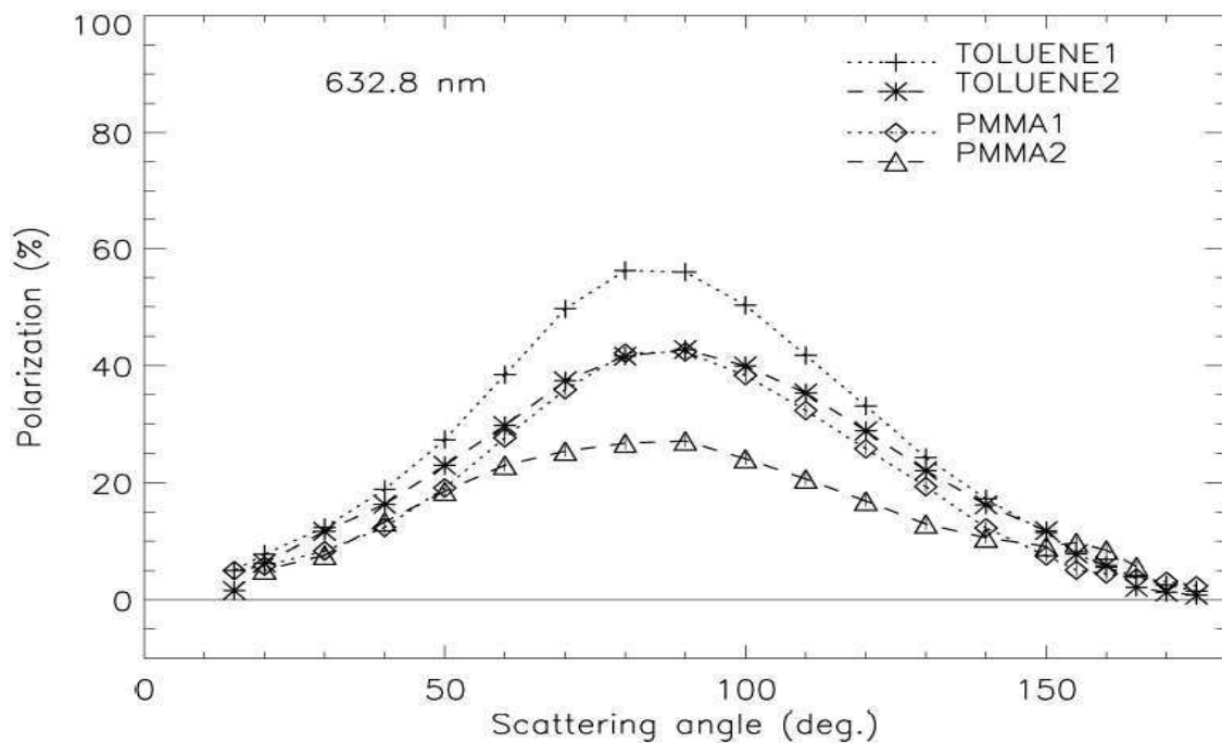
Figure 87 : Courbes de polarisation à \lambda = 632,8 nm produites par l'ensemble complet d'agglomérats de suies en lévitation.
