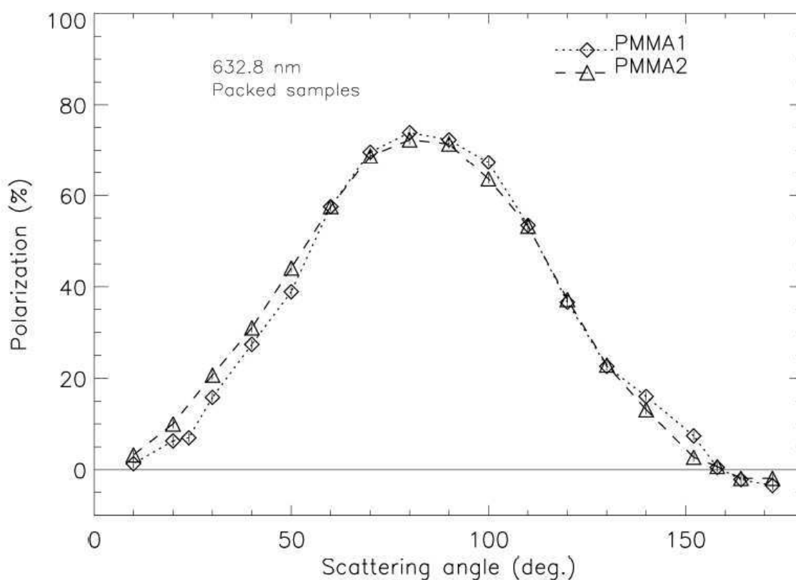
Figure 85 : Courbes de polarisation à \lambda = 632,8 nm produites par les échantillons de suies tassées en surface
