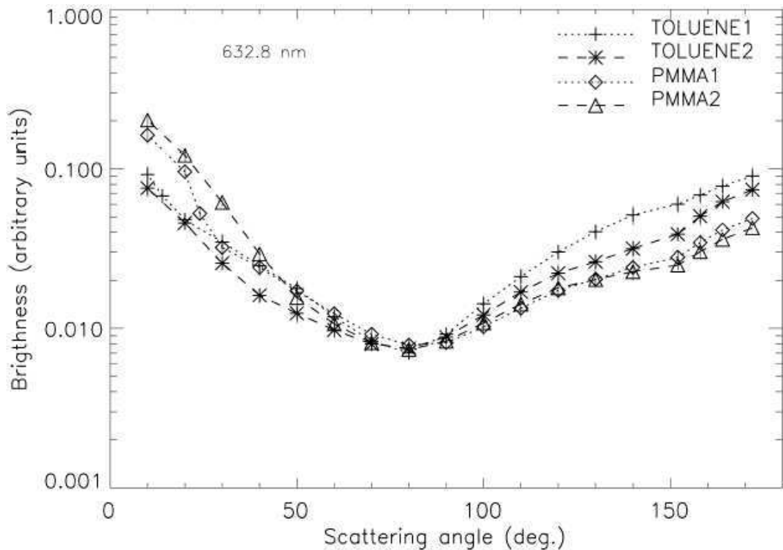
Figure 105 : Les courbes de radiance normalisées à 80^\circ d'angle de diffusion produites par les suies en surface à \lambda = 632,8 nm.
