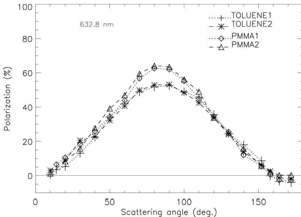
Figure 84 : Courbes de polarisation à \lambda = 632,8 nm produites par les échantillons de suies déposées en surface
