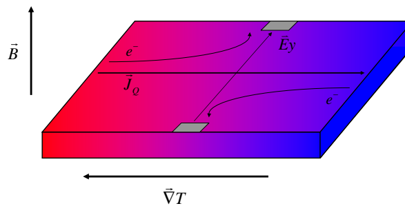
Figure 1.13 – Compensation de Sondheimer. Le dégradé de couleur représente la diffusion de la chaleur due au gradient thermique (rouge = chaud, bleu = froid).
