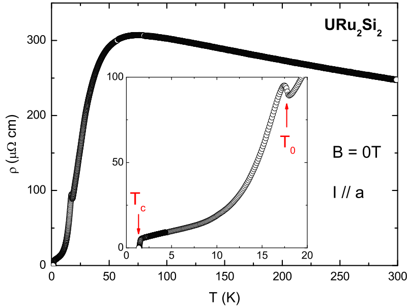
Figure 6.5 – Résistivité de URu 2 Si 2 en fonction de la température à champ magnétique nul pour un courant I//a . Dans l'insert sont montrées un zoom entre la transition ordre caché à T_0 = 17.5 K et la transition supraconductrice à T_c = 1.5 K.
