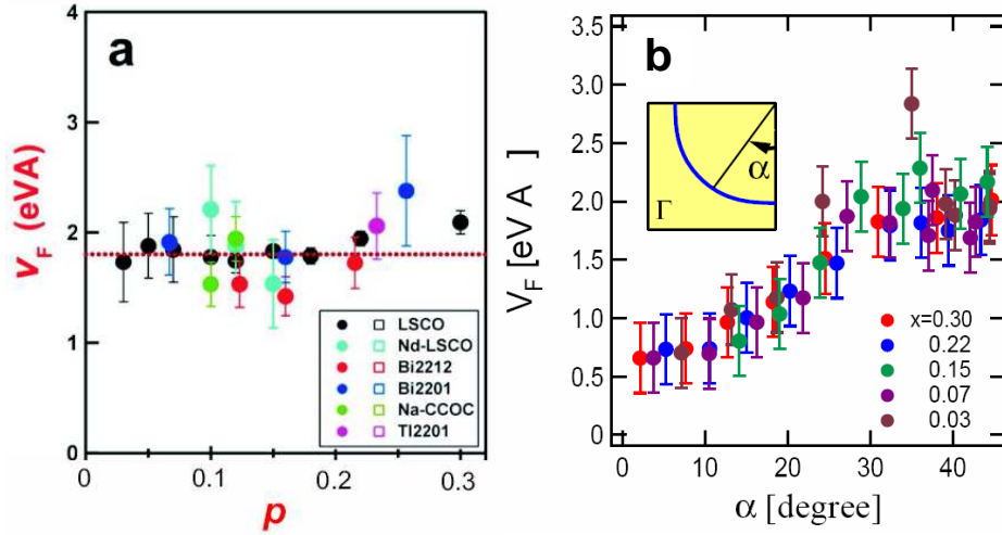
Figure 5.14 – a) Dépendance avec le dopage de la vitesse de Fermi dans les régions nodales ( 1 \text{ eV\AA} \approx 1.39 \times 10^5 \text{ ms}^{-1} ) [237]. D'après les mesures d'ARPES, la vitesse de Fermi est constante en (\pi, \pi) pour tout dopage 0.03 < x < 0.3 . b) Vitesse de Fermi autour de la surface de Fermi (un quadrant) de la région antinodale à la région nodale [238]. La vitesse de Fermi ne montre pas de dépendance avec le dopage et sature également en (0, \pi) .
