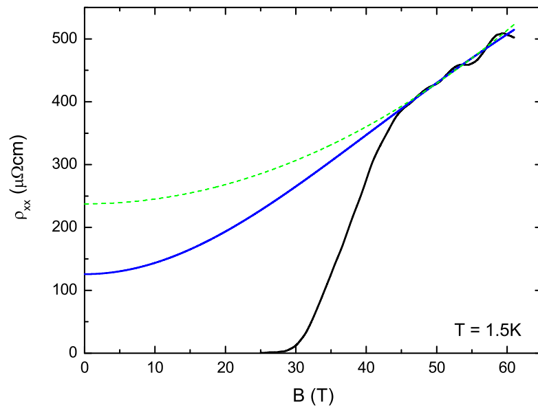
Figure 5.9 – Fit de la magnétorésistance transverse à T= 1.5\text{ K} et haut champ avec la formule 1.34 décrivant le comportement de la magnétorésistance dans un modèle à deux bandes (trait plein) et avec une simple dépendance en B^2 (ligne en pointillé).
