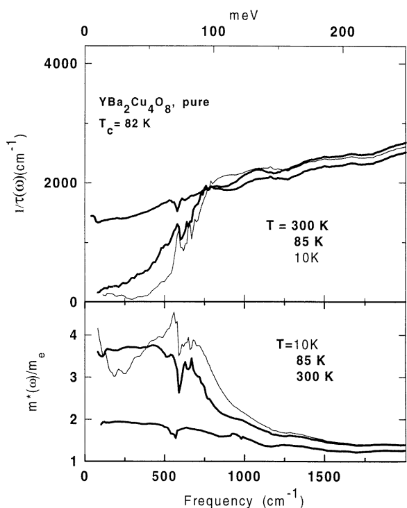
Figure 2.22 – Dépendance en fréquence du taux de diffusion dans Y124 pour trois températures. Le taux de diffusion est quasiment linéaire pour les trois températures au dessus de 750\text{ cm}^{-1} . Une chute du taux de diffusion, associée au pseudogap se développe juste au dessus de T_c [129].
