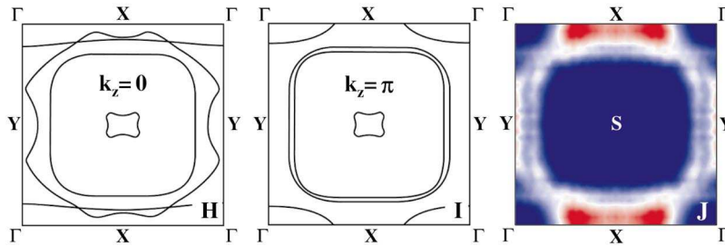
Figure 5.6 – Surface de Fermi de \text{YBa}_2\text{Cu}_3\text{O}_7 déterminée à partir des calculs de structure de bandes LDA [199]. Le quadrant de droite représente la mesure d’ARPES [200] effectuée dans ce composé. On observe un bon accord avec les calculs LDA. D’après [201].
