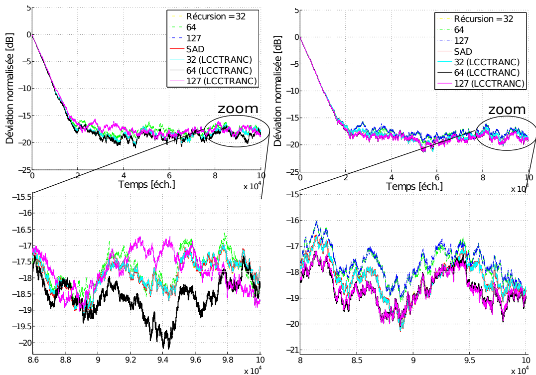
Figure 4.11 – Evolution de la déviation normalisée des filtres w_{21} (gauche) et w_{12} (droit) pour un mélange de deux sources blanches gaussiennes de même puissance \sigma_{s_1}^2 = \sigma_{s_2}^2 = 1 . Les pas d'adaptation sont fixés à 0,01.
