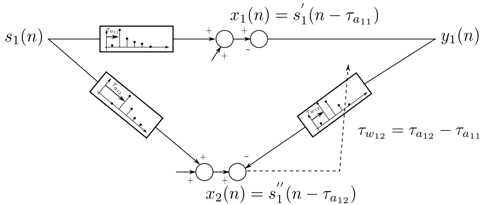
Figure 6.8 – Influence des chemins directs sur les filtres adaptatifs calculés. Illustration pour le filtre w_{12} .
