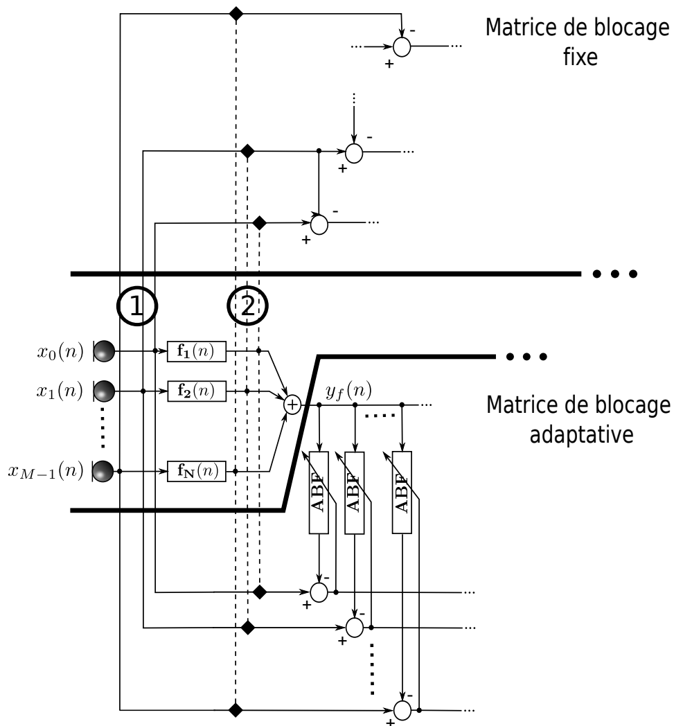
Figure 6.11 – Configurations possibles pour la création des signaux de référence de bruit. La configuration 1 utilise les signaux captés par les microphones. La configuration 2 correspond à la récupération des signaux après filtrage par l'antenne sur chacune des voies.
