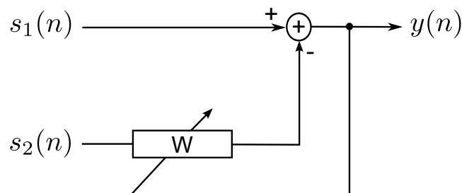
Figure 6.2 – Structure de l’annuleur de bruit adaptatif (ANC) classique.
