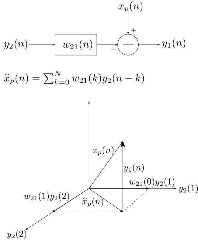
Figure 2.9 – Interprétation géométrique du problème d'estimation basé sur l'erreur quadratique moyenne. Cas du filtre à deux coefficients.
