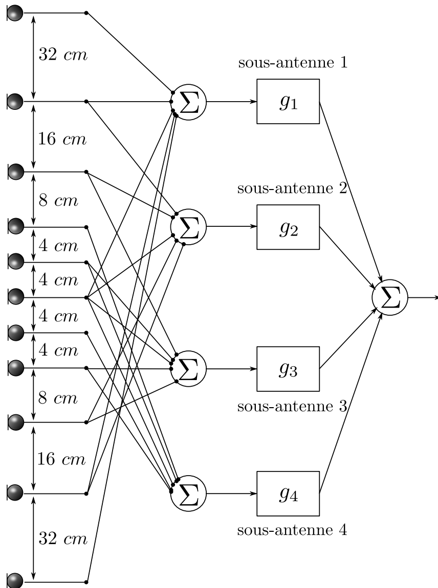
Figure 6.14 – Antenne rectiligne logarithmique composée de 11 microphones groupés en 4 sous-antennes. La distance inter-capteur n'est pas respectée sur ce schéma (doublement des distances d'une antenne à l'autre).
