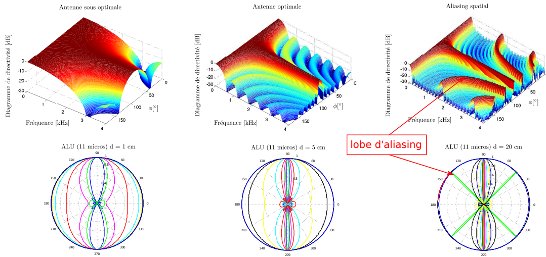
Figure 1.8 – Diagramme de directivité de l’antenne ALU composée de 11 microphones pour d valant (de gauche à droite) 1, 5 et 20 cm. La distance d = 5 cm (milieu) correspond à l’antenne optimale pour l’onde de fréquence f = 3400 Hz. A gauche, nous illustrons le cas d’une antenne sous-optimale, à droite le phénomène de repliement spatial. Le code de couleur utilisé pour les directivités dans le plan n’a pas de lien avec les directivités 3D, il sert seulement à la lisibilité.
