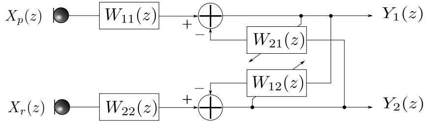
Figure 2.4 – Structure réursive à quatre filtres pour la séparation d'un mélange convolutif de deux sources.
