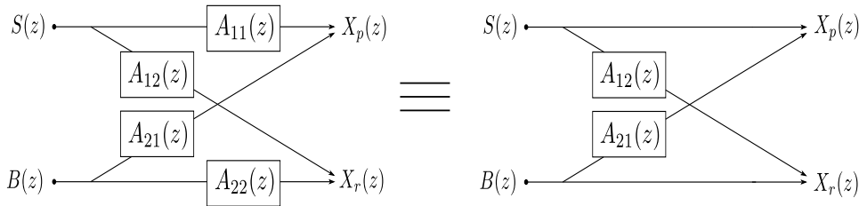
Figure 2.5 – Modèle de mélange simplifié compatible avec une propagation en champ proche.
