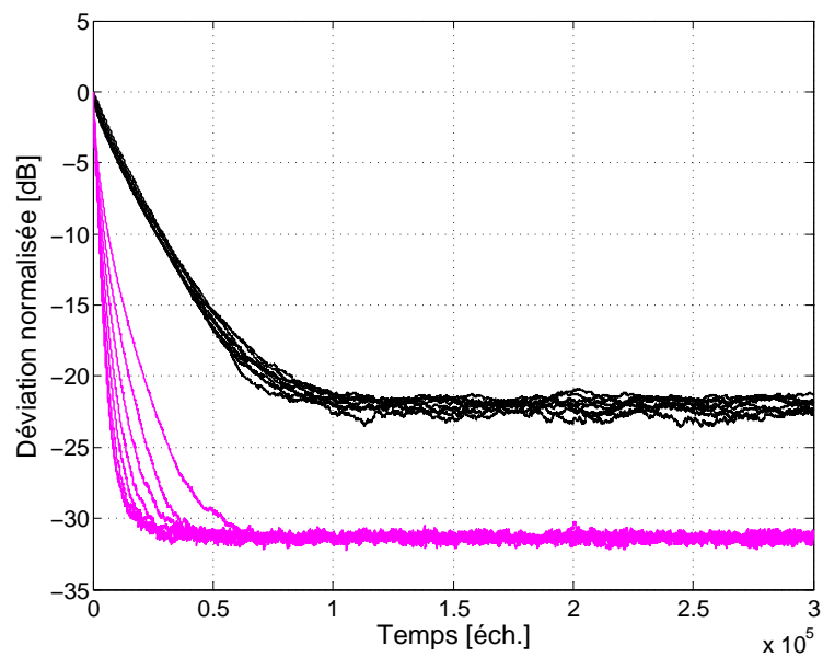
Figure 5.7 – Evolution temporelle de \|\Delta \mathbf{a}_{21}(n)\|^2 / \|\mathbf{a}_{21}(n)\|^2 (noir) et \|\Delta \mathbf{a}_{12}(n)\|^2 / \|\mathbf{a}_{12}(n)\|^2 (magenta) pour différentes valeurs du pôle \alpha = 0, 0.1, 0.2, \dots, 0.9 .
