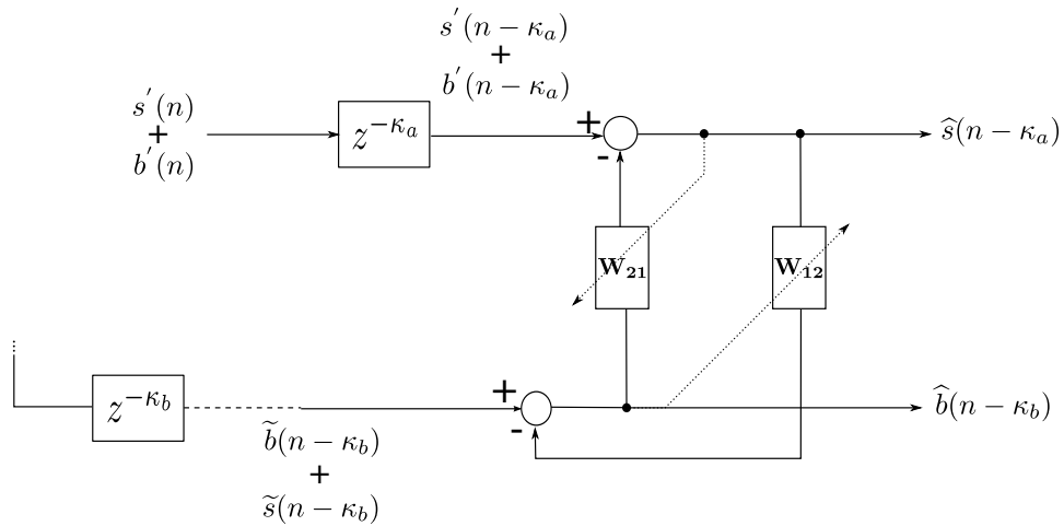
Figure 6.12 – Analyse de l'influence des retards sur la structure réursive.
