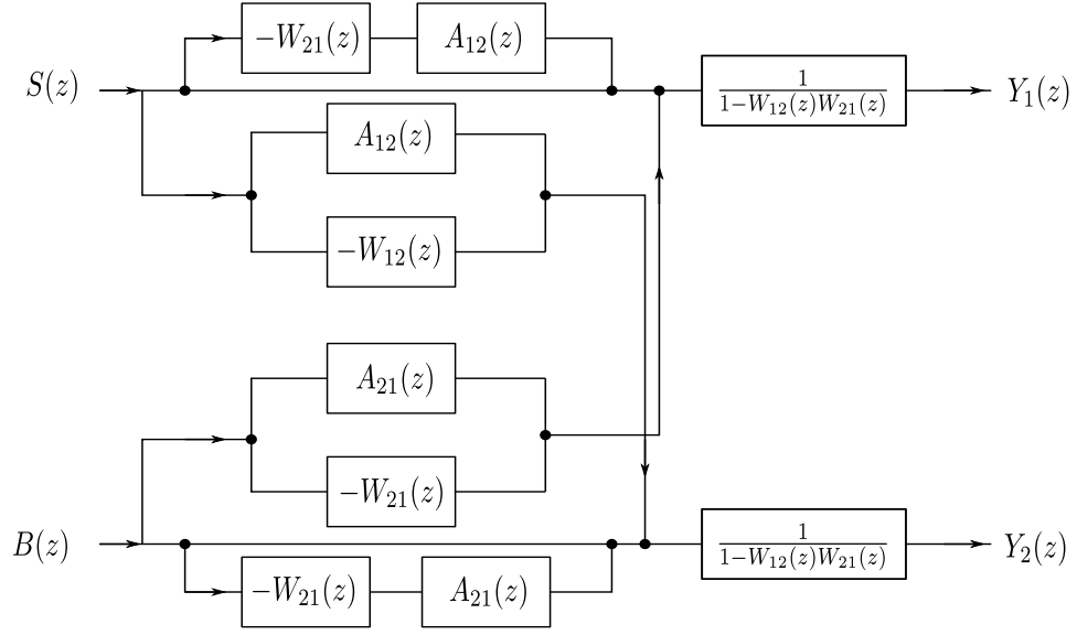
Figure 2.6 – Schéma bloc représentant les relations d'entrée-sortie associées à la structure récur-sive.
