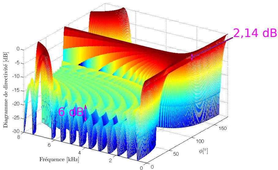
Figure 1.11 – Directivité de l’antenne ALU dans le cas d’incertitude sur la position des micros, la valeur des gains et la direction de la source utile ( \sigma_g = 0,1 , \sigma_\Phi = 10^\circ et \sigma_p = 0,01\text{ m} ).
