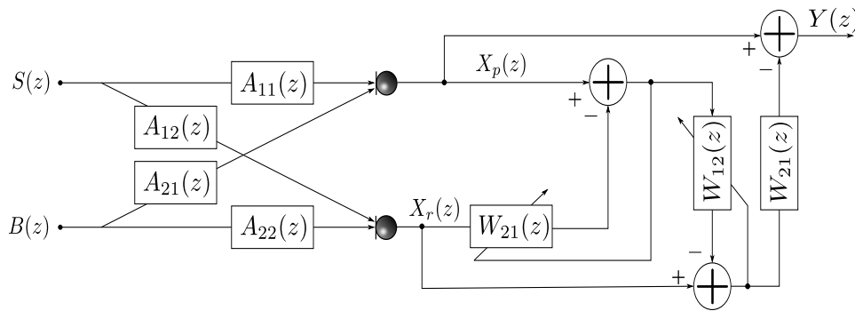
(b) Annuleur de bruit avec pré-traitement.
