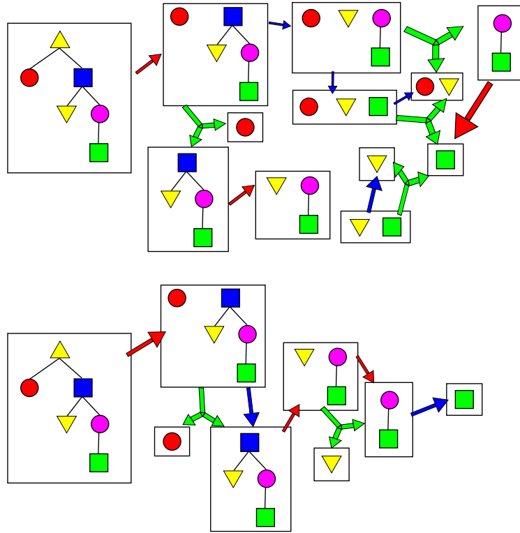
FIG. 2.29 – Décompositions produites par l’algorithme de Zhang et Shasha. Les flèches rouges indiquent une décomposition résultant de la partie 2.2 de la formule. Les flèches bleues indiquent la déletion de la racine de l’arbre gauche/droit de la forêt. Les flèches vertes indiquent la séparation du calcul d’une forêt en arbre gauche/droit et forêt restante. En haut, la décomposition suivant l’utilisation des sous-arbres enracinés aux racines gauches. En bas, la décomposition suivant l’utilisation des sous-arbres enracinés aux racines droites.
