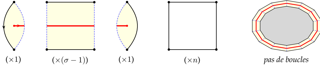
FIGURE 1.10. Modèle de chemins auto-évitants de Jérémie Bouttier et Emmanuel Guitter. Les chemins sont représentés d'un trait (rouge) épais, et les arêtes qu'ils coupent sont en pointillés fins (bleus). Le chemin part de la face de degré 2 incidente à la racine et finit dans l'autre face de degré 2. La pointe de flèche sur le chemin symbolise ce fait.
