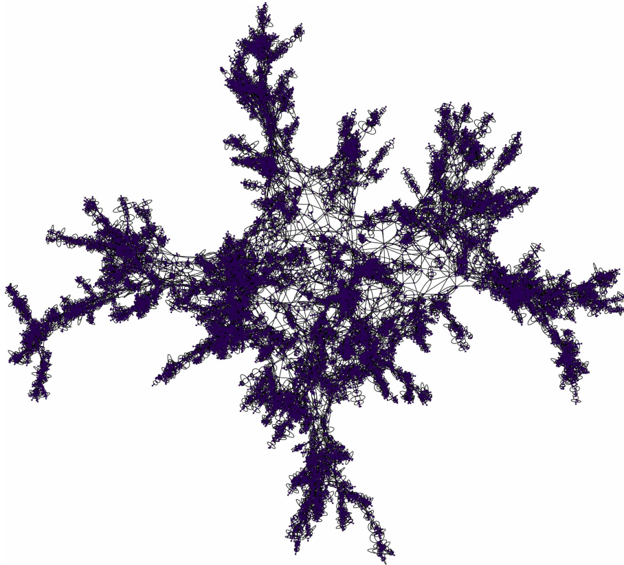
FIGURE 1.5. Simulation d'une quadrangulation planeaire uniforme à 30 000 faces réalisée par Jean-François Marckert. Cette représentation ne prend pas en compte le plongement, mais uniquement la structure de graphe sous-jacente.
