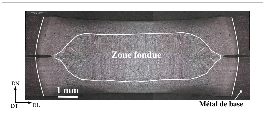
FIGURE B.1 – Observation micrographique d'une coupe transverse d'un point soudé d'acier DP780GA après attaque au nital.
