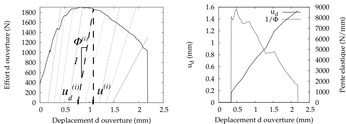
FIGURE 2.8 – (a) Détermination de la complaisance de l'éprouvette \Phi , et de l'ouverture résiduelle u_d à partir de la courbe F - u lors de la succession décharge-recharge (i). (b) Exemple d'évolution de \Phi et u_d en fonction du déplacement d'ouverture.
