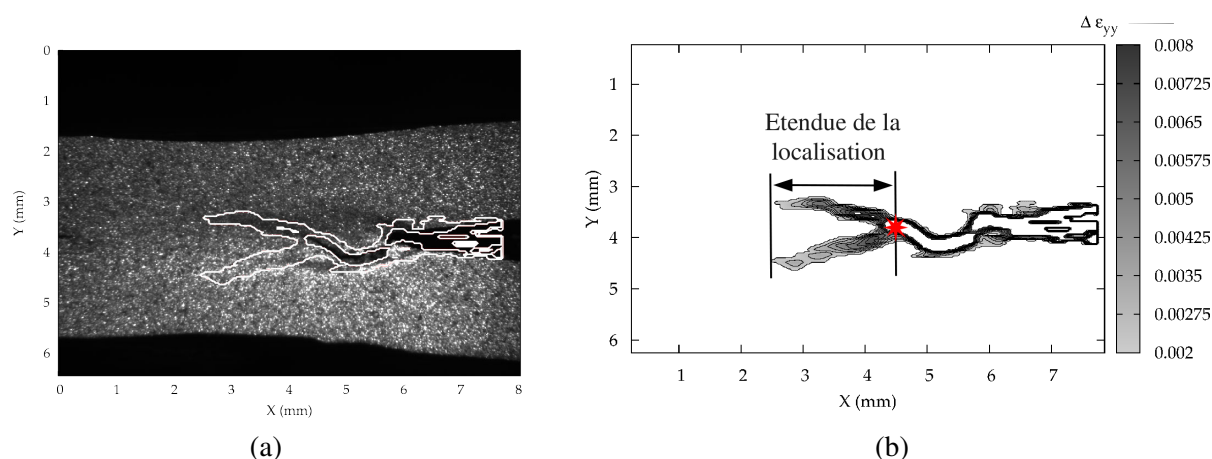
FIGURE 3.14 – Iso-valeurs du champ de déformation verticale incrémentale \Delta\varepsilon de 0,002 à 0,008. Définition de l'étendue de la localisation de la déformation. La position de la pointe de la fissure est illustrée par l'étoile.
