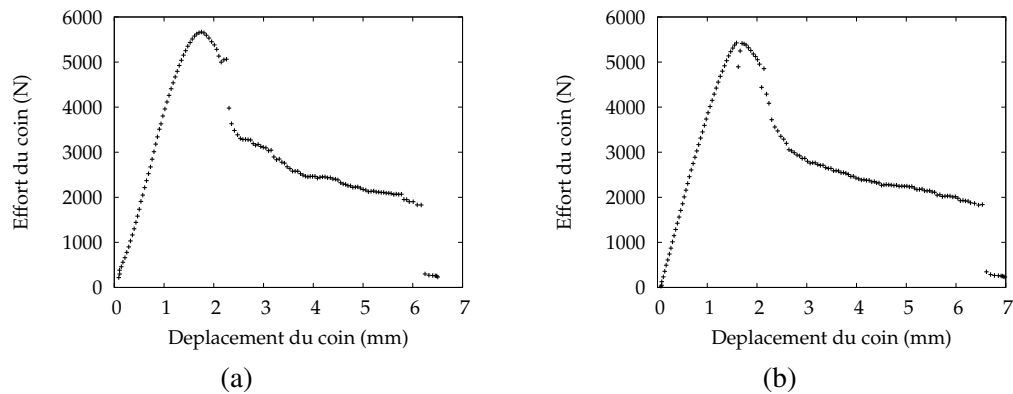
FIGURE 3.4 – Mesure de l'effort et F_{coin} en fonction du déplacement u_{coin} pour les essais n° 2 et 4.
