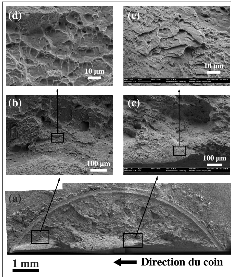
FIGURE 3.28 – Observation de la lèvres de la fissure.
