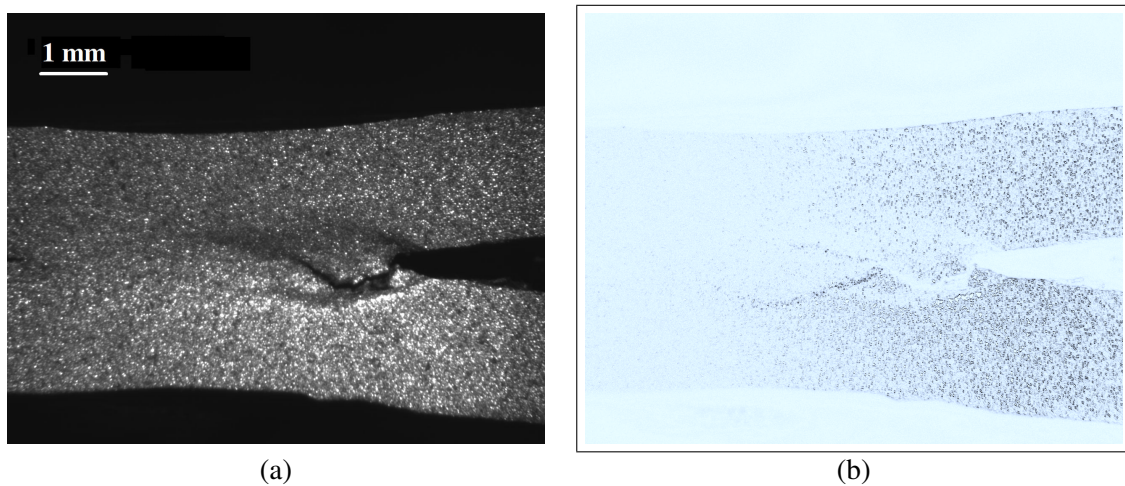
FIGURE 3.13 – (a) Exemple d'image acquise et (b) soustraction des niveaux de gris de cette dernière à l'image précédente, mettant en évidence les zones de l'image dans lesquelles le niveau de gris fut modifié de façon significative. Deux bandes de localisation en aval du front de fissure sont ainsi révélées.
