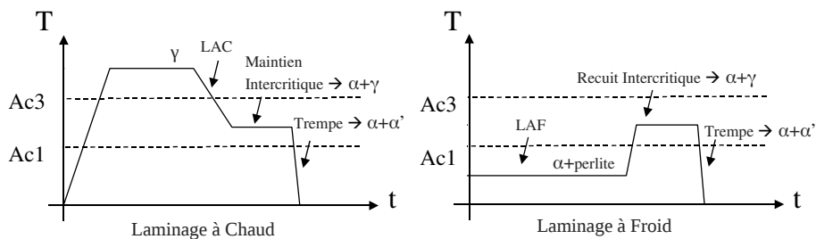
FIGURE A.3 – Cycles thermiques permettant l'obtention de microstructure dual phase par laminage à chaud et à froid [AHSS3 06].
