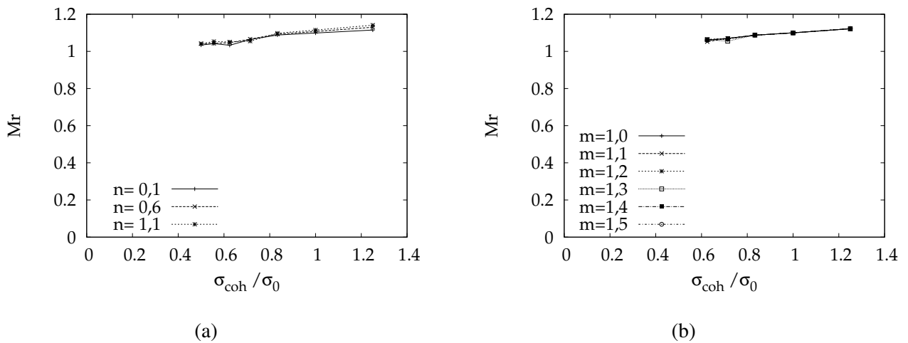
FIGURE 4.4 – Influence du comportement des poutres sur le moment fléchissant en pointe de fissure pour des poutres homogènes (a) et hétérogènes (b).
