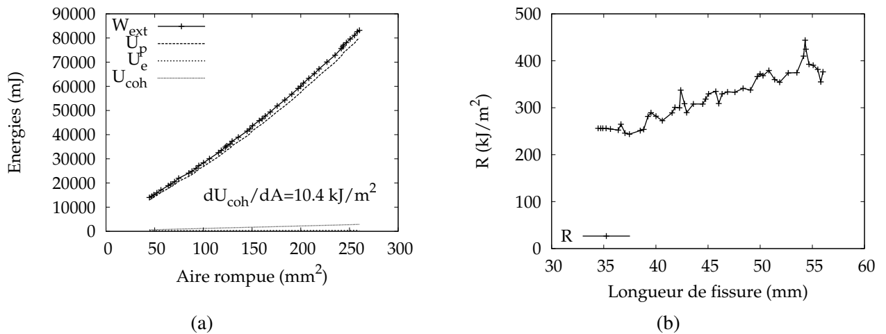
FIGURE D.7 – (a) Exemple d'évolution des énergies internes en fonction de l'aire rompue A . (b) Dérivée instantanée de U_d en fonction de l'aire rompue.
