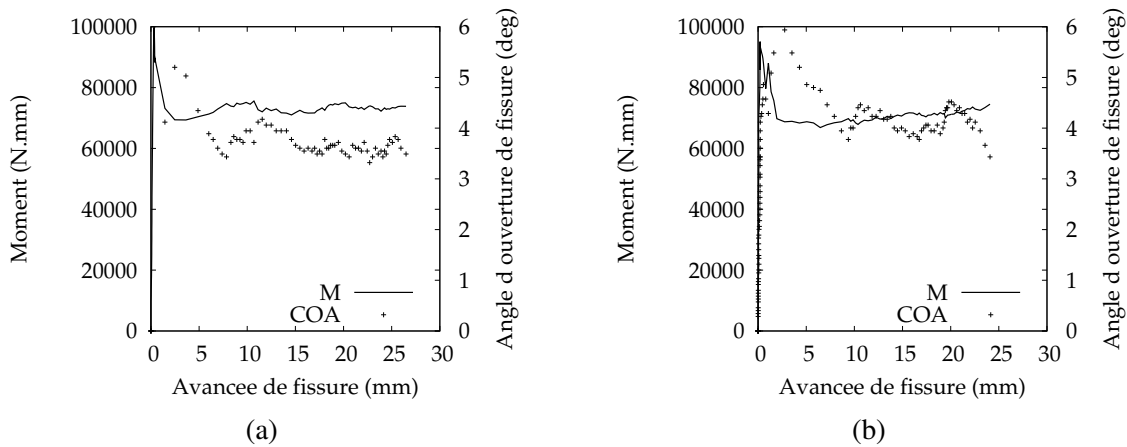
FIGURE 3.6 – Évolution du moment en pointe de fissure M et de l’angle d’ouverture de fissure \Psi en fonction de l’avancée de la fissure pour les essais n° 2 et 4.
