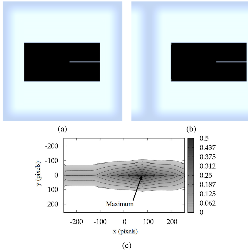
FIGURE C.6 – (a) Image initiale de 512 x512 pixels après fenêtrage de Hanning et filtrage gaussien. (b) Image décalée de 76,3 pixels en abscisse, 0 pixels en ordonnées. (c) Produit d'inter-corrélation associé montrant un maximum pour une ordonnée y nulle et une abscisse x=76 .
