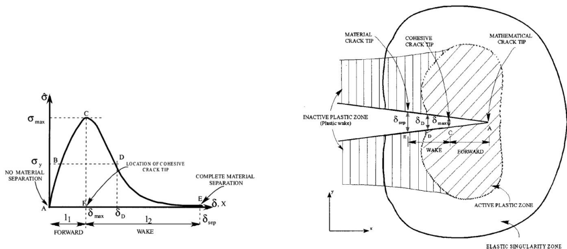
FIGURE 1.32 – (a) Exemple typique de loi cohésive (b) Interprétation de la localisation du fond d'entaille [Shet 02].
