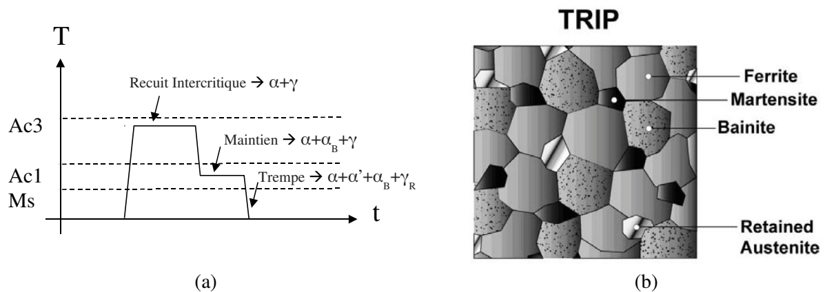
FIGURE A.5 – Cycle thermique d'obtention d'une microstructure d'acier TRIP, et schéma représentant la matrice ferritique et les phases durcissantes [AHSS3 06].
