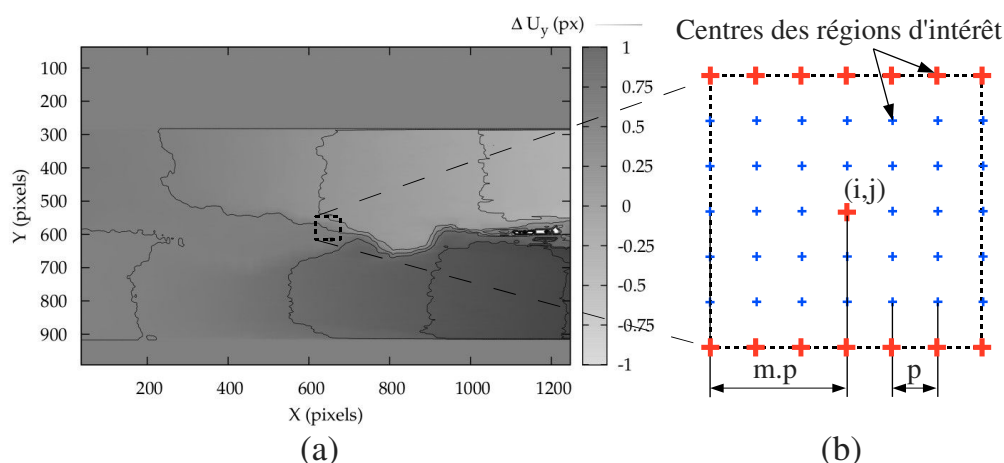
FIGURE C.11 – (a) Champ de déplacement vertical considéré et taille de la fenêtre de moyenne pour le calcul de la déformation \varepsilon_{yy} . (b) Illustration de la fenêtre de moyenne constituée d'un ensemble de noeuds de la grille de régions d'intérêt de période p pixels (croix). Sa dimension est contrôlée par le facteur de moyenne m=3 .
