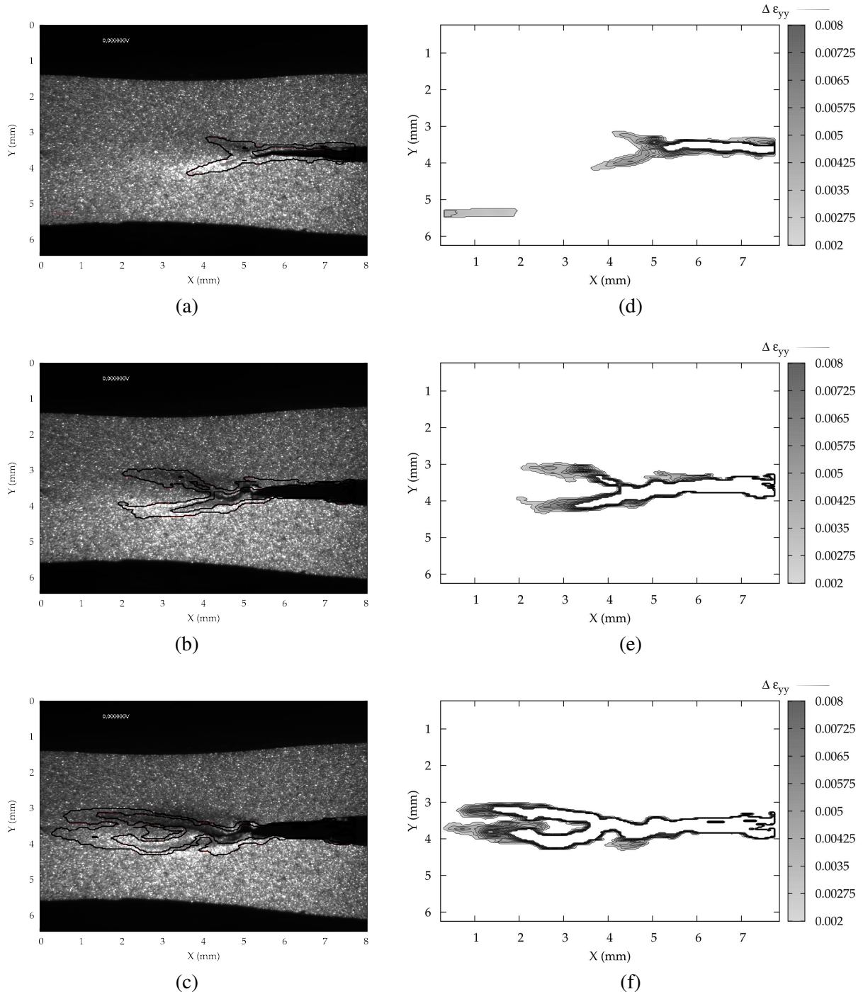
FIGURE 3.15 – Évolutions de la zone à fort incrément de déformation à trois instants de l’essai A. Les images acquises sont présentées en (a), (b) et (c). Les isovalues du champ de déformation verticale incrémentale \Delta\epsilon de 0,002 à 0,008 sont illustrées par les figures (d), (e) et (f). Ces dernières isovalues sont également représentées sur les images acquises.
