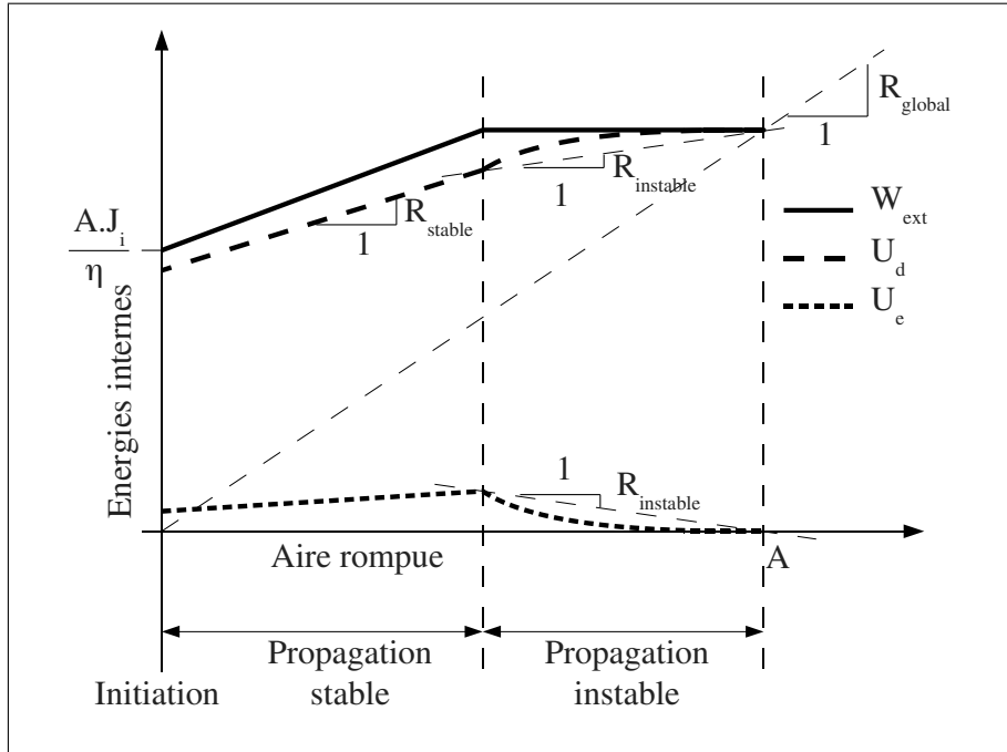
FIGURE 1.34 – Illustration schématique de l'évolution des énergies internes W_{ext} , U_e , et U_d = W_{ext} - U_e au cours d'un essai de fissuration en déplacement imposé, et définition des taux de dissipations d'énergie R_{stable} , R_{instable} et R_{global} .
