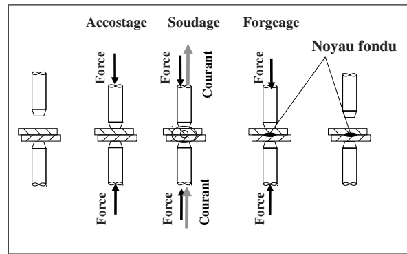
FIGURE 1.1 – Etapes du procédé de soudage par point.
