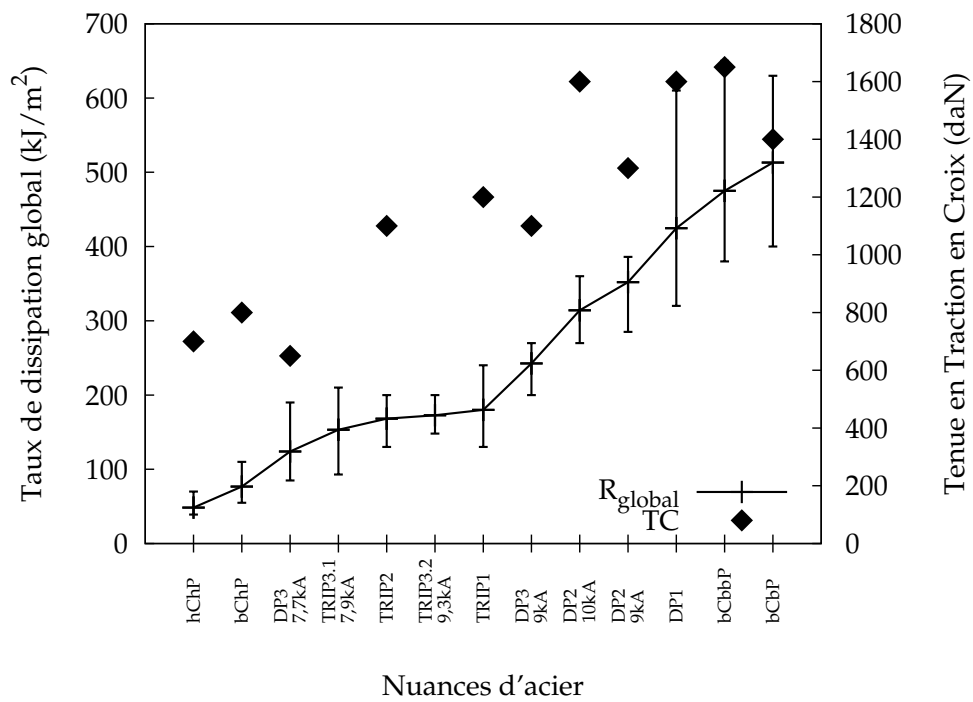
FIGURE 5.2 – Récapitulatif des mesures de taux de dissipation d'énergie globale R_{global} , et tenues en traction en croix associées.
