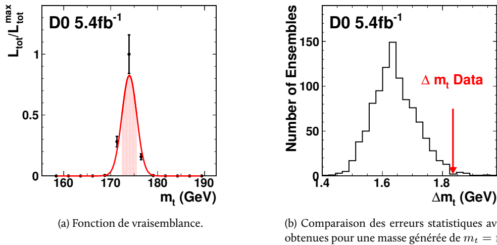
FIGURE 7.17 – Fonction de vraisemblance et comparaison de la distribution des erreurs statistiques obtenues à partir de l'ensemble de test avec la valeur corrigée de l'erreur statistique mesurée dans les données. Ces différentes grandeurs sont déjà corrigées des biais de la méthode.
