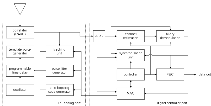
FIG. 1.9 – Exemple de synoptique d'un récepteur UWB.
