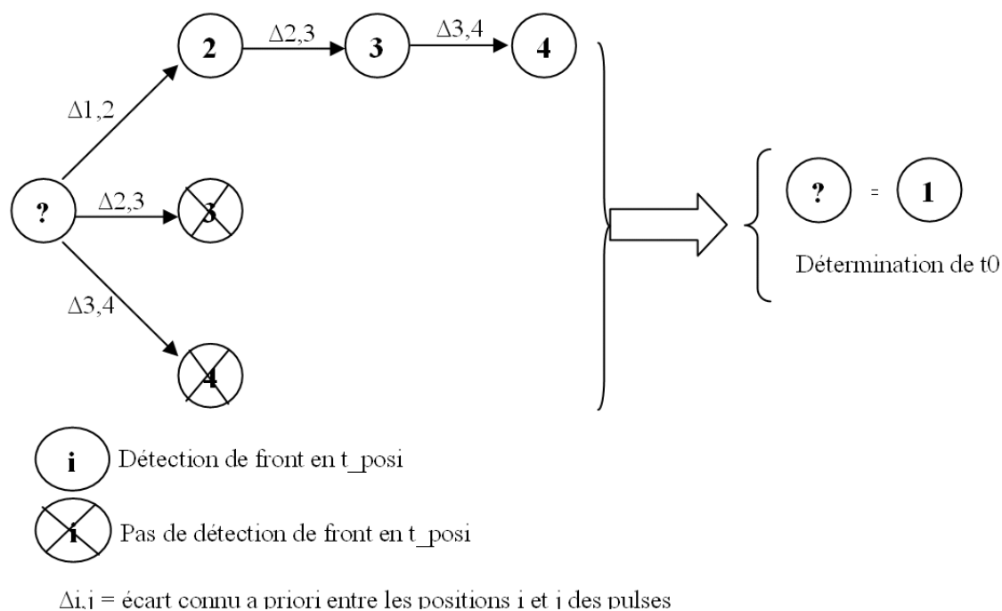
FIG. 4.24 – Schéma de l'arbre de synchronisation
