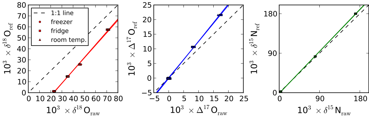
FIGURE 2.4 – Calibration de \delta^{18}O , \Delta^{17}O et \delta^{15}N mesurés par la méthode bactérienne pour les tests de stockage dans trois conditions de températures différentes. Les lignes de couleur représentent les régressions linéaires trois groupes de données pour \delta^{18}O , \Delta^{17}O et \delta^{15}N (les paramètres sont donnés dans le tableau 2.5).
