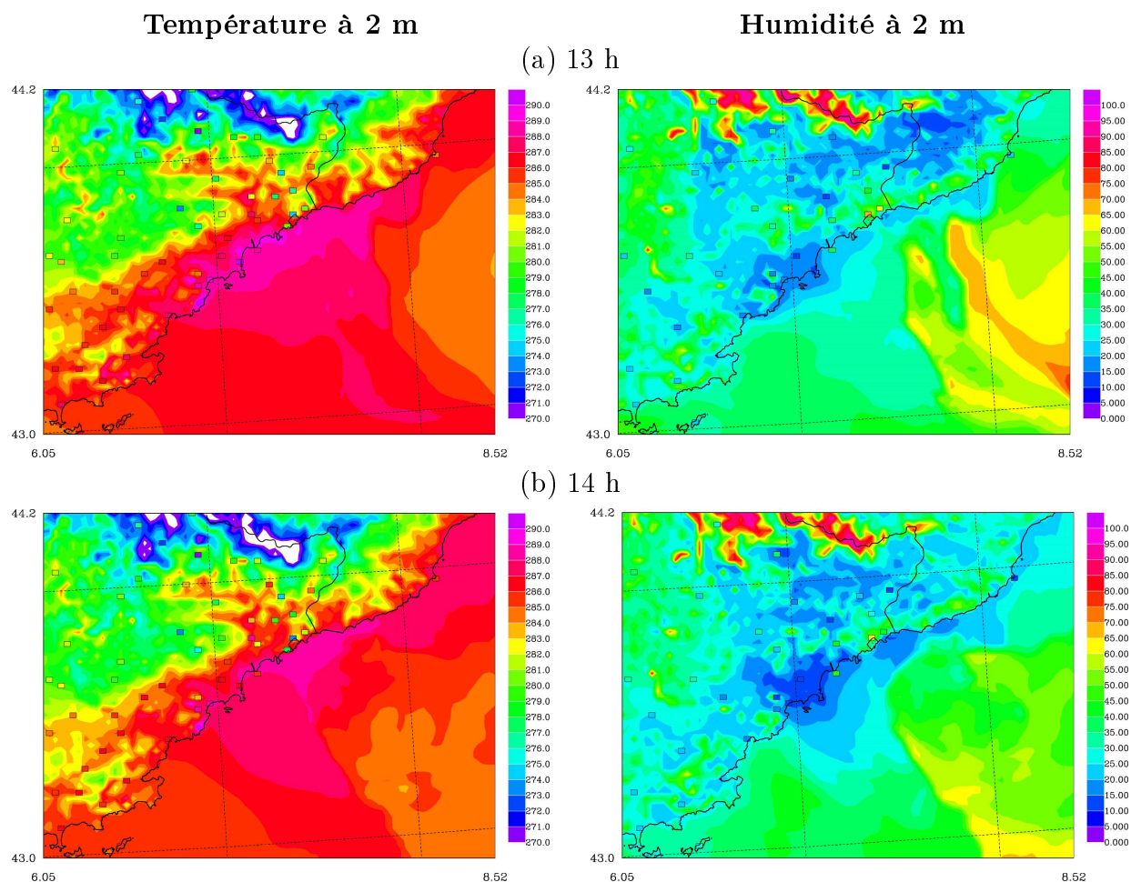
FIGURE 5.41 – Température (à gauche) et humidité (à droite) observées à 2 m (carrés de couleur) le 24 Mars 2009 à 13 h UTC (en haut) et à 14 h UTC (en bas) superposées aux champs simulés par Més0-NH.
