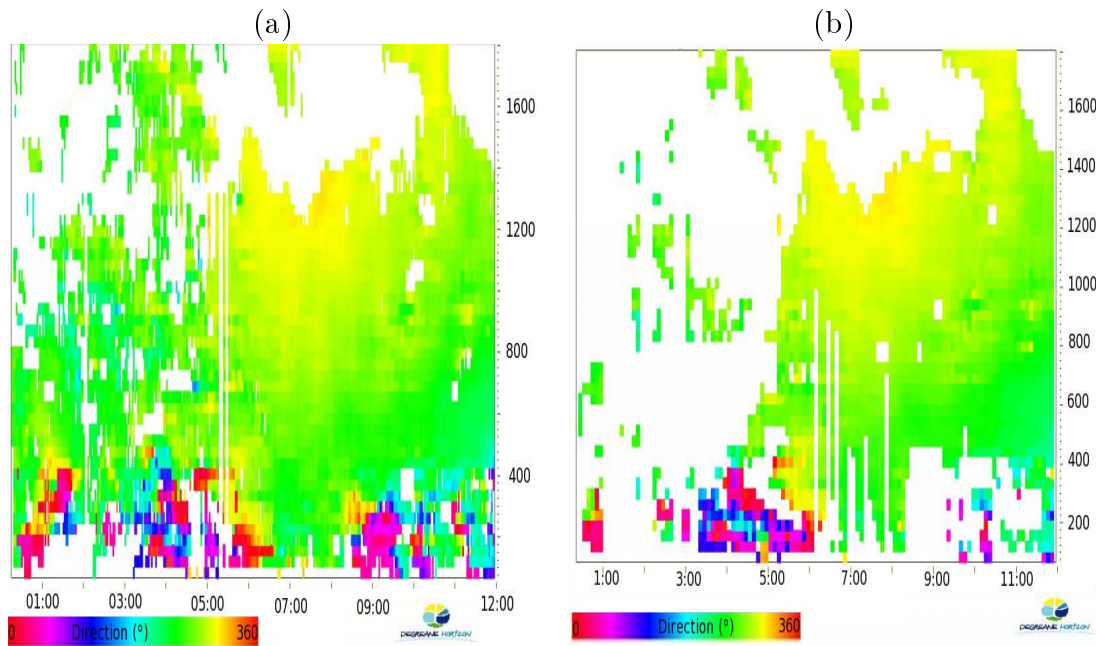
FIGURE 4.8 – Direction du vent observé par le radar profileur de vent PCL-1300 installé sur l'aéroport de Nice entre minuit et midi le 27 Mars 2009. Le graphique (a) est obtenu après traitement des données brutes. Le graphique (b) est le champ stocké dans la banque de données de Météo-France.
