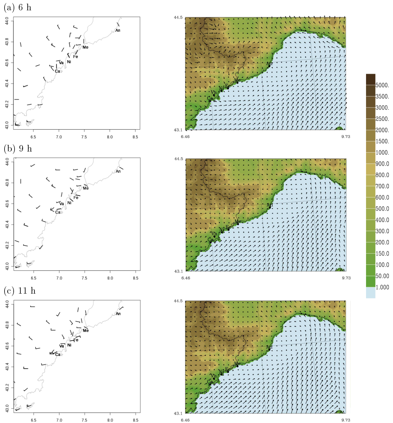
FIGURE 5.22 – Champs de vent à 10 m observés par le réseau de stations de surface le 27 Mars 2009 à 6 h (a), 9 h (b) et 11 h UTC (c), colonne de gauche. Les lettres correspondent aux noms des stations : Cannes (Ca), Valbonne (Va), Nice (Ni), Cap Ferrat (Fe), Menton (Me), Andora (An). La colonne de droite représente le champ de vent simulé par Méso-NH à 2,5 km de résolution (échantillonné une flèche sur trois) au premier niveau du modèle superposé au champ de relief.
