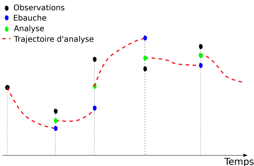
FIGURE 4.12 – Principe des méthodes d'assimilation séquentielles
