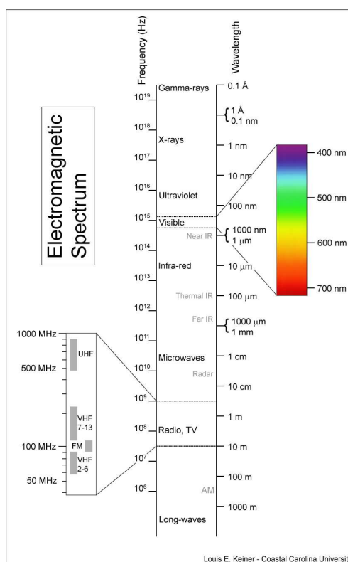
FIGURE 4.1 – Spectre électromagnétique et longueur d’onde associée.
