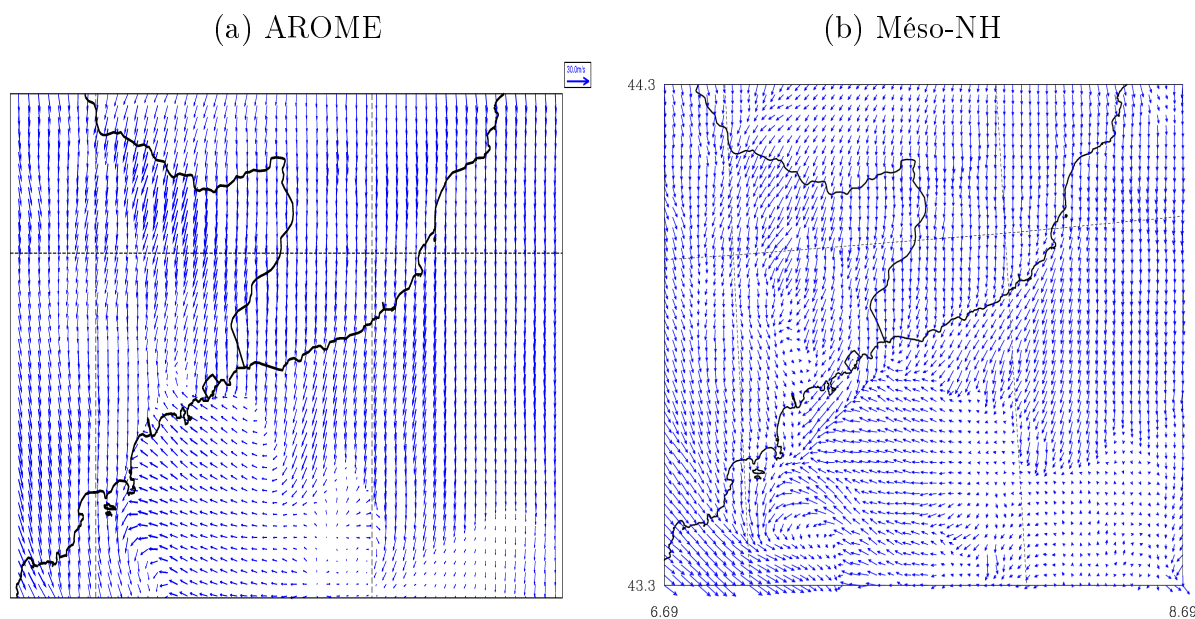
FIGURE 6.6 – Prévision 3 h du réseau de 12 h (à 15 h UTC) du champ de vent au premier niveau du modèle AROME (a) et du modèle Méso-NH (b) le 24 Mars 2009.
