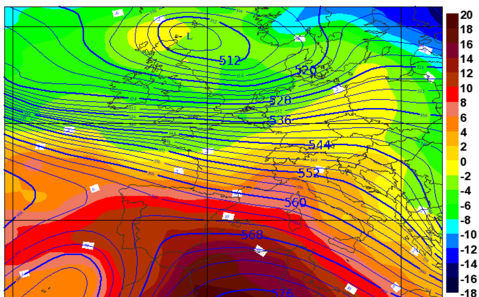
FIGURE 5.16 – Situation synoptique à 6 h du 27 Mars 2009 issue des analyses du CEP-MMT. Les champs colorés correspondent à la température à 850 hPa en °C et les isolignes correspondent au géopotential à 500 hPa en dmgp (décamètres géopotentiels).
