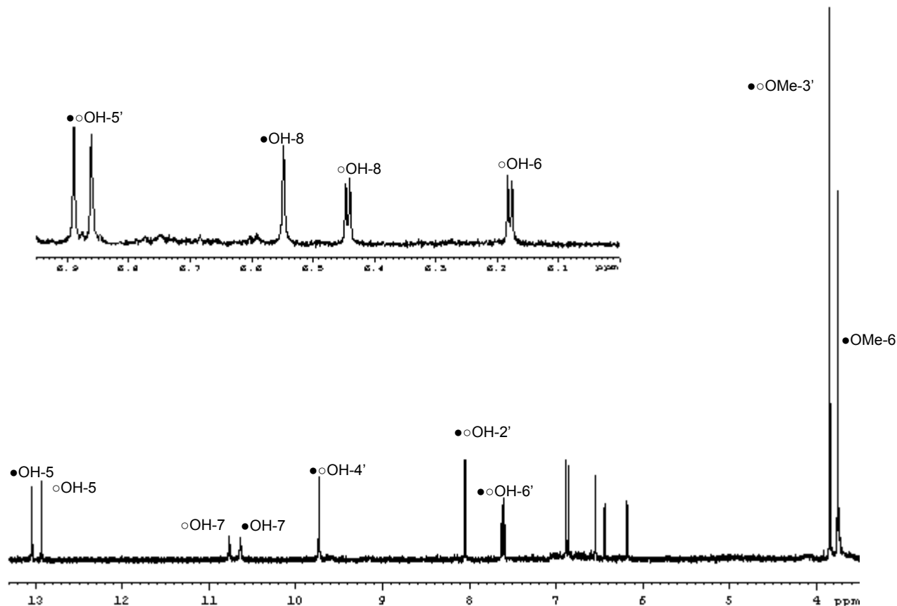
Figure 24 : Spectre de RMN ^1\text{H} du mélange pc2 / pc3 (DMSO, 500 MHz) ; \circ pc2 ; \bullet pc3
