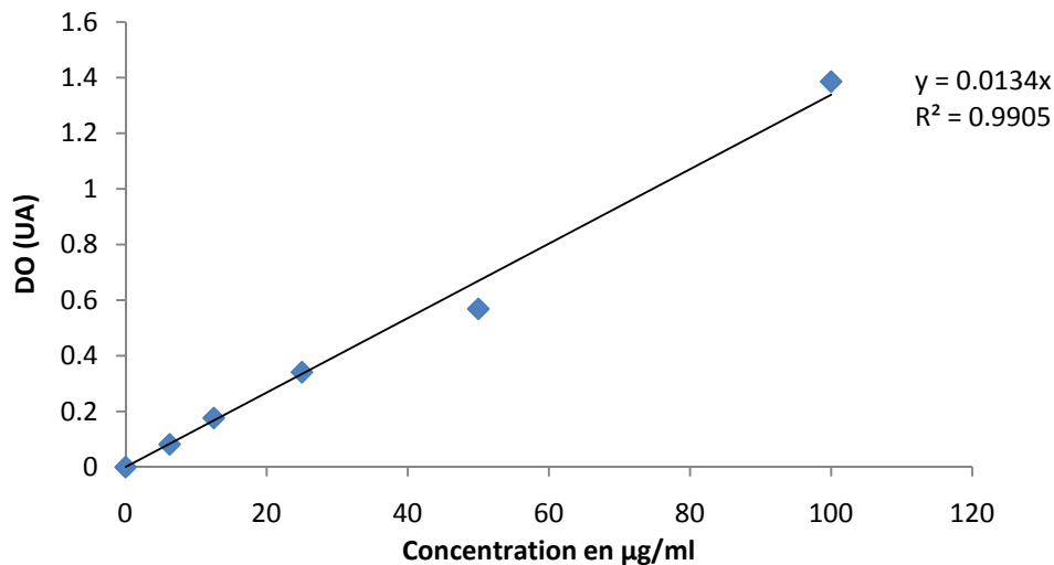
Figure 41 : Gamme étalon des flavonoïdes sulfatés
