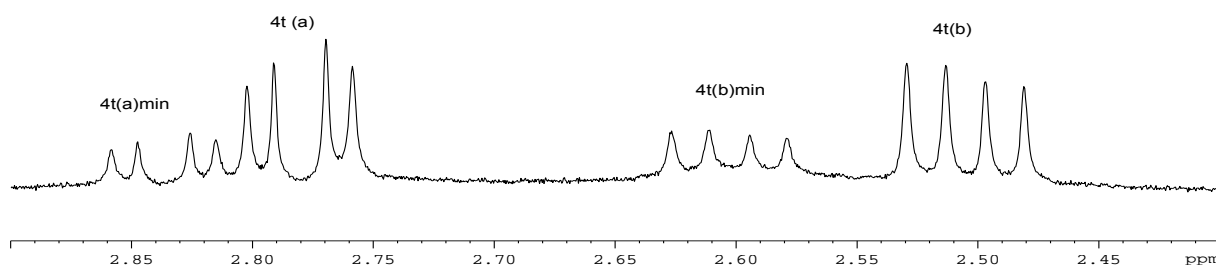
Figure 13 : Agrandissement 1 du spectre de RMN 1 H du composé co2 (CD 3 OD, 500 MHz)
