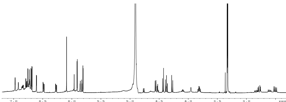
Figure 12 : Spectre de RMN 1 H du composé co2 (CD 3 OD, 500 MHz)
