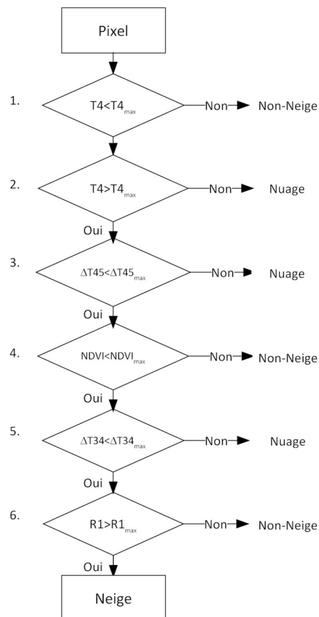
Figure 52 : Schéma d'algorithme de classification des images NOAA-AVHRR.
