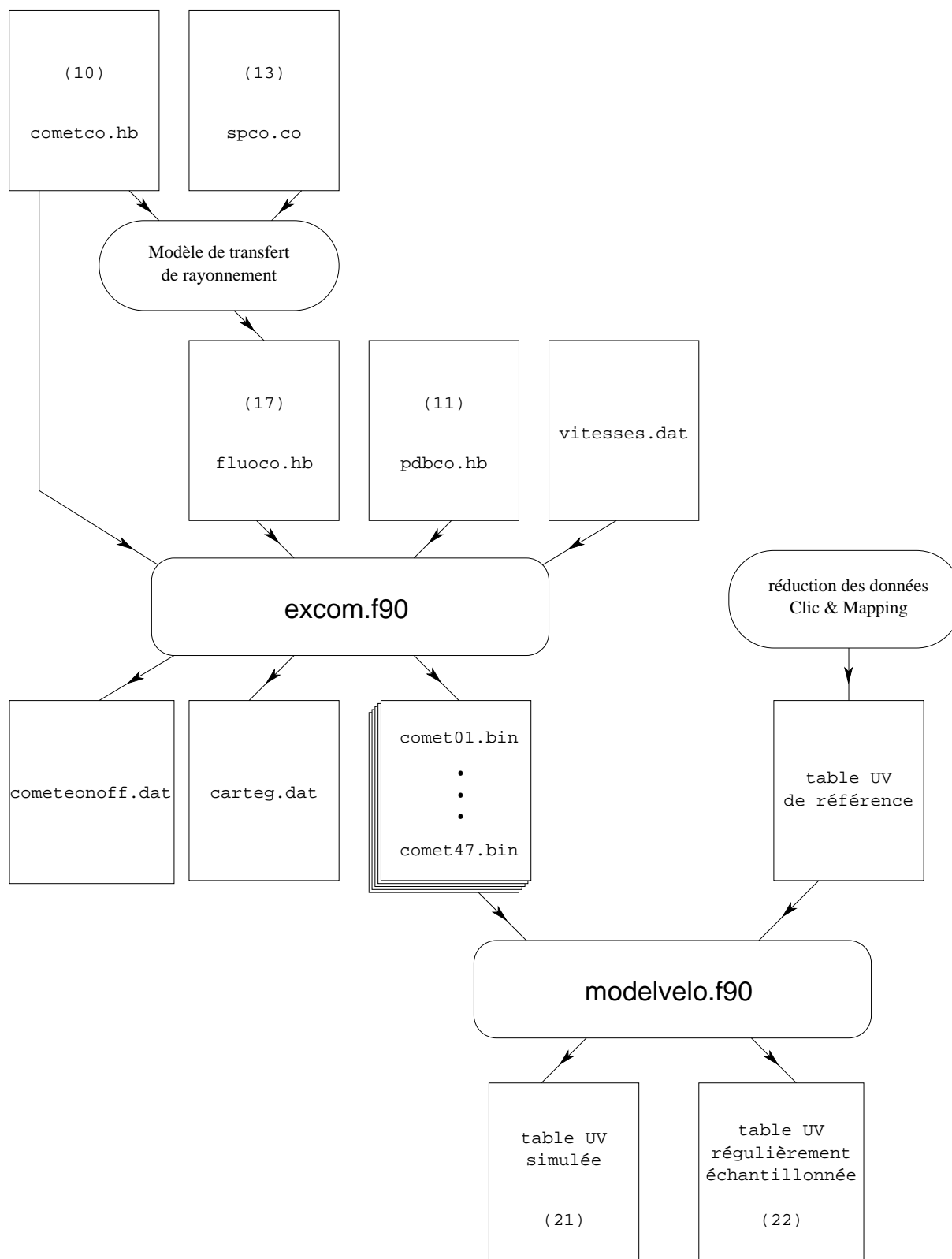
Figure B.1.1 – Schéma des programmes et des fichiers utilisés pour la simulation d'une table uv . Lorsqu'un numéro est donné entre parenthèses, il représente l'unité logique à laquelle il doit être lié.
