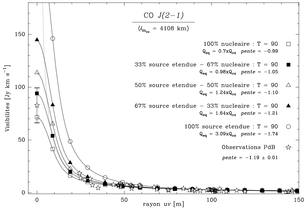
Figure 8.3 – Même légende que pour la figure 8.1, mais avec un parent de CO ayant une longueur d'échelle de \sim 4000 km.
