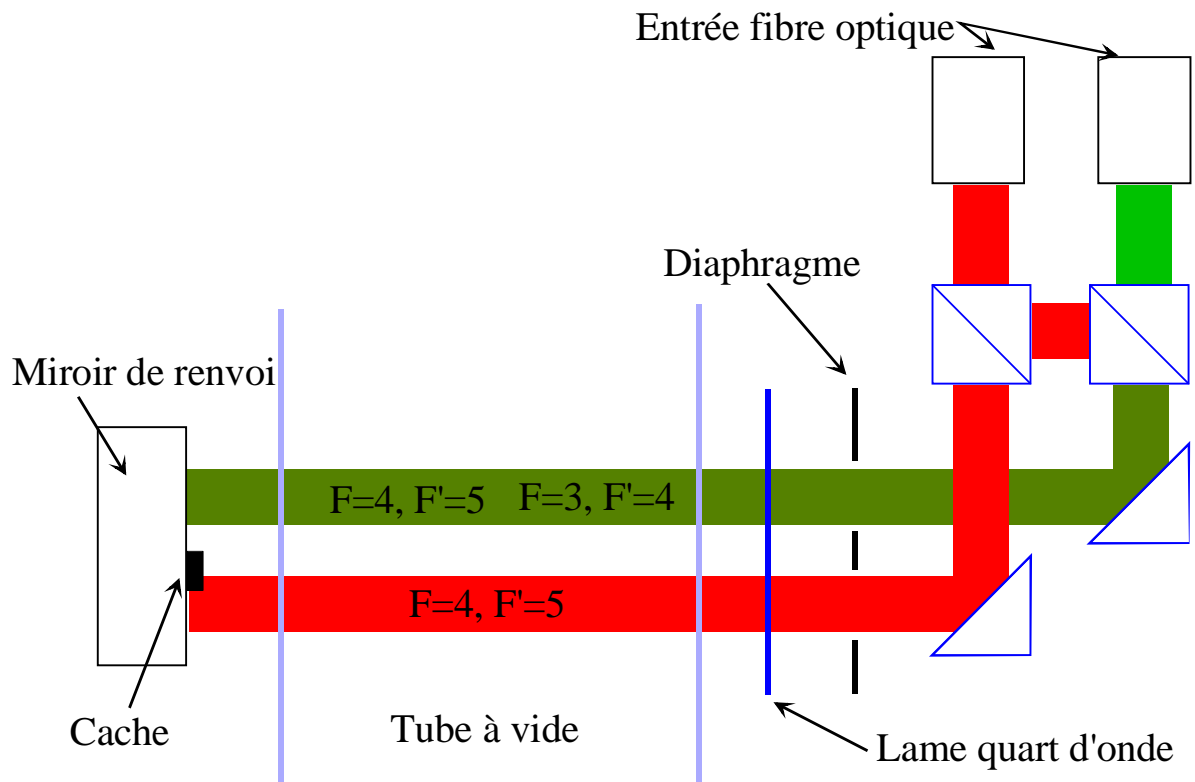
Fig. 6-4: Schéma de principe du système de détection
