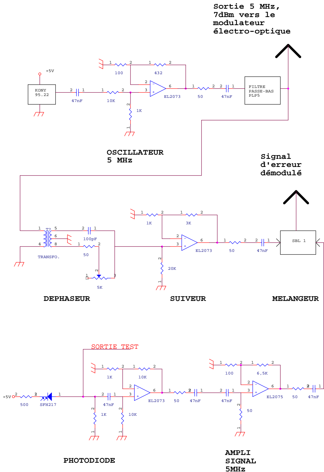
Fig. 8-8 : Schéma du circuit de démodulation du signal d'absorption saturée de la photodiode.
