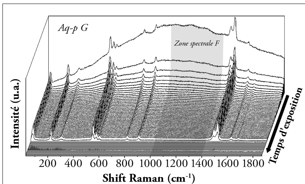
FIG. 3.13 - Évolution du spectre Raman de l'oxalate de cuivre Aq-p G au cours du temps d'exposition à la source laser ( \lambda = 514,5 \text{ nm} , puissance réglée à 3 mW).
