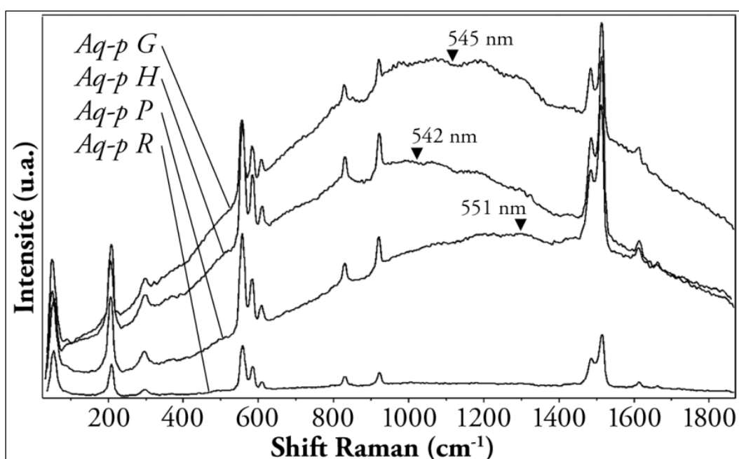
FIG. 3.9 - Spectres de diffusion Raman des poudres d'oxalate de cuivre Aq-p R , Aq-p P , Aq-p H et Aq-p G . Aucun décalage ou changement d'échelle en intensité n'ont été appliqués à ces spectres.
