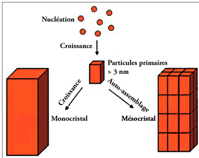
FIG. 1.3 -.Schéma de principe de l'auto-assemblage orienté de NCx comme alternative à la cristallisation par croissance d'un monocristal (d'après Cölfen et al. [21]).
