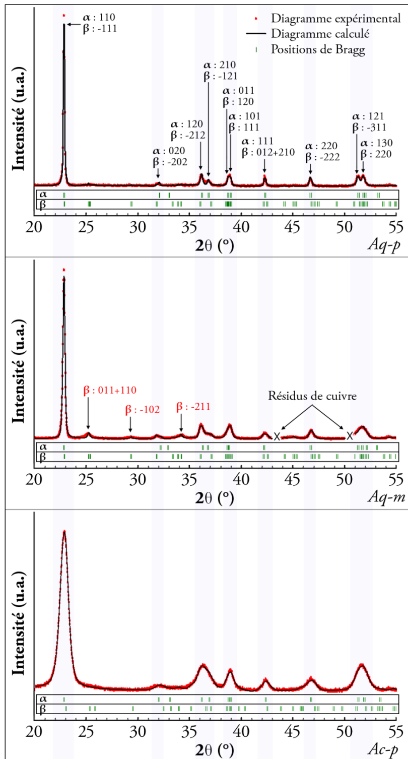
FIG. 2.14 - Diagrammes de DRX expérimentaux et résultats des affinements obtenus pour le \text{CuC}_2\text{O}_4 Aq-p (en haut), Aq-m (au milieu) et Ac-p (en bas).
