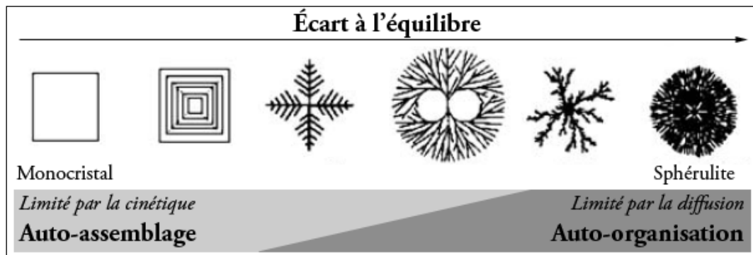
FIG. 1.1 - Représentation schématique de structures issues de processus d'auto-assemblage et d'auto-organisation (d'après Imai [2]).
