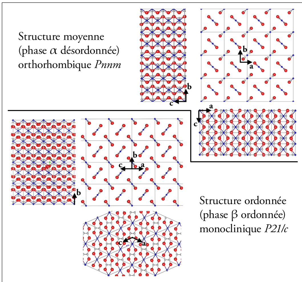
FIG. 2.16 - Représentation schématique des structures désordonnée et ordonnée de CuC_2O_4 affinées par la méthode de Rietveld à partir des diagrammes de DRX puis des diagrammes de DN.
