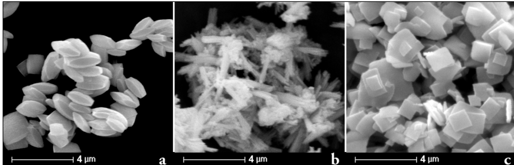
FIG. 2.4 - Images MEB de particules de \text{CuC}_2\text{O}_4 Aq-p (a), Ac-p (b) et Aq-m (c).
