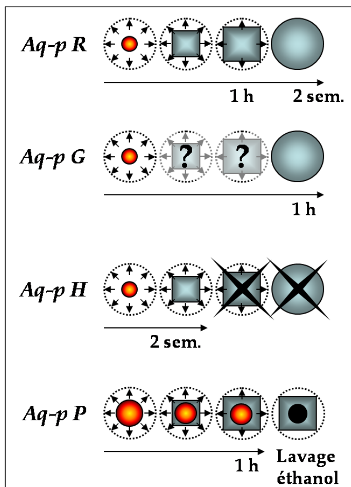
FIG. 3.4 – Schéma résumant les effets cinétiques du glycérol, de l'HPMC et du PEG sur les étapes du mécanisme d'auto-assemblage menant aux mésocristaux respectivement Aq-p G , Aq-p H et Aq-p P . La zone du mésocristal représentée en jaune et rouge correspond au cœur constitué de nanocristaux désordonnés. La zone représentée en vert est celle constituée de nanocristaux ordonnés de manière orientée.
