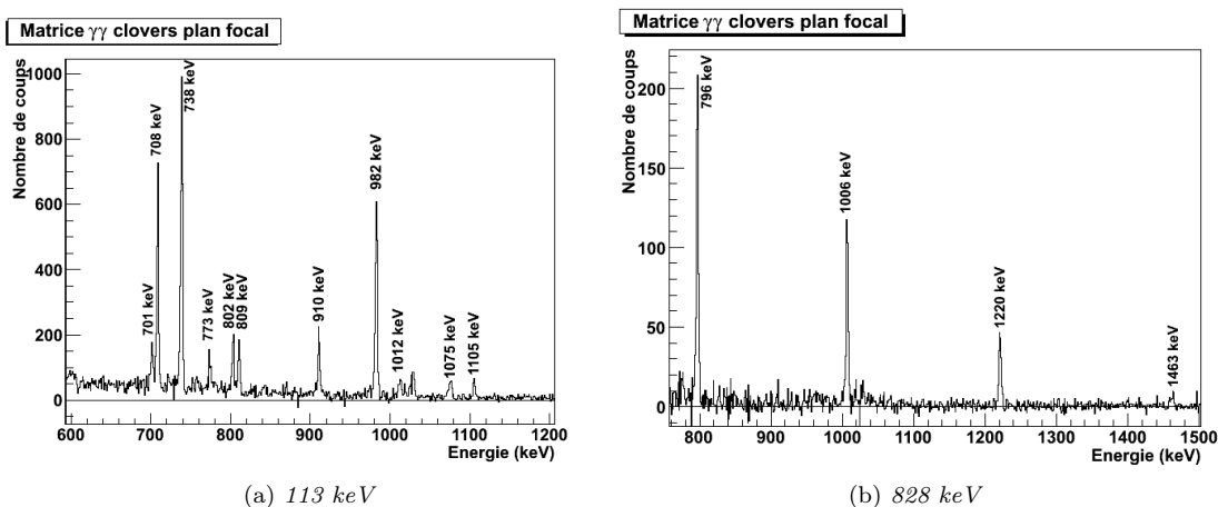
FIGURE IV.6 – Spectres conditionnés par les transitions à (a) 113 keV ou (b) 828 keV qui alimentent le niveau fondamental du ^{139}\text{Pr} observé par décroissance \beta du ^{139}\text{Nd} au plan focal.
