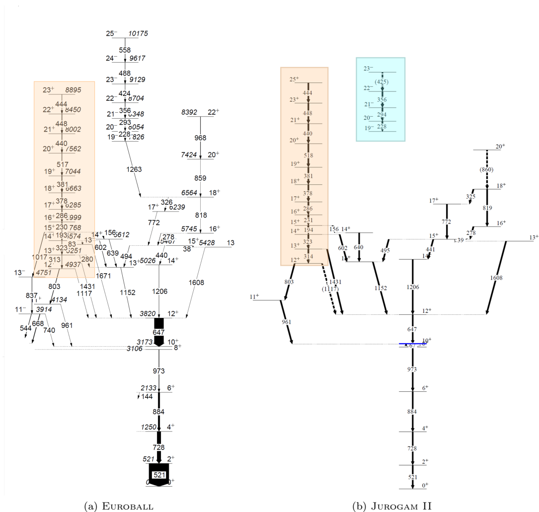
FIGURE IV.19 – Schémas de niveaux partiels du noyau ^{138}\text{Nd} montrant l'alimentation de l'état isomérique du niveau 10^+ . Ils ont été établis (a) par l'expérience Euroball et (b) par notre étude. Les zones encadrées représentent respectivement la bande principalement étudiée dans le texte (orange), et la bande flottante observée dans notre étude (en vert sur la figure (b)). Le niveau isomérique est noté en bleu.
