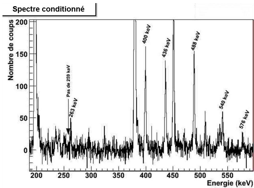
FIGURE V.13 – Spectres conditionnés des transitions intrabandes des bandes \gamma de spins (a) pairs et (b) impairs obtenus en imposant des coïncidences sur les interbandes vers la bande fondamentale.
