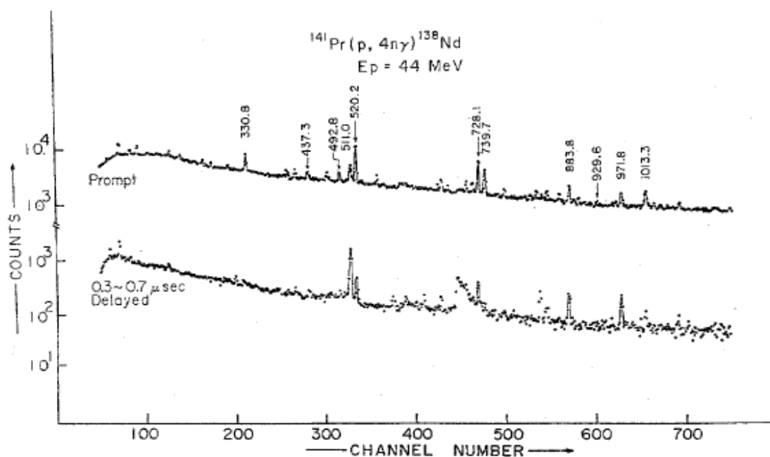
FIGURE III.5 – Spectre \gamma prompt et retardé du ^{138}\text{Nd} montrant l'existence d'un état isomérique au dessus du niveau à 3130 keV [Yos75].
