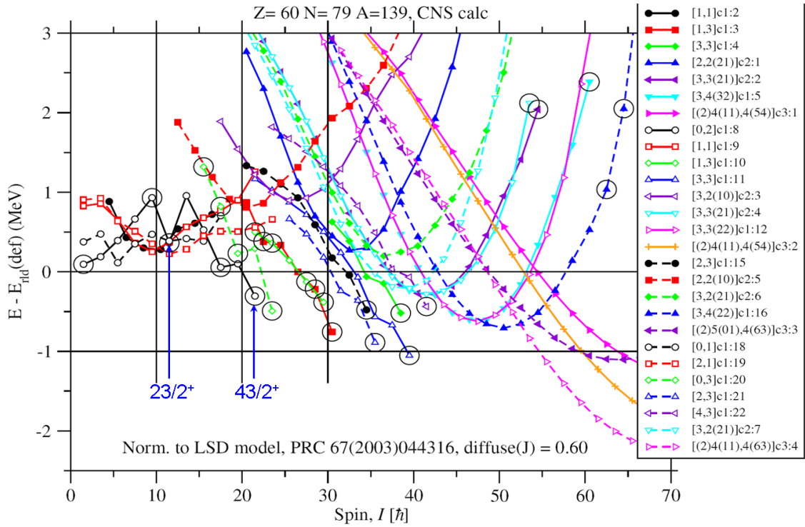
FIGURE II.4 – Etats de configurations calculés par modèle CNS du ^{139}\text{Nd} [Rag]. Les flèches bleues repèrent deux états favorisés de spin 23/2^+ et 43/2^+ qui sont des candidats pour des états isomériques.
