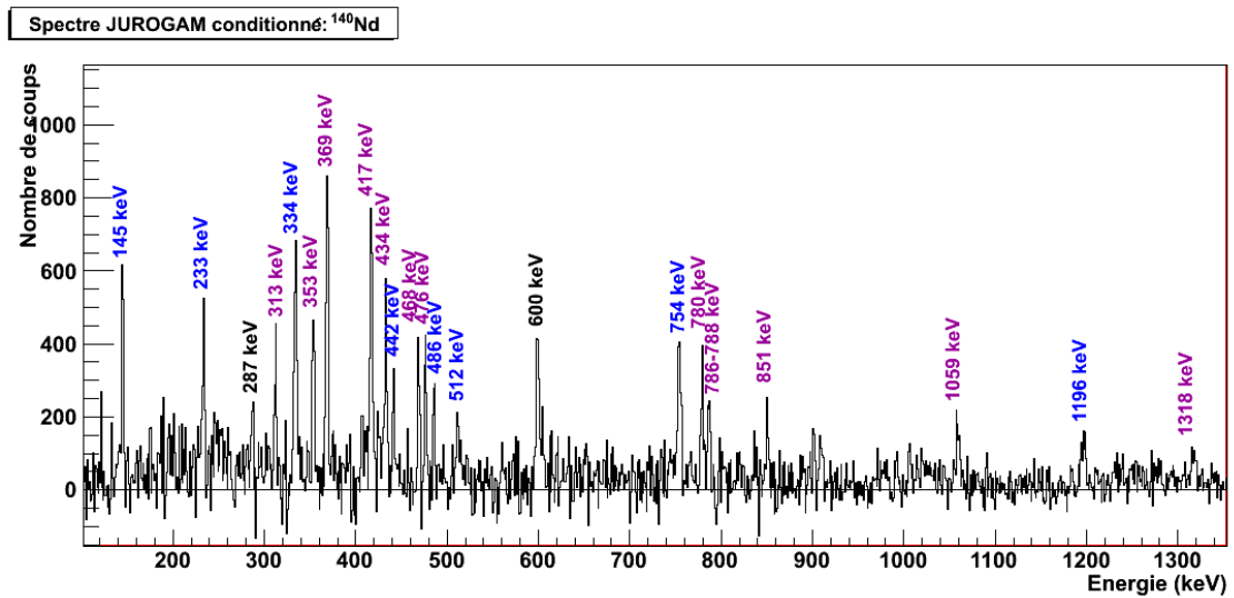
FIGURE IV.16 – Spectre conditionné par les transitions de la bande flottante au dessus du spin 26.
