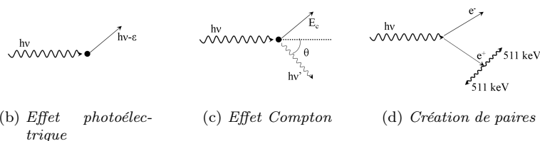
FIGURE III.8 – Sections efficaces des interactions photon-matière pour le germanium en fonction de l'énergie du photon incident (a) et schéma des trois interactions majeures d'un photon avec la matière : (b) effet photoélectrique, (c) effet Compton, et (d) création de paires électron-positron.
