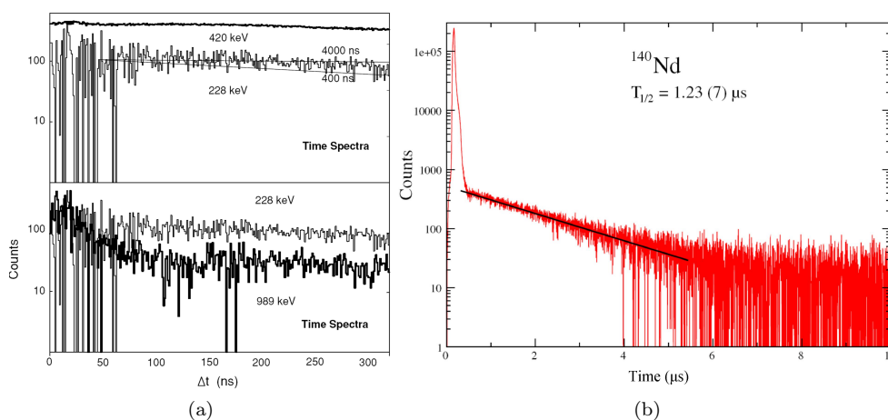
FIGURE III.1 – Spectres en temps des transitions en dessous de l'isomère 20^+ à 7393 keV du ^{140}\text{Nd} obtenus dans les études de (a) Petrache et al. [Pet06] en 2006 et (b) Ferraton et al. [Fer08] en 2008.
