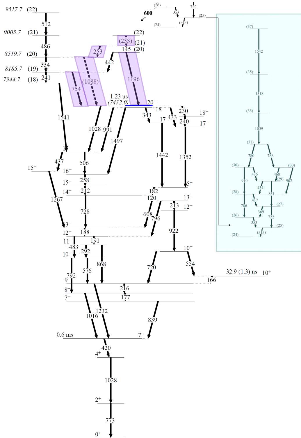
FIGURE IV.9 – Schéma de niveaux partiel du ^{140}\text{Nd} montrant les nouvelles transitions d'alimentation du niveau isomérique 20^+ (repéré en bleu sur le schéma). Les transitions mises en évidence dans cette étude sont encadrées et la bande flottante encadrée en vert est discutée section IV.3.
