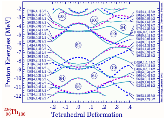
FIGURE V.3 – Niveaux d'énergie individuelles pour les protons en fonction de la déformation tétraédrique [Dud03].
