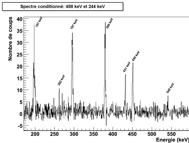
FIGURE V.18 – Spectres conditionnés par la transition à 488 keV ( 13_{\gamma}^{+} \rightarrow 11_{\gamma}^{+} ) et par (a) 341 keV ou (b) 244 keV. Sur le spectre (a) nous apercevons la transition à 244 keV et le spectre (b) permet de confirmer son placement dans le schéma.
