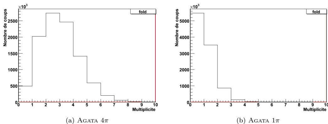
FIGURE VI.11 – Multiplicité des événements détectés par le multidétecteur de rayonnement \gamma (a) AGATA 4\pi et (b) AGATA 1\pi . La multiplicité est déterminée ici pour 10 millions de cascades générées dans le détecteur.
