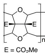
Schéma 113 : Analogie structural cyclique des CB
