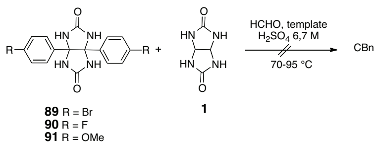
Schéma 80 : Adaptation de la voie de synthèse du CB6Ph2 aux diphenylglycolurils fonctionnalisés
