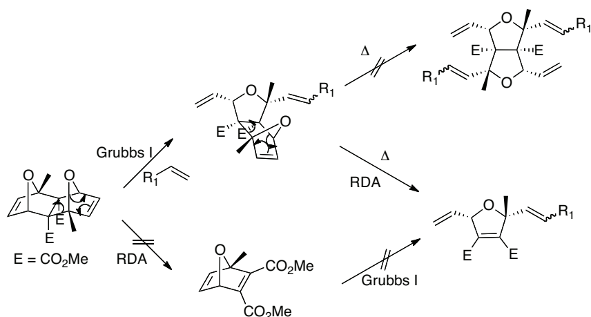
Schéma 138 : Mécanismes éventuels de la réaction de rétro Diels-Alder
