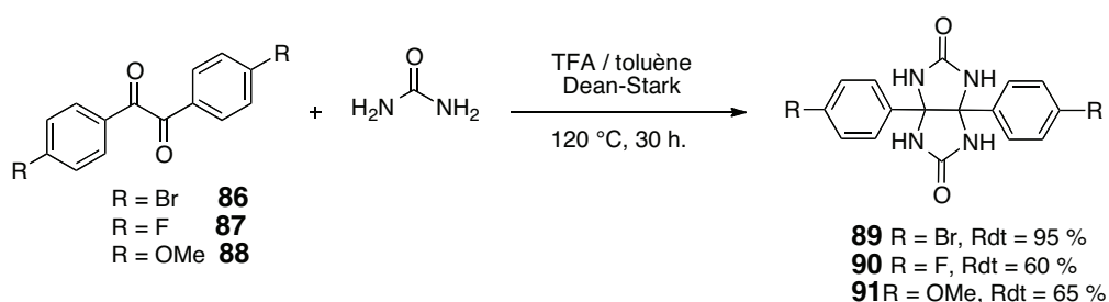
Schéma 79 : Synthèse des diphenylglycolurils fonctionnalisés
