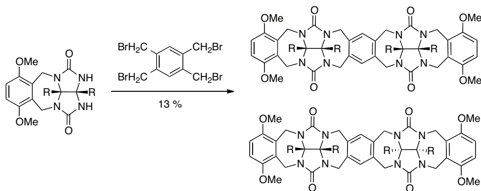
Schéma 116 : Analogues linéaires du cucurbituril
