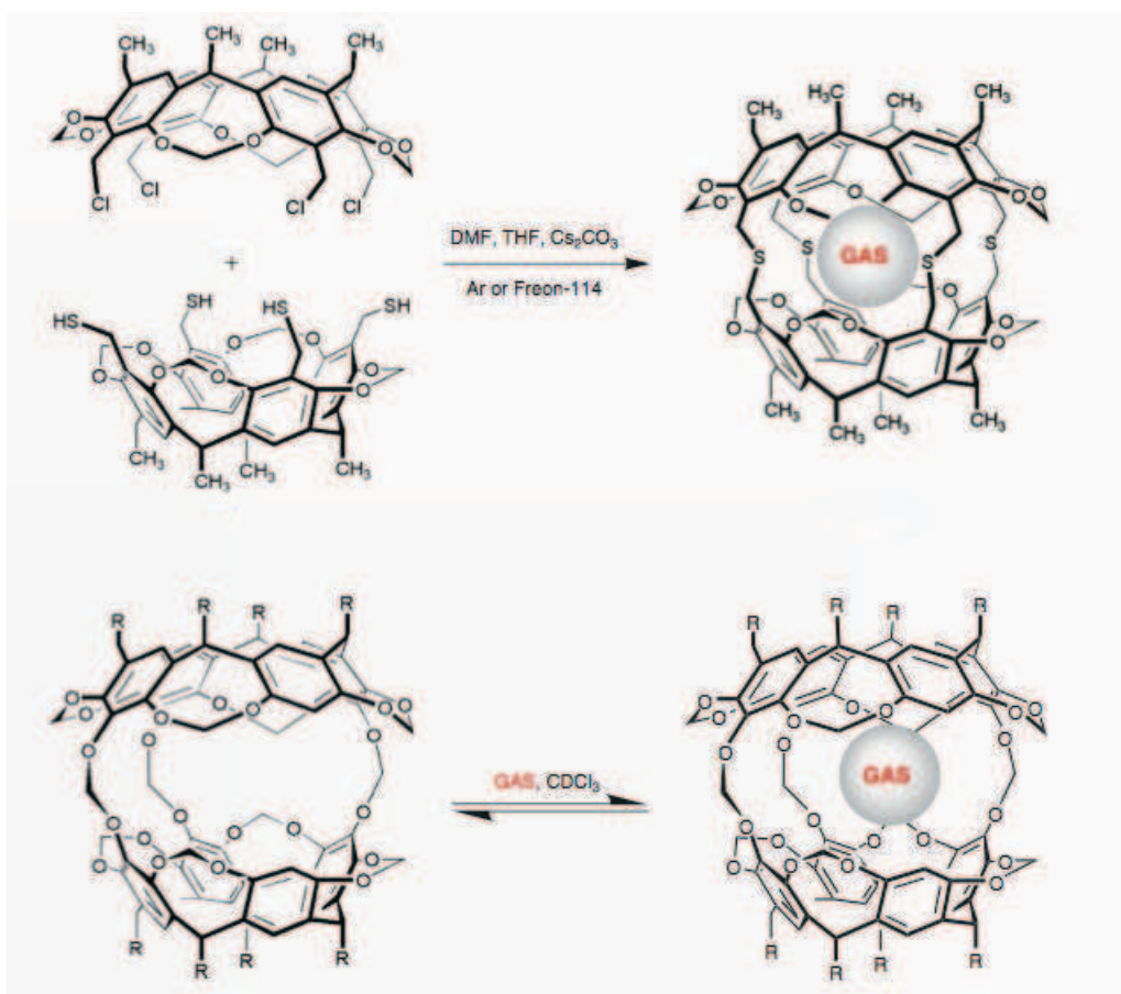
Schéma 5 : Carcérand (en haut) et hémicarcérand (en bas) en présence de gaz
