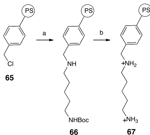
Schéma 59 : Préparation de la résine 67
