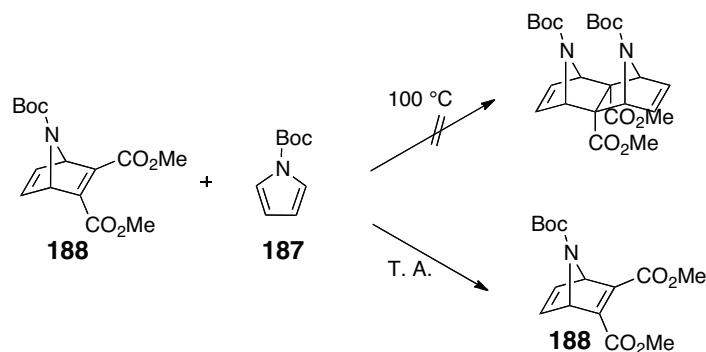
Schéma 147 : Essais de synthèse du tétracycle azoté à partir du bicyclic 188
