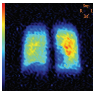
Schéma 10 : IRM des poumons après inhalation d'hélium-3 hyperpolarisé (en bleu : hélium)
