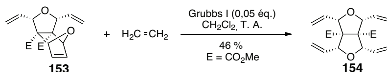
Schéma 128 : Réaction du produit mono-ouvert 153 en présence d'éthylène
