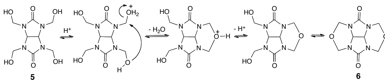
Schéma 22 : Équilibre tétra-alcool diéther (R = H)
