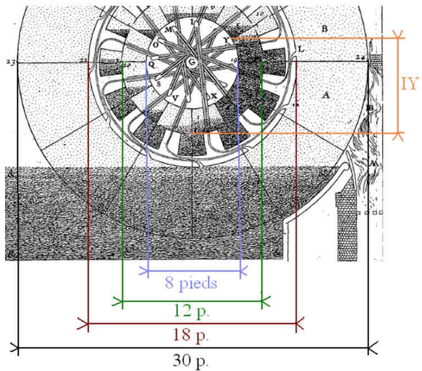
Figure 18 : Cotes du moulin à feu d'Amontons. La profondeur des cellules est de 2 pieds, et la longueur IY représente la hauteur d'eau.
