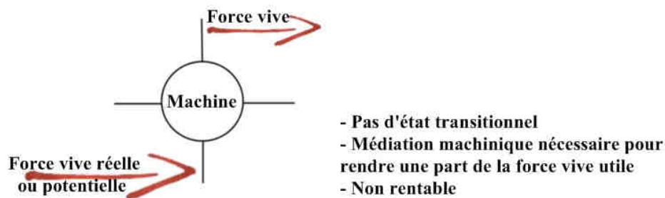
Figure 50 : La conversion du travail en force vive a lieu dans tous les cas. Il n'en va pas ainsi pour la conversion réciproque, qui n'a lieu que de manière intra organique, et qui n'est qu'une modélisation, la force vive originelle restant inquantifiable.
