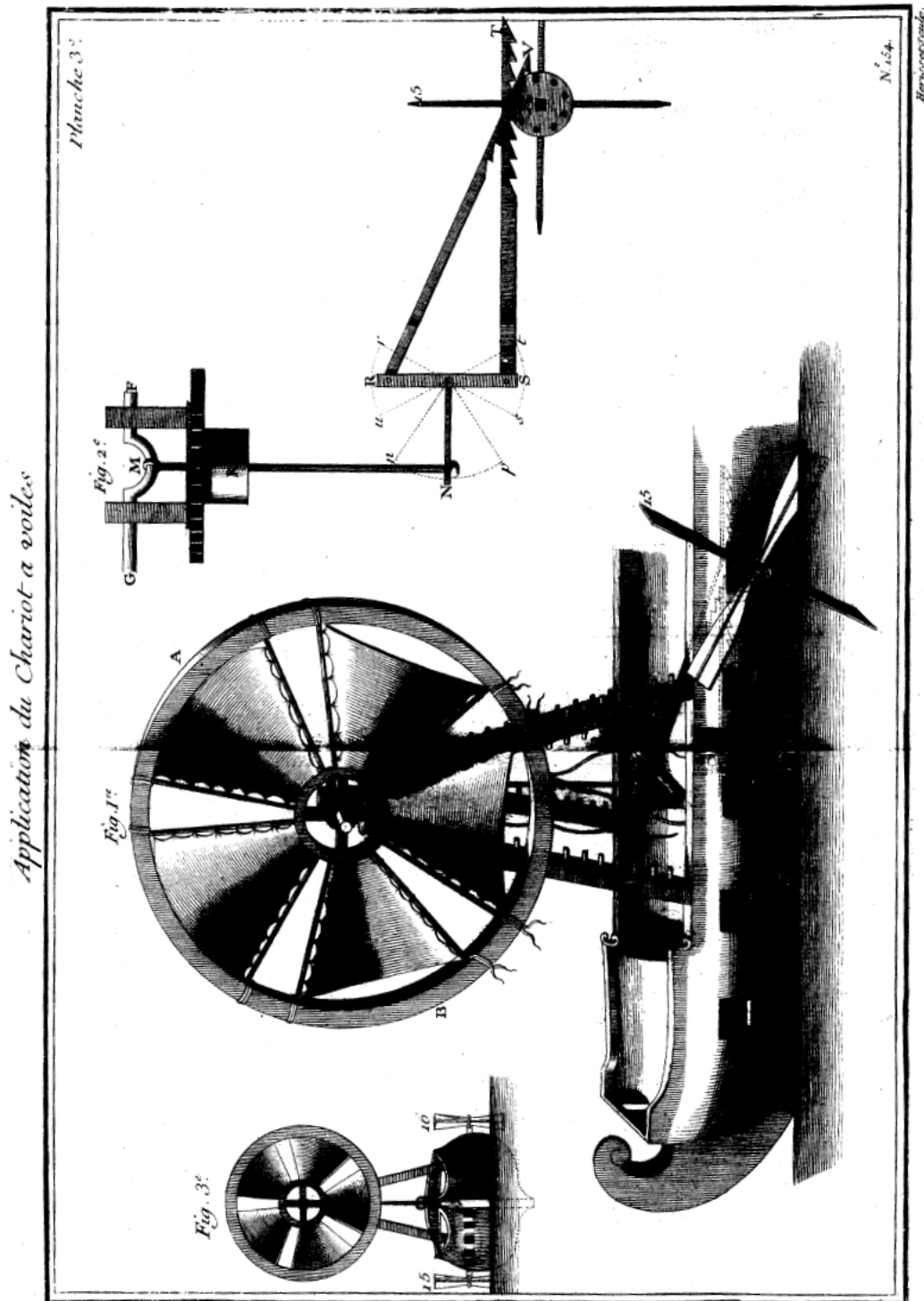
Figure 72 : Application de la mécanique du chariot à voile de Du Quesne à un vaisseau, approuvé en 1714 à l'Académie (figure tiré du tome III des Machines, p. 42)
