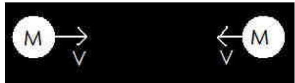
Figure 42 : Deux corps de même masse, et de même vitesse arrivant l'un sur l'autre.
